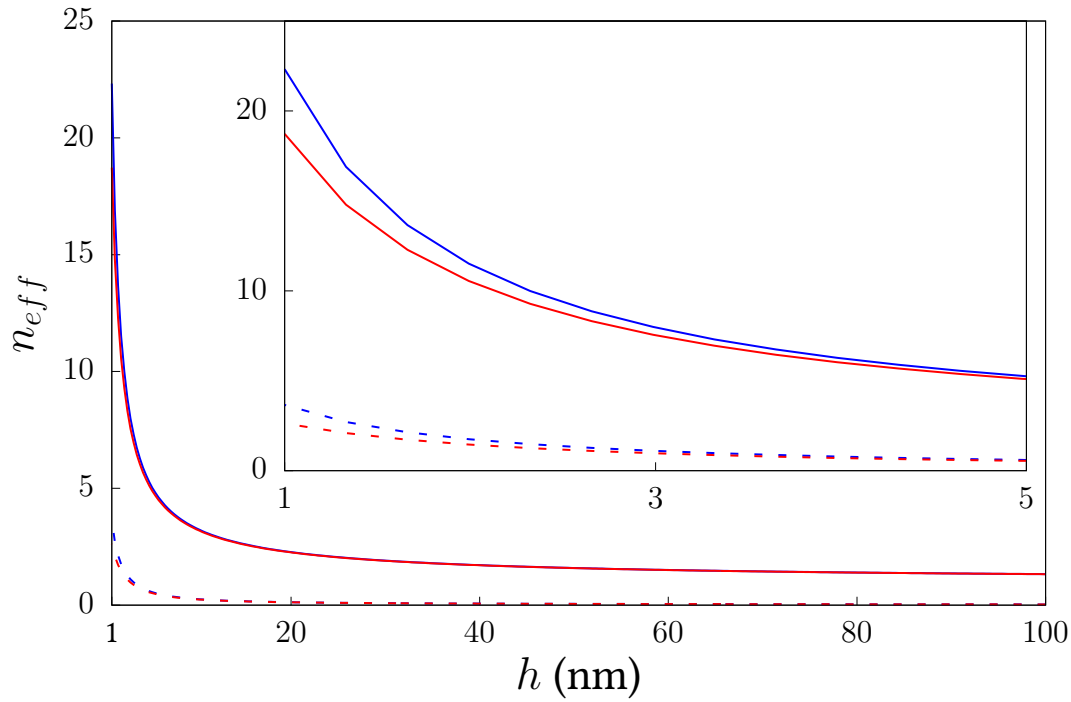
FIGURE 2.11 – Courbe de dispersion du gap-plasmon en fonction de l'épaisseur du gap h pour un M.I.M. fait d'Air et d'Or et \lambda_0 = 600 nm. Les courbes bleues sont obtenues en considérant un métal local et les rouges un métal non local. Les courbes pleines sont des \Re(n_{eff}) et les pointillées des \Im(n_{eff}) . L'inset montre un zoom aux très faibles épaisseurs.
