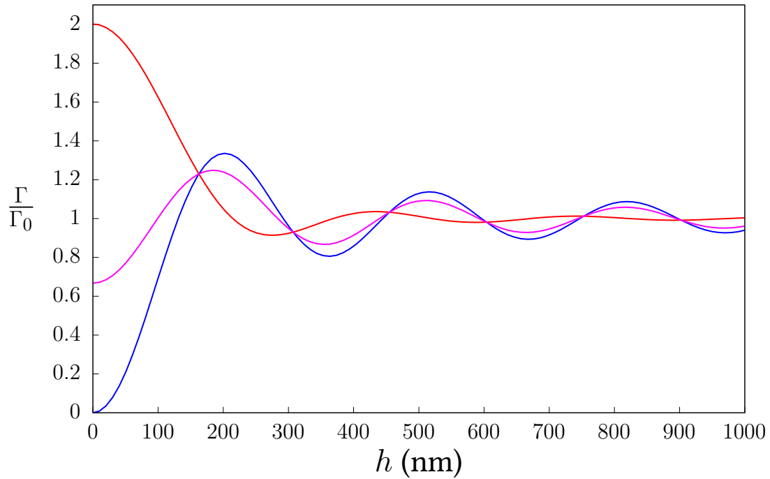
FIGURE 4.14 – Taux d’émission normalisé pour un dipôle au dessus d’un plan métallique parfait pour différentes orientations du dipôle. La courbe rouge correspond à un dipôle perpendiculaire à l’interface, la bleu à un dipôle parallèle à l’interface et la magenta à une orientation isotropique.
