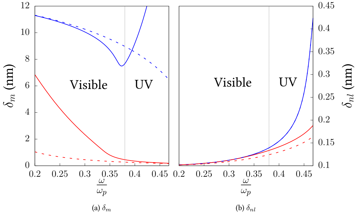
FIGURE 2.24 – Distances de pénétration dans le métal de l’onde transverse \delta_m (a) et de l’onde longitudinale \delta_{nl} (b) en fonction de la fréquence normalisée pour un I.M.I. symétrique de \text{TiO}_2 et d’argent d’épaisseur h = 10 nm (courbes pleines) et h = 1 nm (courbes pointillées). Les courbes rouges correspondent au SRSP et les bleues au LRSP. Chacune est obtenues en considérant un métal non local. Pour le LRSP \delta_{nl} est identique quel que soit l’épaisseur alors que \delta_m varie à cause de l’augmentation de la fréquence de bend back avec la diminution en épaisseur.
