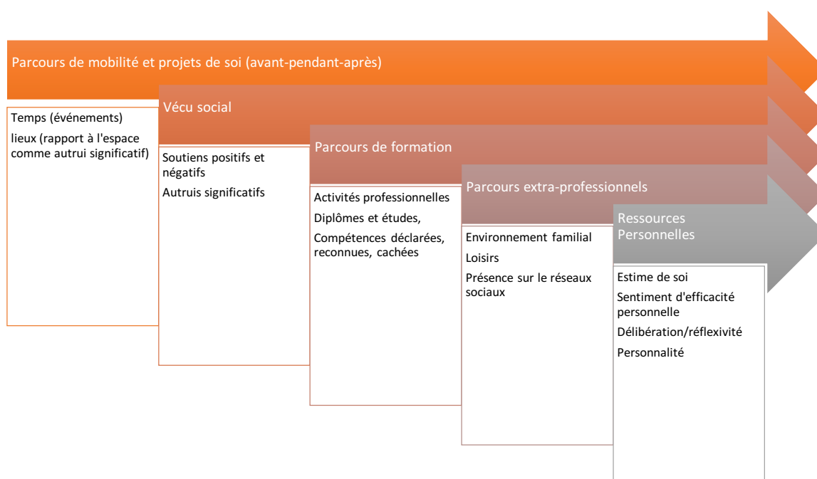
Figure 4 : Les dynamiques emboîtées à l'œuvre durant la transition et dans la situation mobilité.
