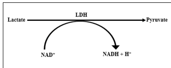
Figure 15: Principe de dosage de la LDH
