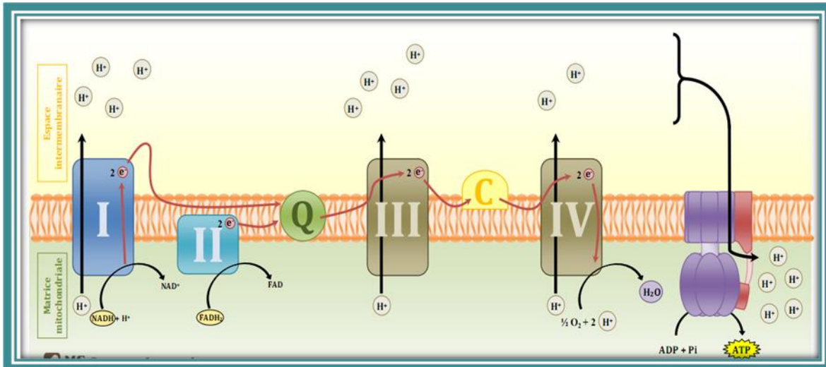
Figure 6 : Schéma représentatif de chaîne de transport des électrons et des sites de production des ERO au niveau de la membrane interne mitochondriale
