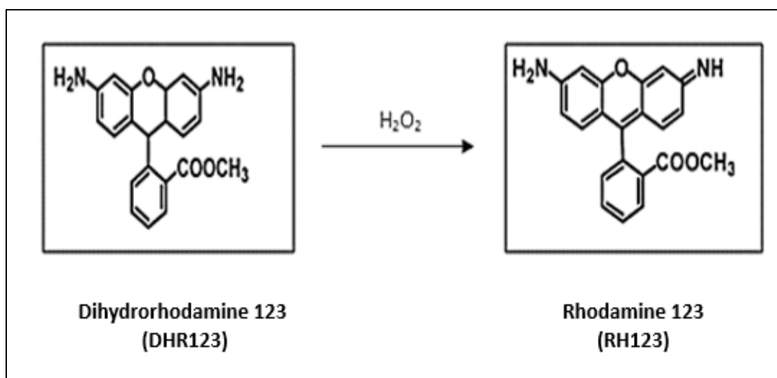
Figure 13: Schéma d'oxydation de DHR123 en RH123 en présence de H_2O_2 (Richardson et al., 1998)
