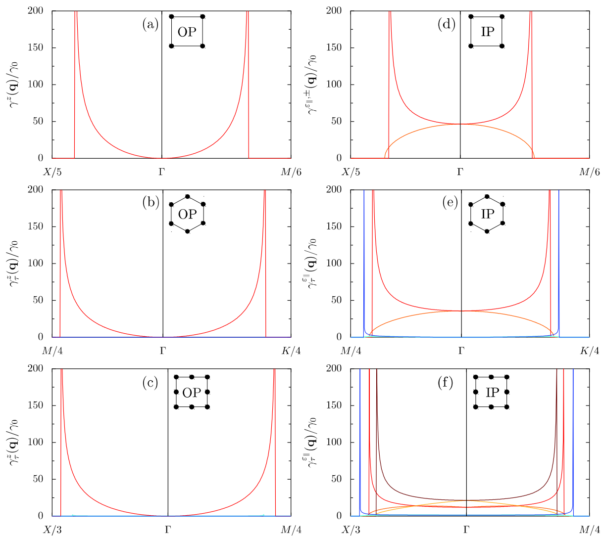
Figure 8: Les lignes de couleurs montrent le taux de décroissance radiatif \gamma_{\tau}^{\epsilon}(\mathbf{q}) écrit à l'Eq. (15) (divisé par \gamma_0 , cf. Eq. (2)) pour les réseaux (a),(d) carré, (b),(e) en nid d'abeilles et (c),(f) Lieb. Les panneaux (a)–(c) [(d)–(f)] montrent les modes polarisés hors du [dans le] plan. Mêmes paramètres que pour la Fig. 7.
