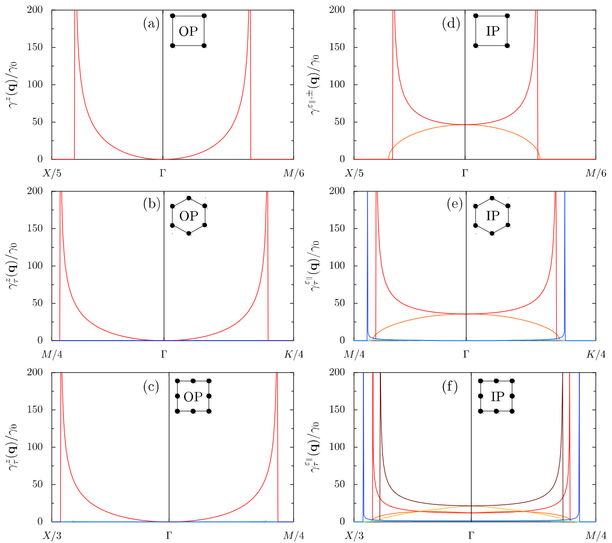
Figure 8: Les lignes de couleurs montrent le taux de décroissance radiatif \gamma_\tau^\varepsilon(\mathbf{q}) écrit à l'Eq. (15) (divisé par \gamma_0 , cf. Eq. (2)) pour les réseaux (a),(d) carré, (b),(e) en nid d'abeilles et (c),(f) Lieb. Les panneaux (a)–(c) [(d)–(f)] montrent les modes polarisés hors du [dans le] plan. Mêmes paramètres que pour la Fig. 7.
