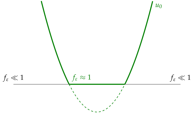
FIGURE 1.3 : Illustration du comportement de la solution de l'équation de Hamilton-Jacobi (1.1.10).
