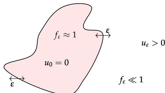
FIGURE I.2 : Lien entre le comportement de u_\varepsilon et f_\varepsilon quand \varepsilon est petit.
