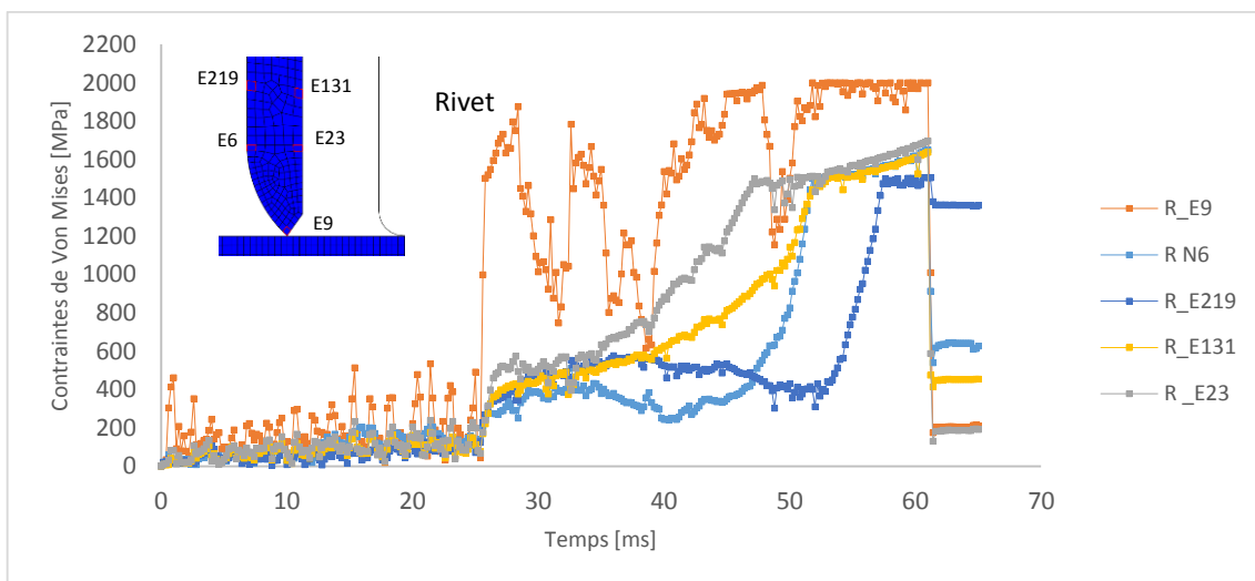
Figure 3-17: Évolution des contraintes de Von Mises à différentes positions du modèle pour le rivet
