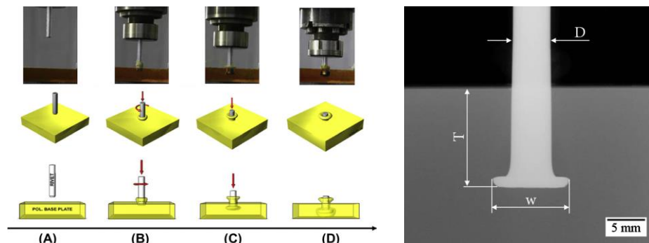
Figure 1-24: Principe du procédé FricRiveting [78] et vue en coupe d'un joint riveté par rayon X [76]
