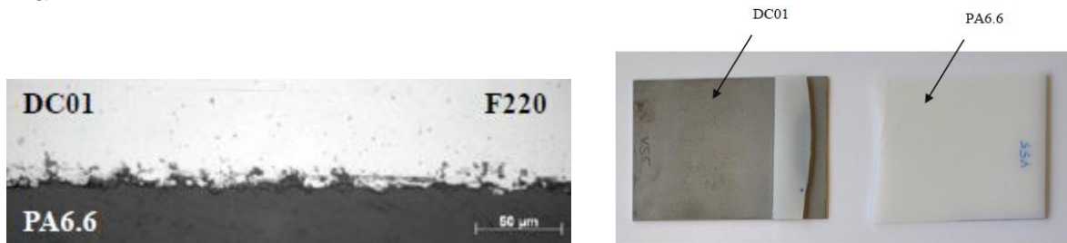
Figure 1-21: Vue en coupe à l'interface d'un joint soudé acier DC01 / PA6.6 et profil de rupture [62]
