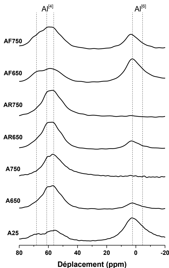
Figure 1. Spectres RMN MAS de l' Al^{27} des différents types d'argilites crue et calcinées.
