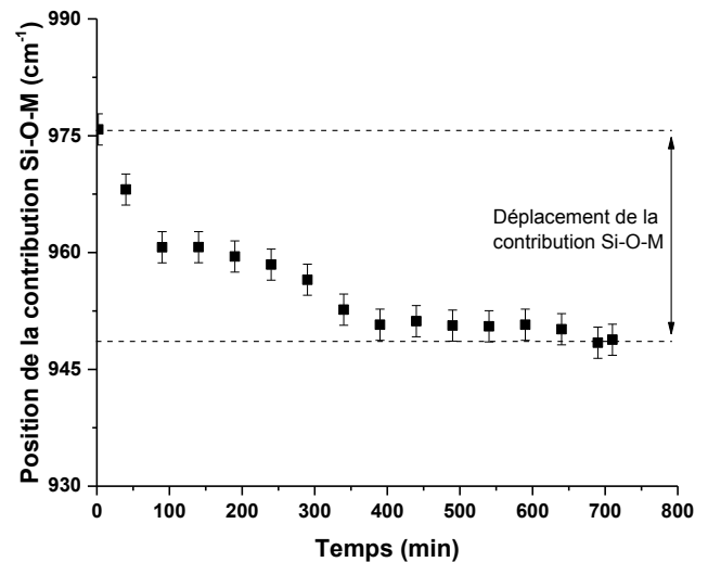
Figure 5. Données IRTF de (A) l'argilite crue A25 et (B) du suivi cinétique de la consolidation du mélange réactif S1 1,17 A750 0,58 (a) spectres et (b) récapitulatif de l'évolution de la position de la contribution Si-O-M au cours du temps.
