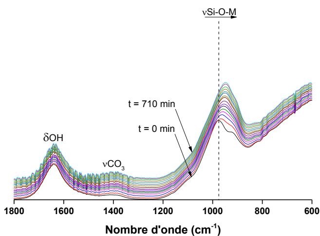
Figure 5. Données IRTF de (A) l'argilite crue A25 et (B) du suivi cinétique de la consolidation du mélange réactif S1 1,17 A750 0,58 (a) spectres et (b) récapitulatif de l'évolution de la position de la contribution Si-O-M au cours du temps.
