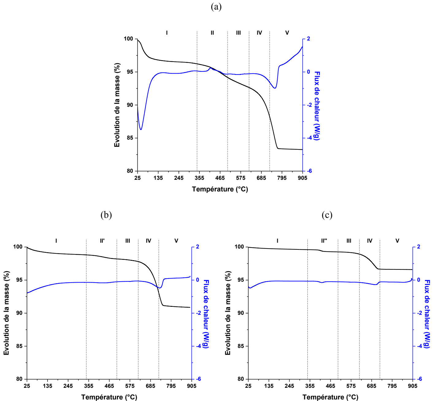
Figure 1. Thermogrammes de (a) l'argilite crue (A25) et des argilites calcinées en four statique à (b) 650 et (c) 750 °C.
