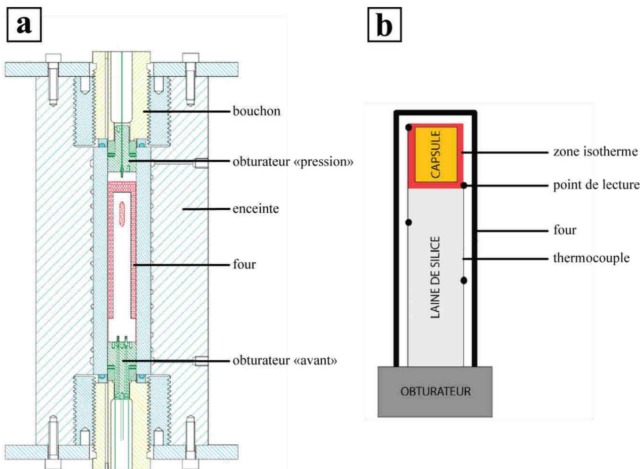
Figure V-1: (a) coupe longitudinale d'un autoclave à chauffage interne schématisant la disposition du four, des obturateurs et des bouchons associés [ Champallier , 2005]. (b) Vue conceptuelle de l'agencement entre thermocouples et capsule au sein d'un four, d'après Picard [2009].
