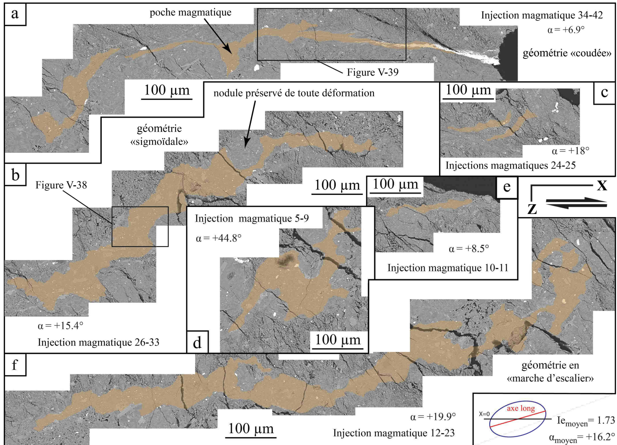
Figure V-37: clichés MEB pris dans la zone de cisaillement au sein de la section [xz] du produit expérimental #4 déformé en torsion (expérience PP565 ; cf. Figure V-31), répertoriant l'ensemble des injections magmatiques (a-f) observées. Ces injections magmatiques sont coloriées en beige sur les clichés. En bas à droite : ellipse tensorielle moyenne des injections magmatiques, avec \alpha_{moyen} la direction d'allongement moyenne de l'ellipse et I_{e_{moyen}} la force de fabrication moyenne.
