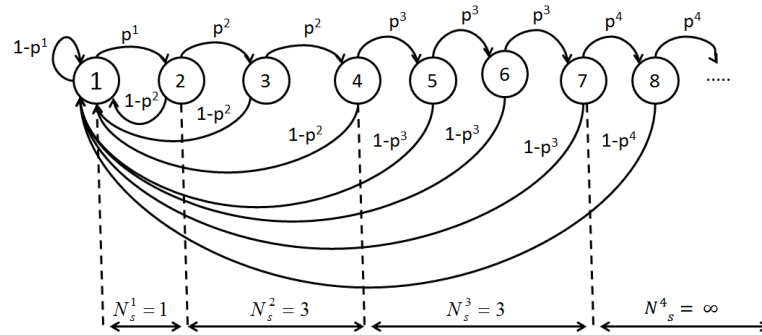
Figure 8.14: La chaîne de Markov modélisant la phase de contention après une période occupée.
