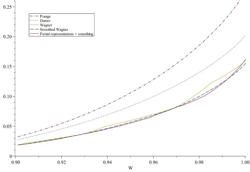
Figure 3.6 – Comparaisons des différents exposants asymptotiques des algorithmes pour résoudre le problème du décodage ternaire en fonction de \omega \triangleq w/n pour R = 1/2 .
