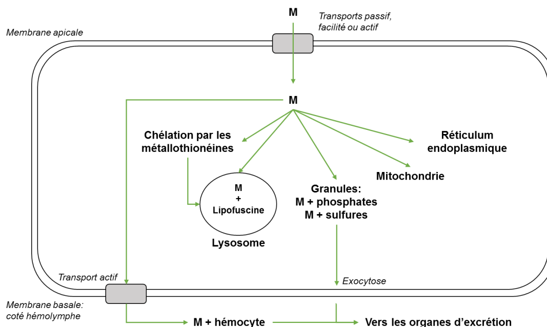
Figure I-B. 10 Principaux devenir des éléments métalliques dans les cellules. Une fois la membrane plasmique franchie, les métaux peuvent être excrétés rapidement dans l'hémolymphe, chélatés par des protéines ayant une forte affinité pour ces éléments (comme les métallothionéines), transportés dans divers organites (lysosome, mitochondrie ou réticulum endoplasmique) où ils seront stockés sous formes détoxiquées ou être complexés à d'autres molécules (sulfures, phosphates) sous forme de granules qui seront exocytés. D'après Ahearn et al. (2004).
