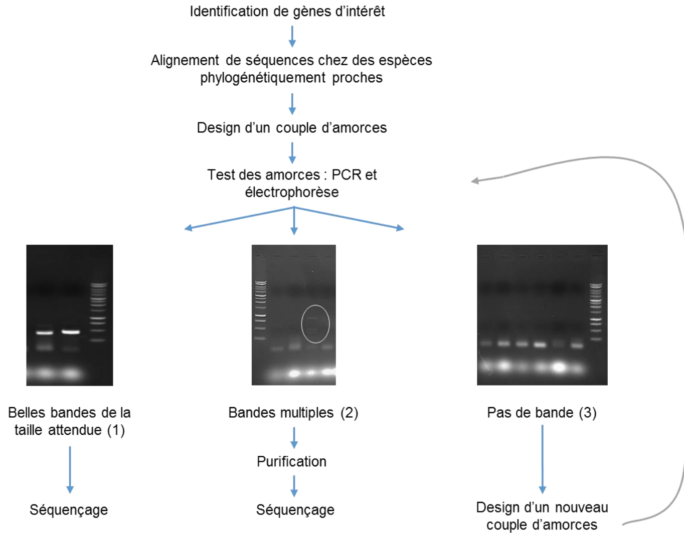
Figure II. 11 Travail préliminaire à la définition des amorces pour cibler des gènes d'intérêts en Q-PCR. (1) : les amorces testées ciblent uniquement la séquence d'intérêt et permettent son amplification spécifique; (2) : les amorces testées ciblent la séquence d'intérêt et des séquences autres, ne permettant pas une amplification spécifique; (3) : les amorces testées ne permettent pas l'amplification de la séquence d'intérêt. Il faut donc définir de nouvelles amorces.
