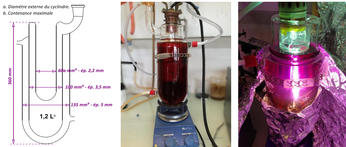
Figure 22 – Montage : réacteur de photolyse en Pyrex®
