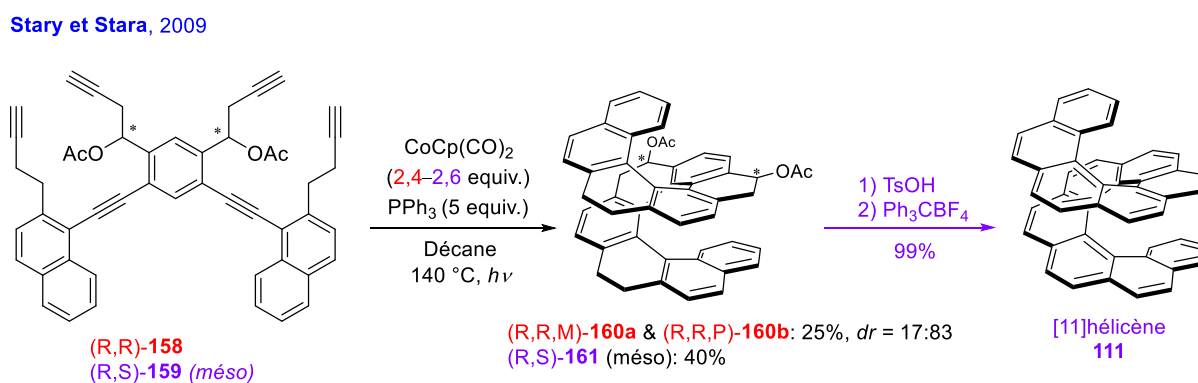
Schéma 38 – Accès au [11]hélicène par cyclotrimérisation catalysée au cobalt.
