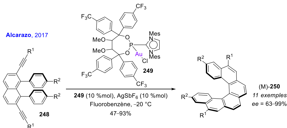
Schéma 59 – Catalyse à l'or, synthèse asymétrique de [6]héliènes.
