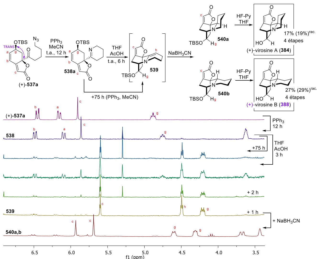
Schéma 130 – Synthèse des (+)-virosoines A ( 384 ) et B ( 388 )
