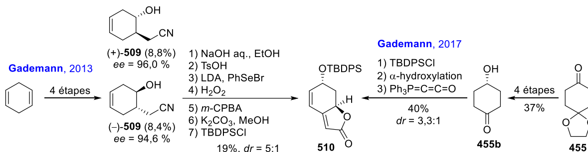
Schéma 114 – Synthèses de l'aquilégiolide TBDPS-protégé 510 .
