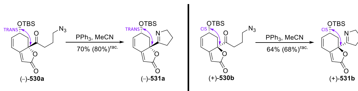
Schéma 126 – Séquence Staudinger/aza-Wittig. Synthèse des imines 531a et 531b .
