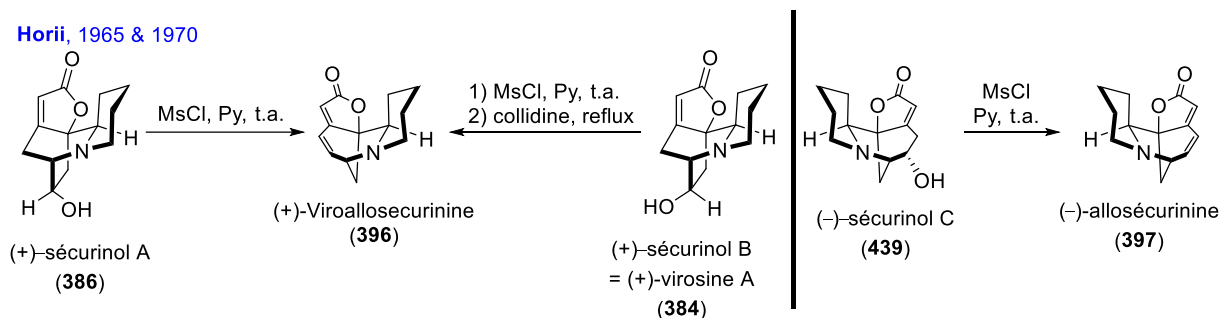
Schéma 99 – Réarrangements des sécurinols A (386) et B (384) et déshydratation du sécurinol C (439).
