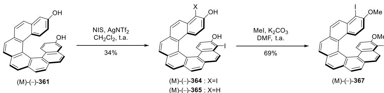
Schéma 90 – Iodation du bis-phénol hélicénique (M)- 361 , éthérification des phénols.
