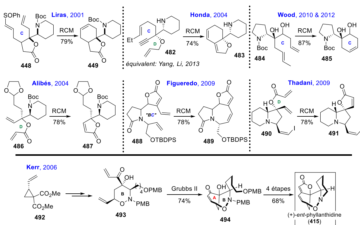
Schéma 109 – Méthathèse cyclisante et synthèses d'alcaloïdes de Securinega .
