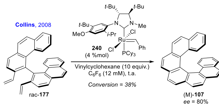
Schéma 57 – Métathèse cyclisante asymétrique pour la synthèse du [7]helicène.
