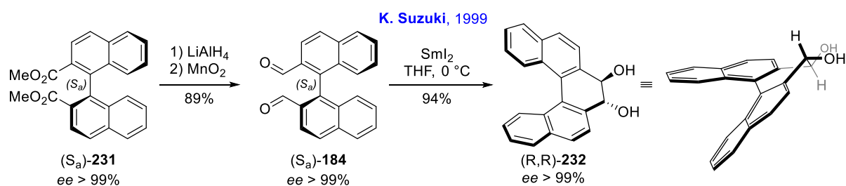
Schéma 53 – Couplage pinacolique et synthèse d'un [5]hélicénoïde énantio-pur.
