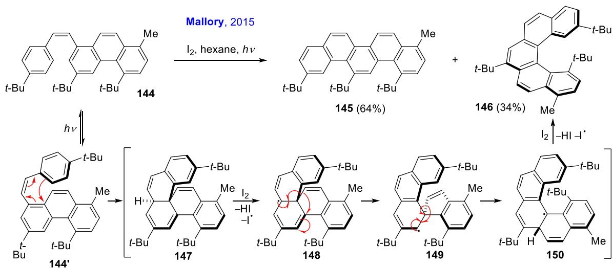
Schéma 34 – Réarrangement du squelette carboné dans les conditions de photocyclisation.
