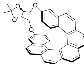
(S,S,P)-(+)-353P
