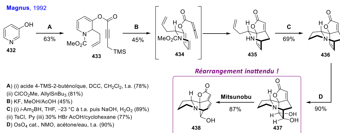
Schéma 98 – Découverte formelle du réarrangement des néonorsécurinanes.
