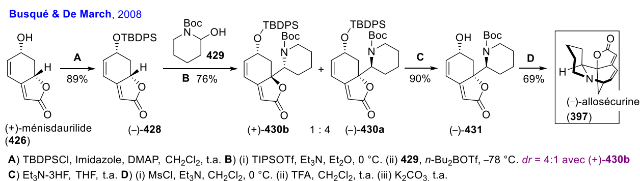
Schéma 97 – Proposition de Busqué et De March. Synthèse asymétrique de l'allosécurinine.
