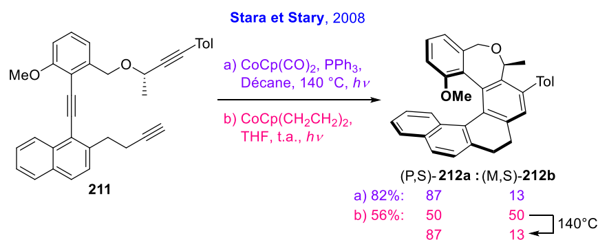
Schéma 47 – Diastérocontrôle en cycloisomérisation [2+2+2] d'alcynes.
