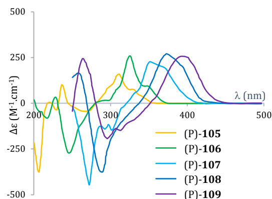
Figure 17 – Spectres CD expérimentaux des [5–9]héliènes. [80]
