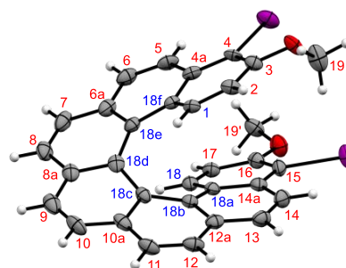
ORTEP
