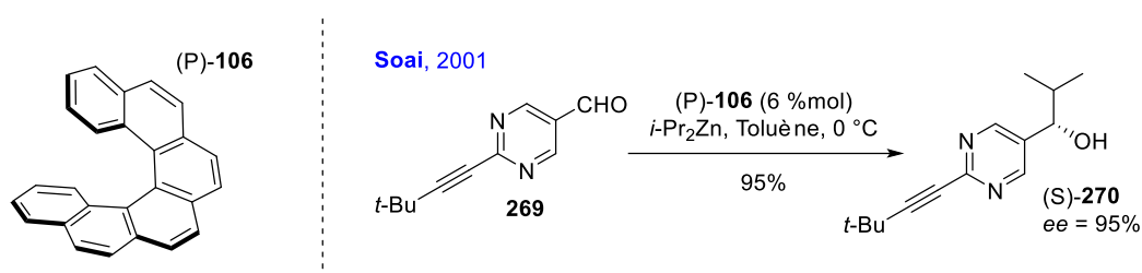
Schéma 64 – Induction de chiralité par un motif héliénique nu.
