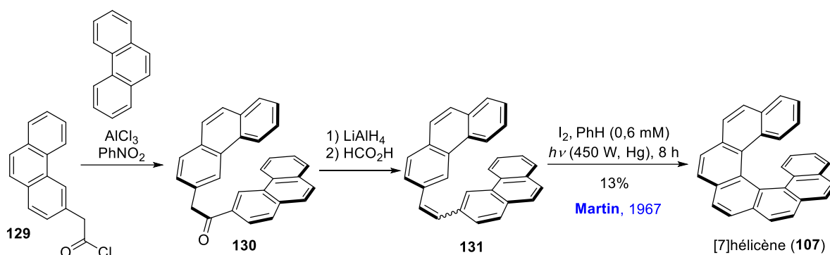
Schéma 28 – Synthèse du [7]héliène 107 par photocyclisation.
