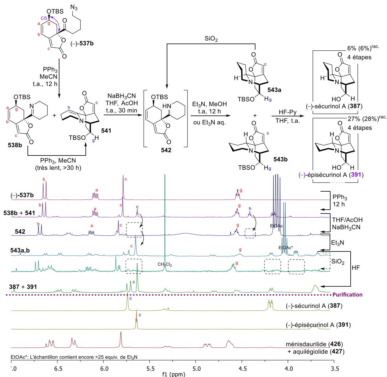
Schéma 131 – Synthèse des (-)-sécurinol A ( 387 ) et (-)-épisécurinol A ( 391 )
