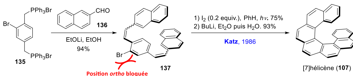
Schéma 30 – Synthèse améliorée du [7]héliène. Effet régiodirecteur du brome.
