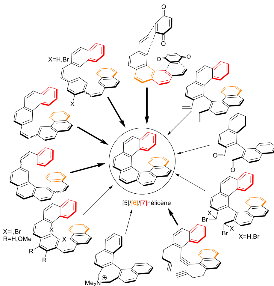
Schéma 27 – Méthodes d'accès aux motifs [5-7]héliçène
