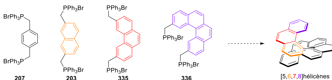
Figure 21 – Sels de phosphonium et cibles helicéniques.
