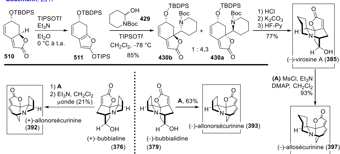
Schéma 116 – Synthèse totale de la (-)-viroisine A ( 385 ), Gademann (2017) et réarrangements vers le squelette (nor)sécurinane.
