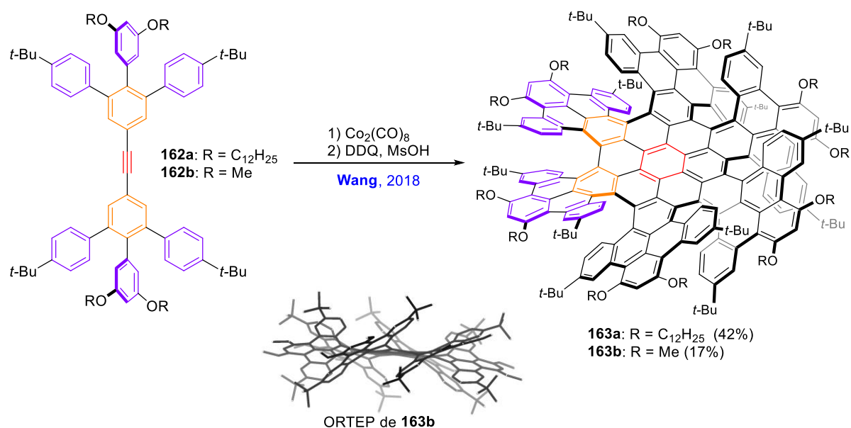
Schéma 39 – Synthèse du [7]héliène hexapôle 163 .
