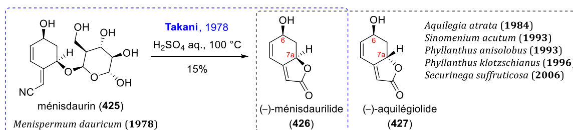
Schéma 96 - (-)-ménisdaurilide et (-)-aquiléiolide
