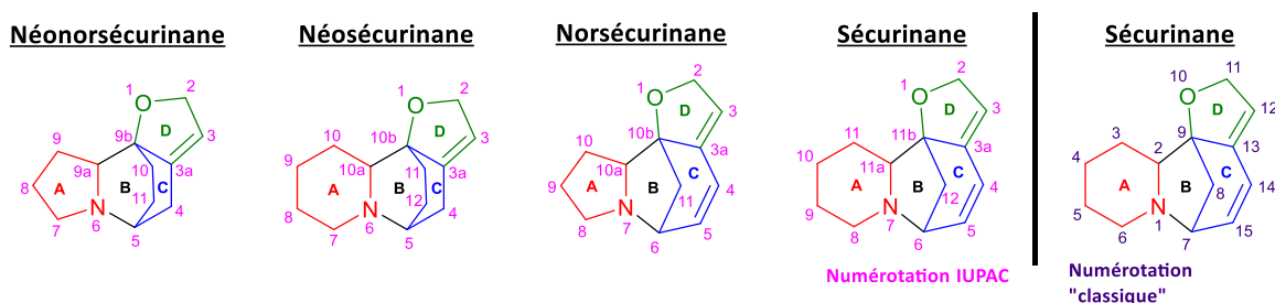
Figure 29 – Alcaloïdes de Securinega , sous classes et numérotation.
