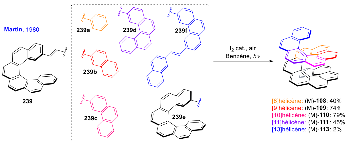
Schéma 56 – Synthèse des (M)-(-)-[8-11 & 13]helicènes.
