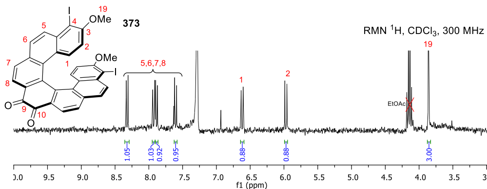
Figure 27 – RMN 1 H du sous-produit isolé de la réaction de désaromatation hydroxylante / tandem cycloaddition 4+2 du Carvacrol 371 . Attribution.
