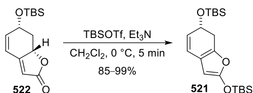
Schéma 120 – Formation du cétène-acétal silylé 521 .
