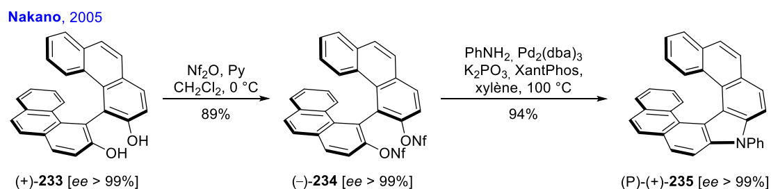
Schéma 54 – Synthèse de l'azahélicène énantio-pur ( P )- 235 .
