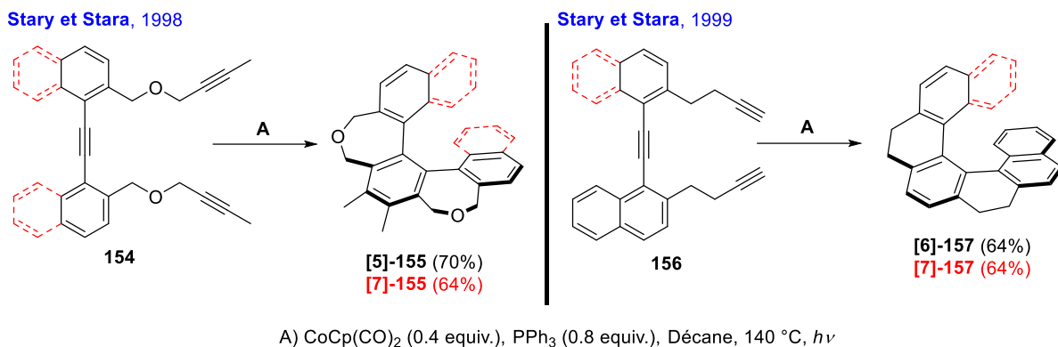
Schéma 37 – Synthèse d'hélicènes par cycloisomérisation [2+2+2] d'alcynes.
