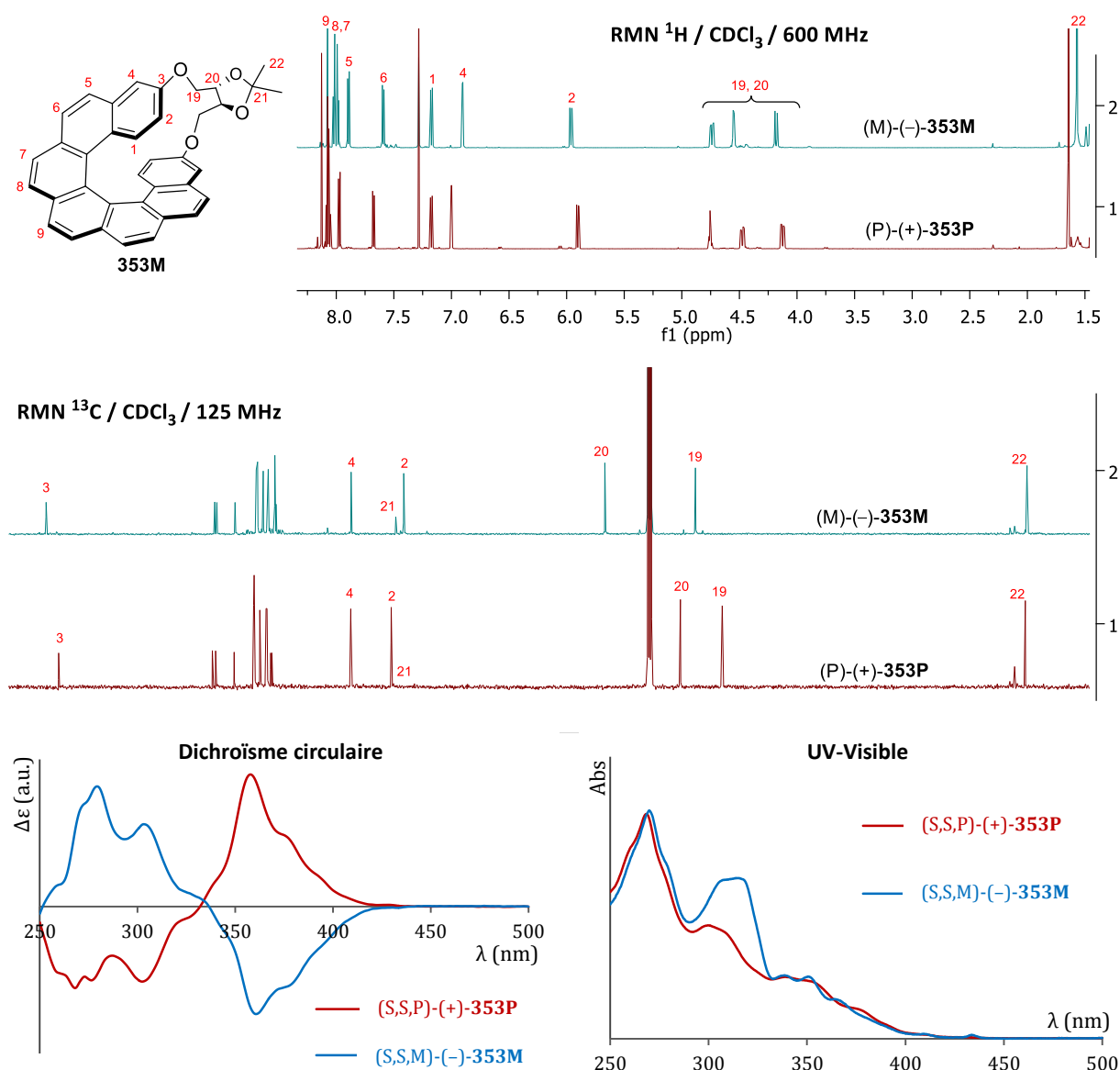
Figure 23 – Données de caractérisation RMN 1 H, RMN 13 C, CD, et UV-Vis des héliconoïdes optiquement purs (S,S,M)-(-)- 353M et (S,S,P)-(+)- 353P
