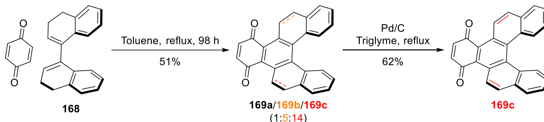
Schéma 40 – Synthèse d'un [5]héliène par Diels-Alder.
