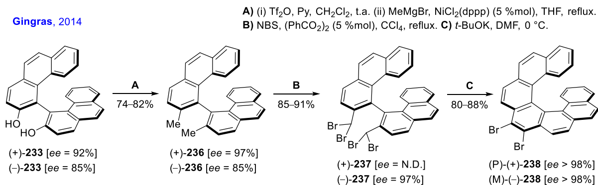
Schéma 55 – Synthèse asymétrique de [7]héliènes via un couplage benzylique.
