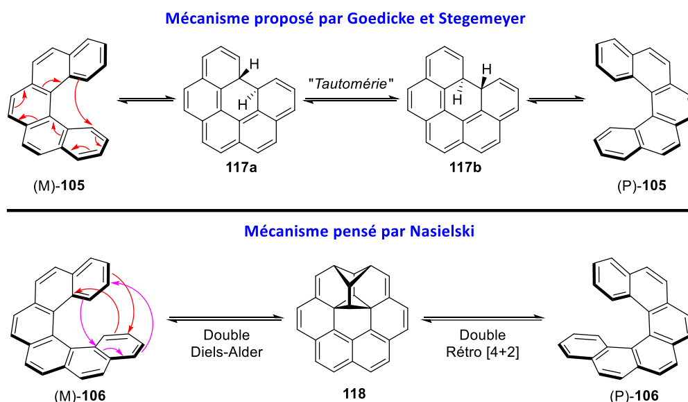
Schéma 23 – Propositions mécanistiques pour la racémisation des [5] & [6]héliènes ( 105 & 106 )
