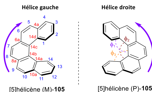
Figure 15 – (M)/(P)-[5]hélicène. Numérotation des carbones. Angles de torsion.
