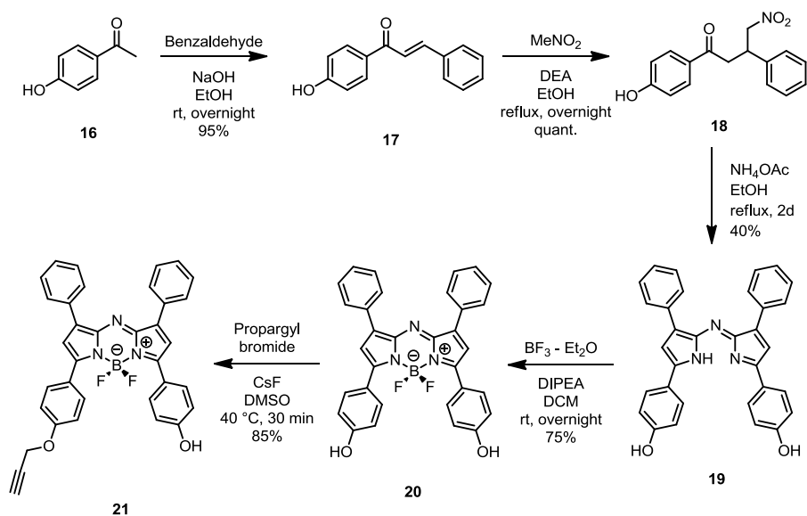
Figure 5 - Schéma de synthèse du tétraarylazadipyrrrométhène monopropargylé \text{BF}_2 -chélate 21 .
