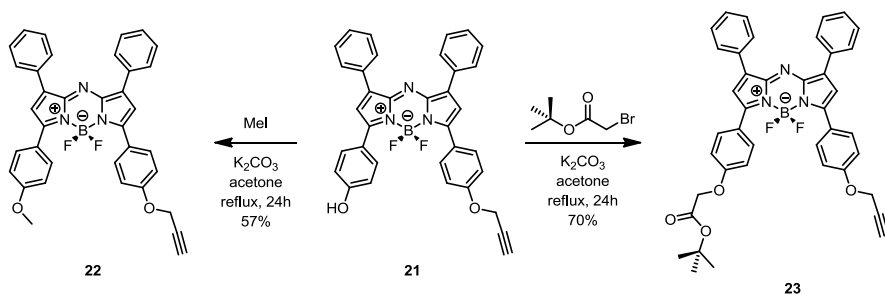
Figure R6 - Schéma de synthèse des deux tétraarylazadipyrrrométhène \text{BF}_2 -chélates asymétriques 22 et 23 .
