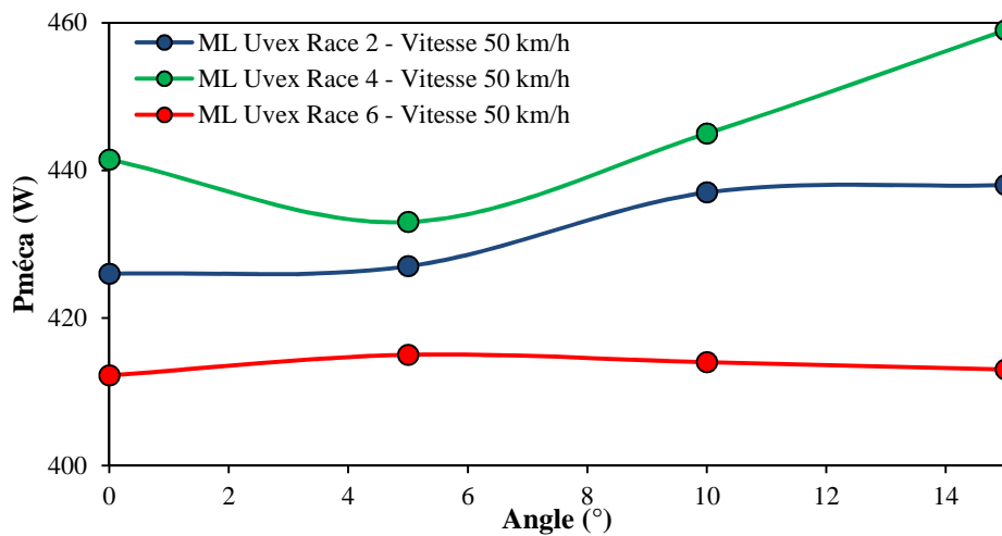
Figure 107 Relations P_{méca} – angle de vent de ML avec une vitesse de 50 km/h avec les casques Uvex Race 2, Race 4 et Race 6
