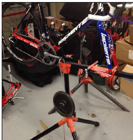
Figure 23 Etalonnage par une méthode statique du pédalier SRM
