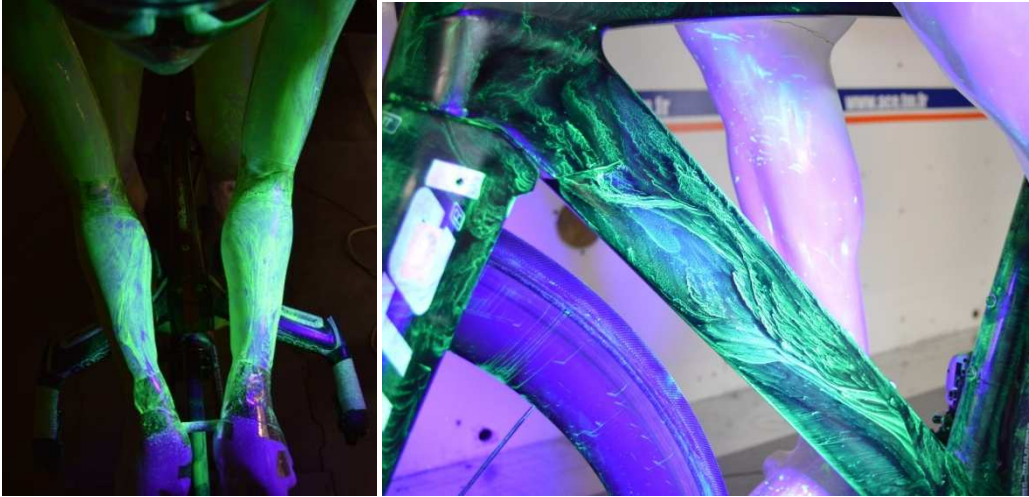
Figure 57 Visualisation des écoulements pariétaux
