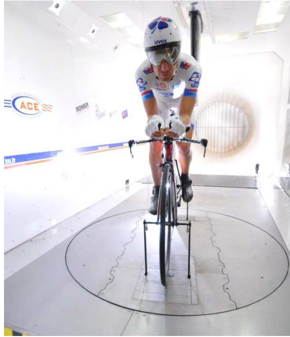
Figure 36 Veine d'essai de la soufflerie de Magny-Cours avec l'ensemble cycliste - vélo positionné sur la balance de force
