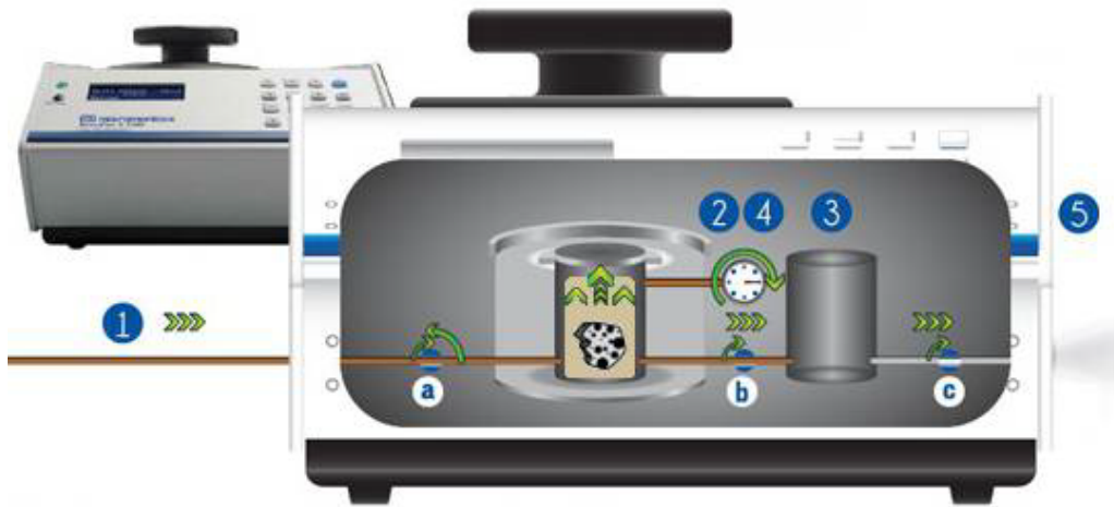
Figure 3.6 – Schéma montrant le fonctionnement de l'AccuPyc II 1340 de Micromeritics. Voir le texte ci-dessus pour la procédure expérimentale.
