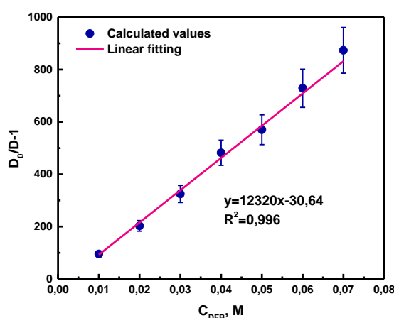
Figure 7 : Variations de [D_0/D-1] en fonction de la concentration totale de DFB ( 25^\circ\text{C} , I=0,7 \text{ M} , pC_H=1,5 ) et ajustement associé.
