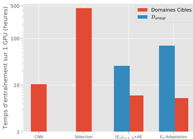
FIGURE 5.4.2 – Temps d'entraînement en heures (échelle logarithmique) avec un GPU P-100 pour différentes méthodes présentées dans cette section. Nous distinguons la phase d'entraînement non supervisée sur d_g en bleu et la phase d'entraînement pour chacune des connaissances cibles en rouge.
