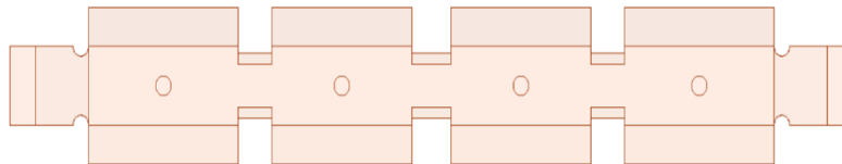
Figure III-26- Filtre 4 pôles
