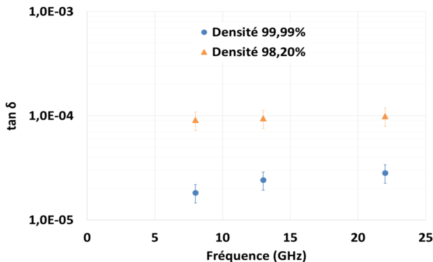
Figure II-29- Impact de la densité sur la tangente de pertes
