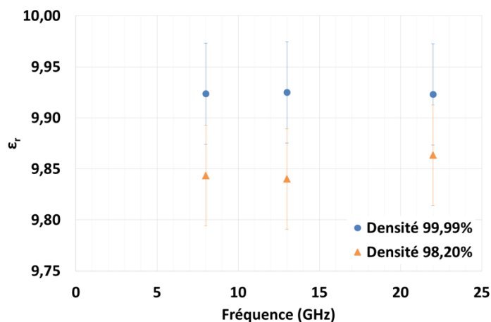
Figure II-28- Impact de la densité sur la permittivité
