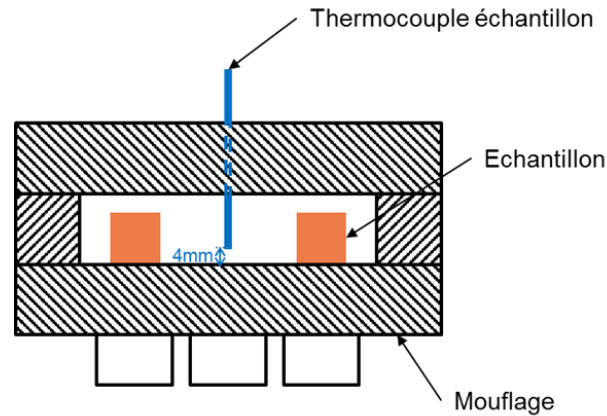
Figure II-20- Schéma du mouflage utilisé pour le frittage des échantillons
