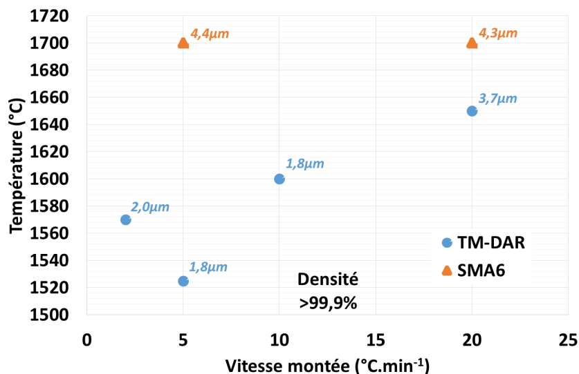
Figure II-21- Evolution de la température de frittage de la TM-DAR et de la SMA6 en fonction de la rampe de montée en température
