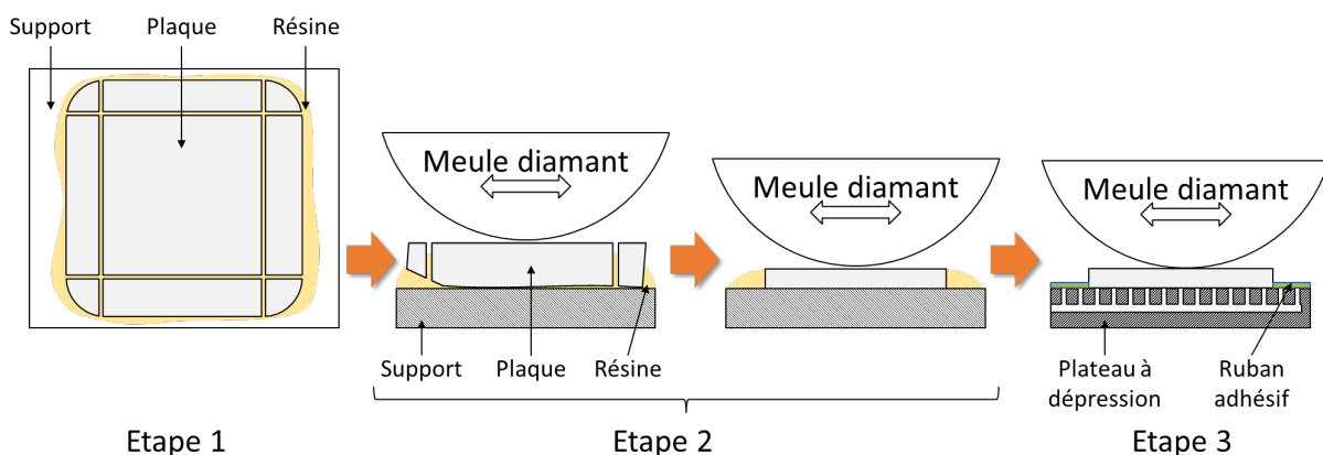
Figure II-25- Schéma représentant les étapes d'usinage des plaques
