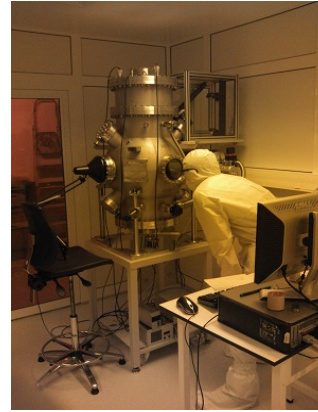
Figure IV-24- Bâti d'ablation laser Méca 2000 (PLD : Pulsed Laser Deposition) et panache d'ablation d'une cible de nickel
