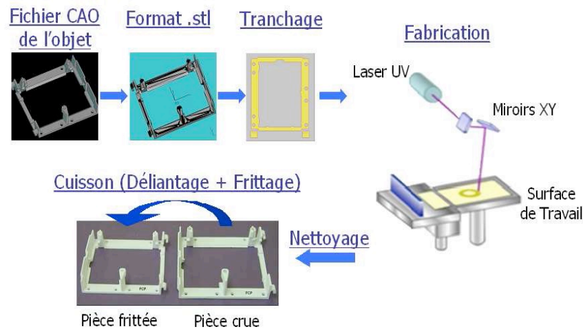
Figure I-46 - Principe de fabrication d'objets 3D céramiques par SLA 3D [38]
