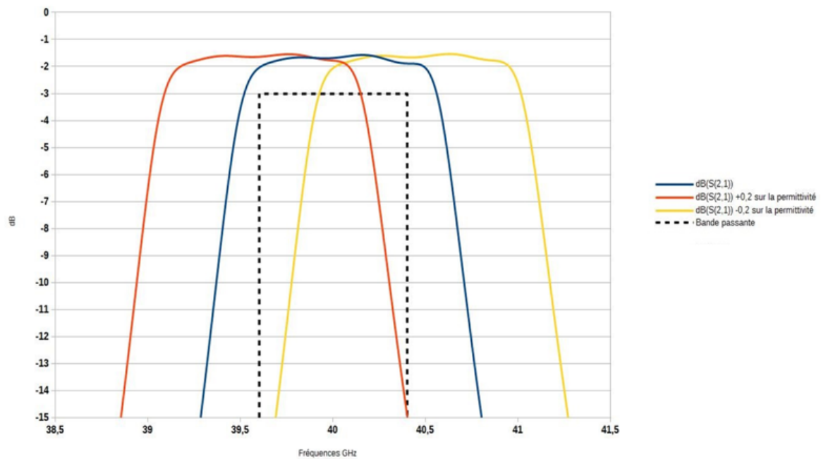
fig k- Zoom sur la variation dimensionnelle de \pm 1\% sur toute la structure filtre bande Q excitation micro ruban
