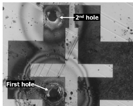
Figure IV-46- Trou dans la partie supérieure d'un résonateur planaire (diamètre 350\mu\text{m} ) [70]
