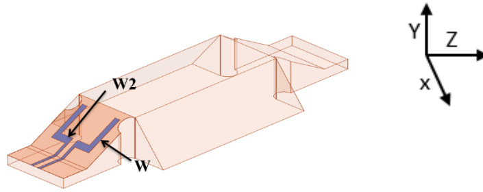
Figure III-13- Excitation coplanaire sur la pente
