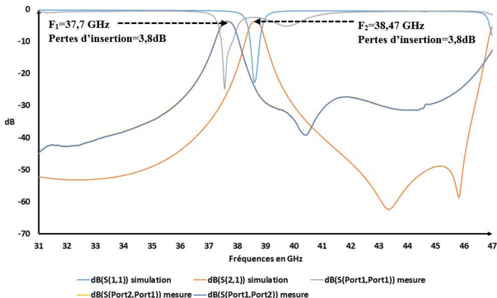
Figure IV-44- Comparaison simulation/ mesure filtre deux pôles bande Q
