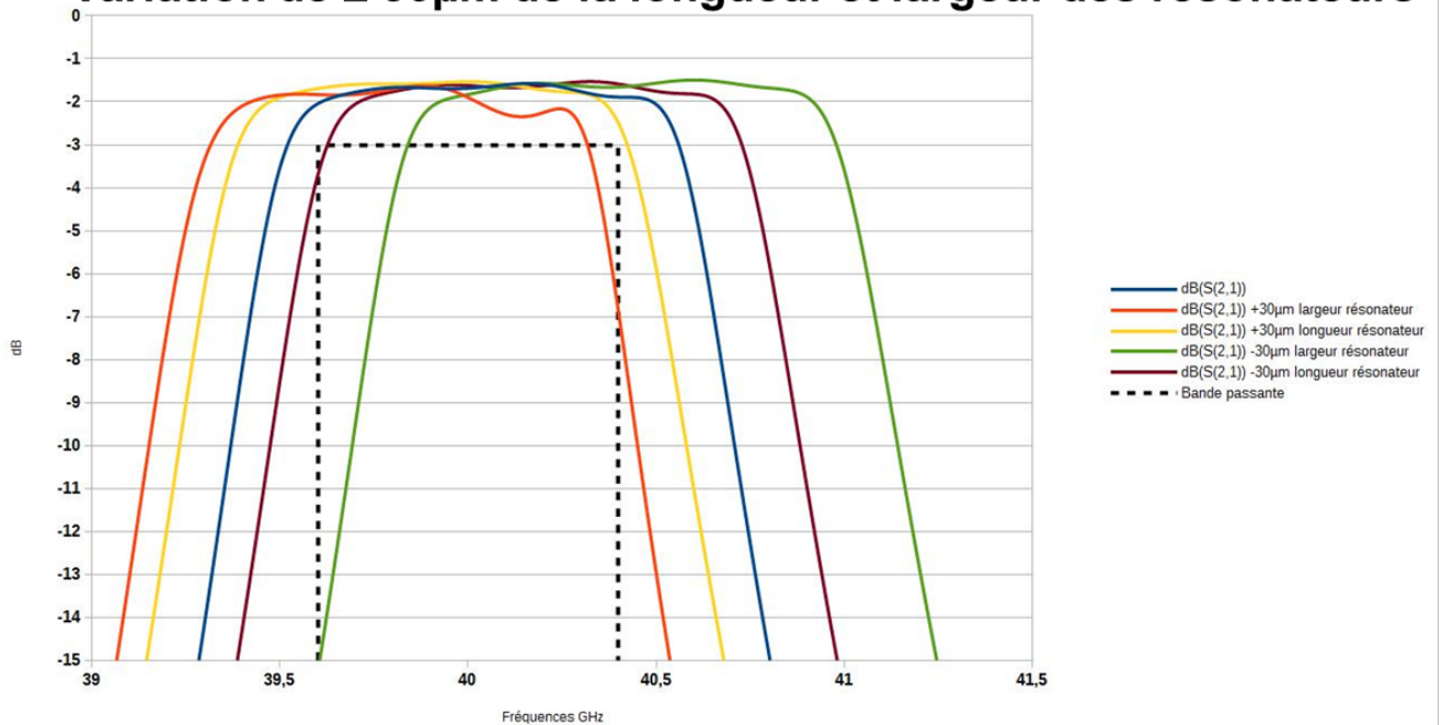
fig g- Zoom sur la dispersion dimensionnelle (Longueur-largeur des résonateurs) filtre bande Q excitation micro ruban
