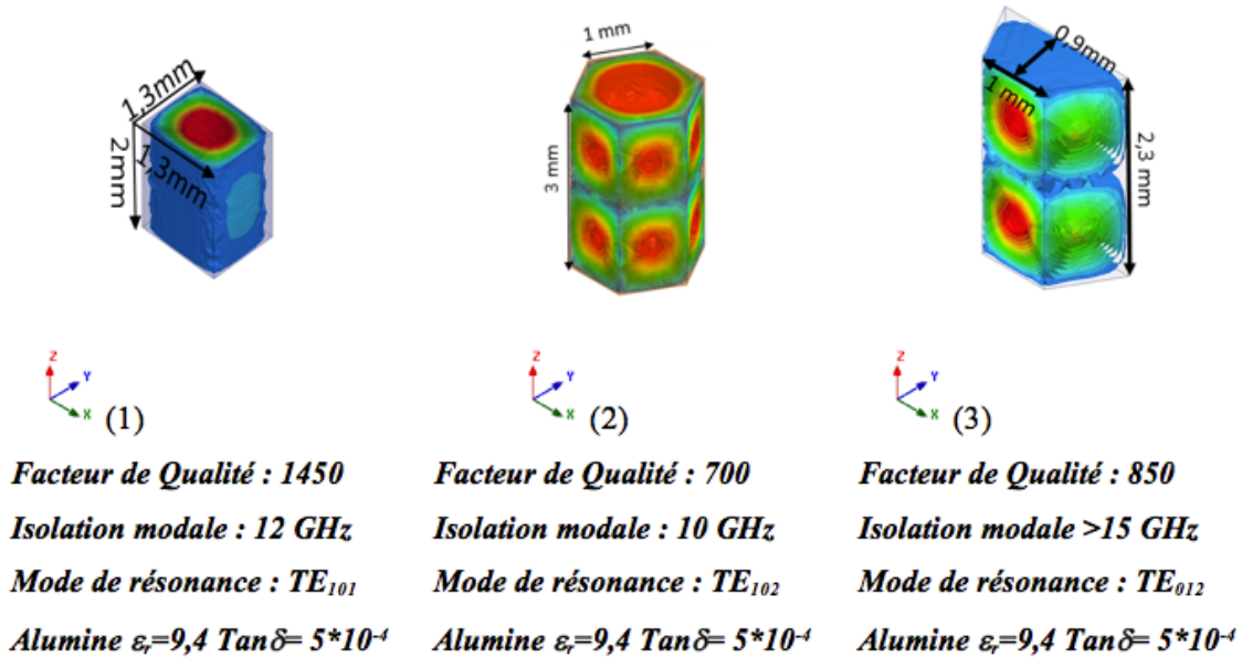
Figure III-5- Géométries des résonateurs étudiés
