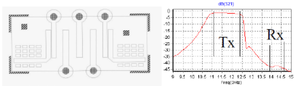
Figure I-9- Filtres interdigités [46]
