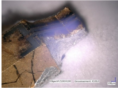
Figure IV-30- Utilisation de la laque d'argent pour couvrir les zones non métallisées
