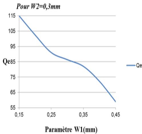
Figure III-11- Variation du facteur de qualité extérieur Q_e en fonction du paramètre W_1
