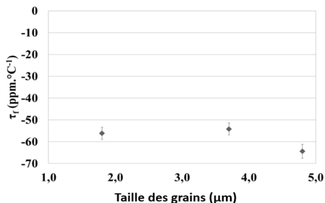
Figure II-32- Impact de la taille des grains sur le facteur de température
