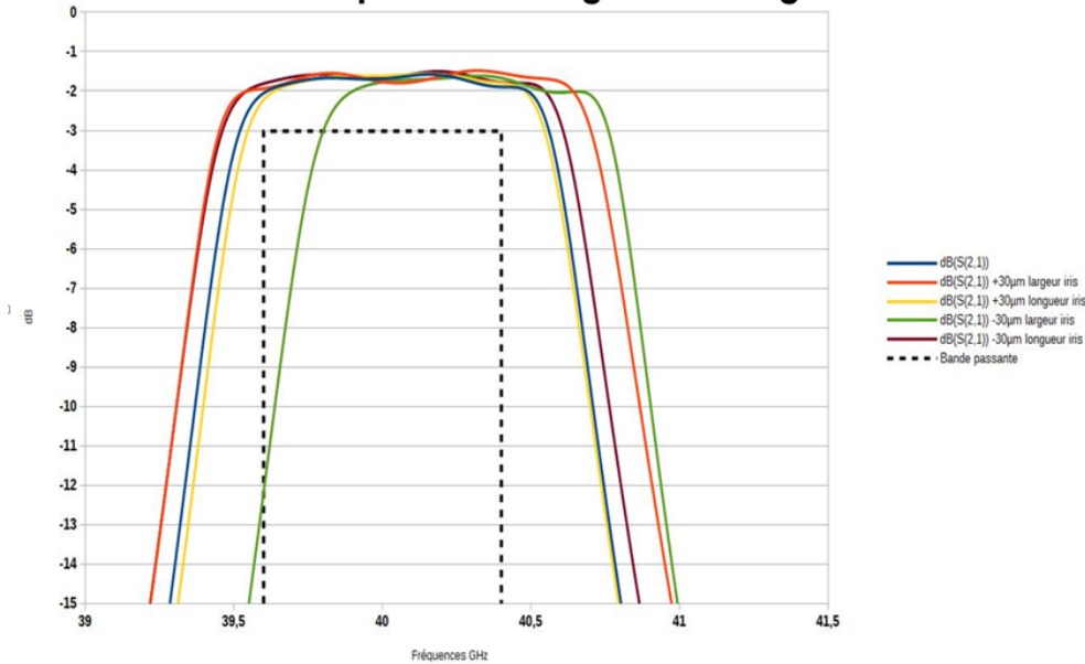
fig i- Zoom sur la dispersion dimensionnelle (Longueur-largeur des iris) filtre bande Q excitation micro ruban
