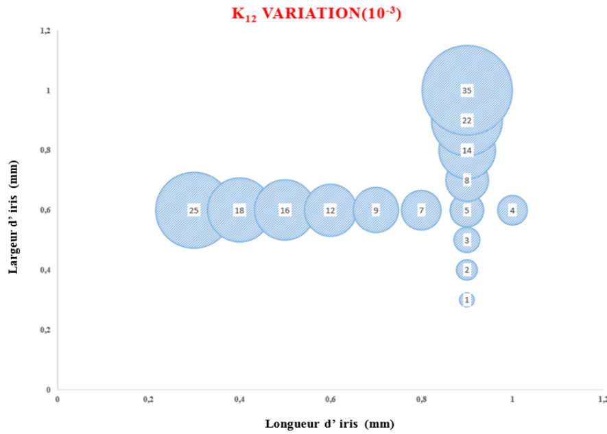
Figure III-21- Variations de K_{12} en fonction des variations dimensionnelles de l'iris de couplage
