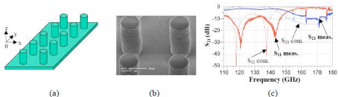
Figure I-48 - (a) Vue 3D du cristal ; (b) Photographie SEM de quatre cylindres ; (c) Réponses simulées et mesurées correspondantes [41]
