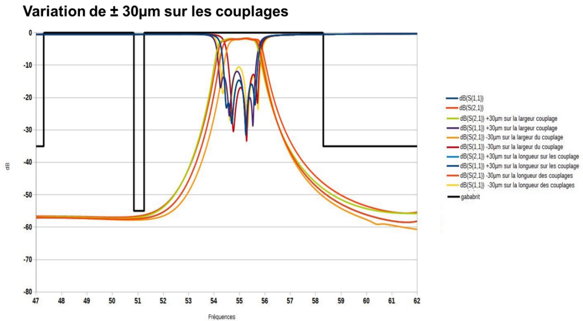
fig o- Dispersion dimensionnelle (Longueur-largeur des iris) filtre bande V excitation micro ruban
