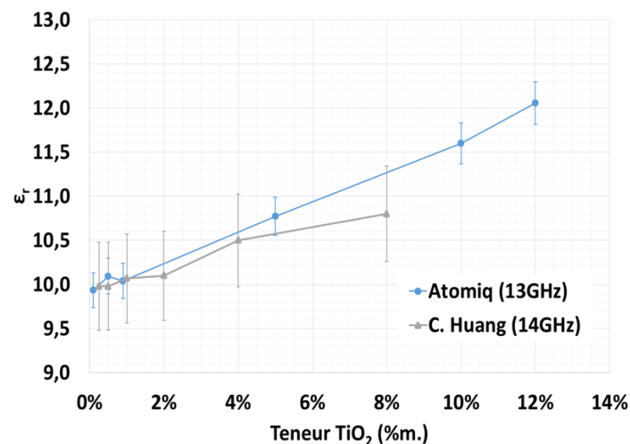
Figure II-44- Comparaison des permittivités des aluminés dopés sans recuit à la littérature [53]
