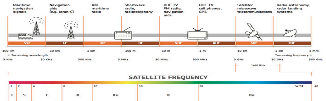
Figure I-1- Bandes de fréquences pour les satellites de télécommunication [1]
