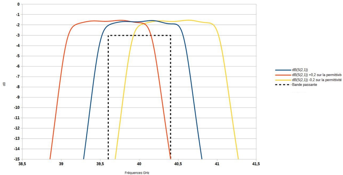
fig e- Zoom sur S21 du filtre bande Q excitation micro ruban avec une dispersion de permittivité de \pm 0,2
