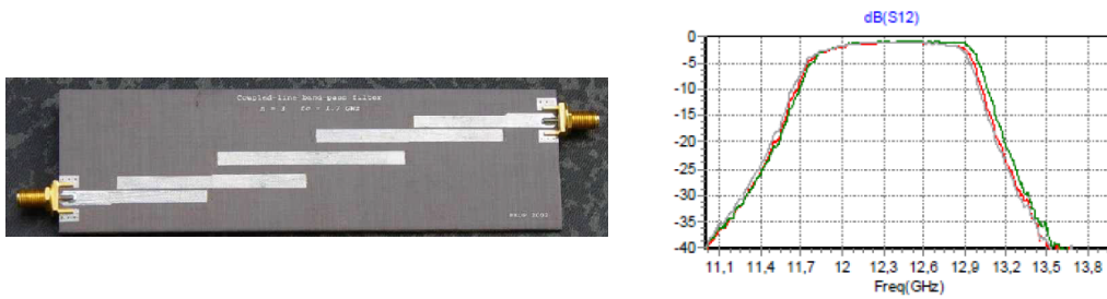
Figure I-6- Filtre à lignes couplées [46]
