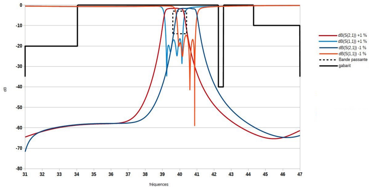
fig j- Variation dimensionnelle de \pm 1\% sur toute la structure filtre bande Q excitation micro ruban
