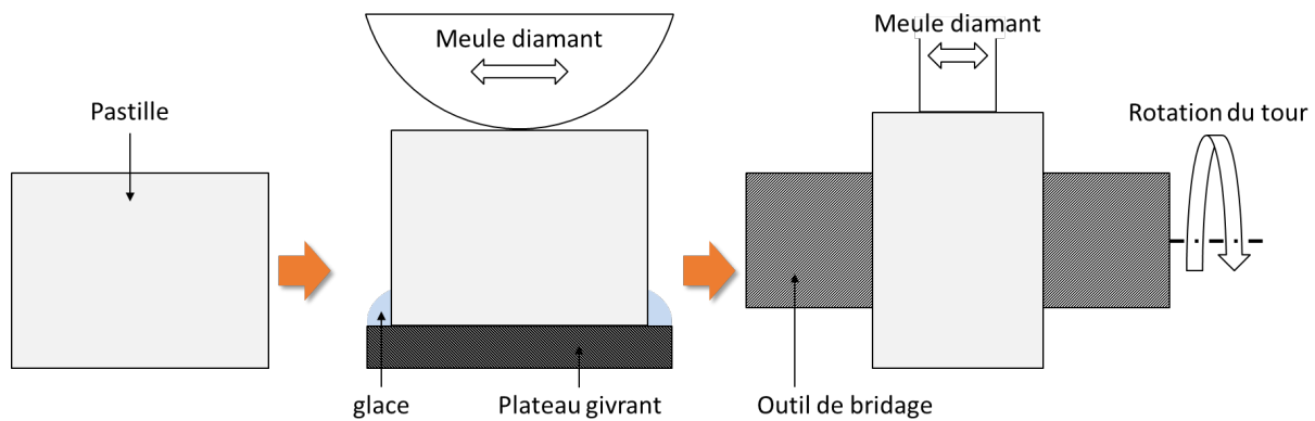
Figure II-24- Schéma des étapes d'usinage des cylindres
