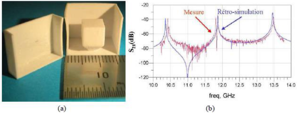
Figure I-47- Résonateur monobloc (a), Comparaison simulation/mesure (b) [40]
