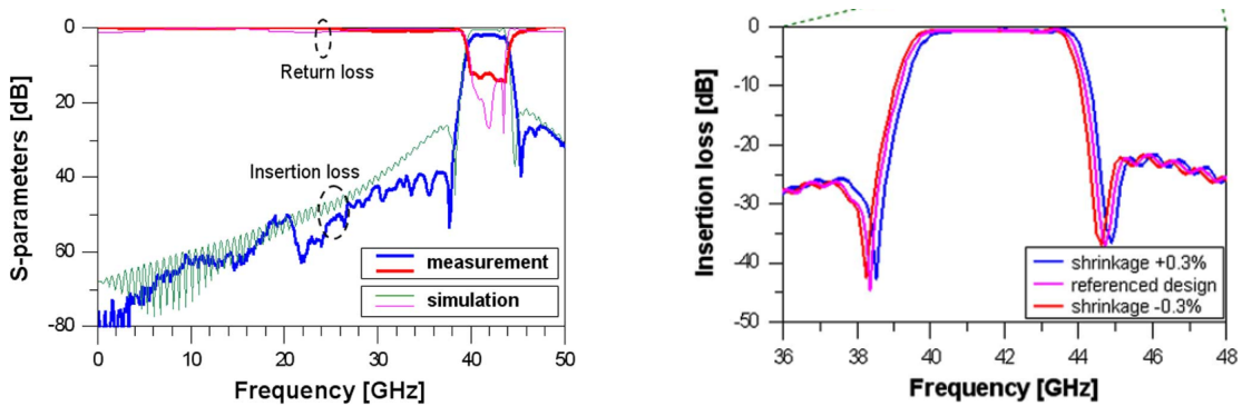
Figure I-22 – Comparaison des réponses fréquentielles simulée et mesurée – étude de dispersion technologique [24]
