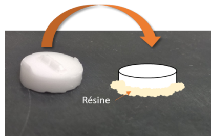
Figure IV-4- Mise en place et collage du filtre pour l'étape de rectification
