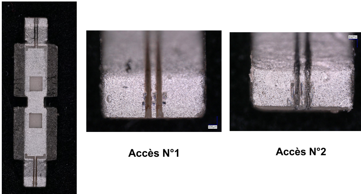
Figure IV-62- Motifs de correction sur un filtre deux pôles (fabriqué par 3DCeram)
