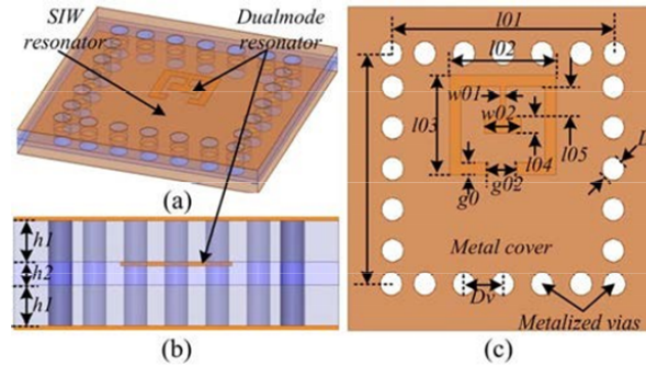
Figure I-27- (a) Layout du filtre hybride – (b) Vue 3D de la coupe transversale de la structure – (c) Vue du dessus [27]
