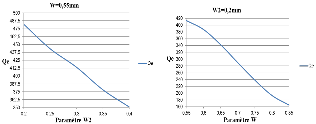
Figure III-13- Excitation coplanaire sur la pente
