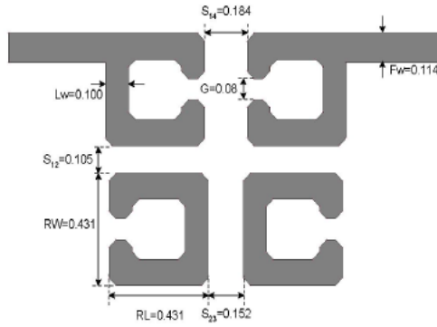
Figure I-13- Vue de dessus du filtre 4 pôles quasi-elliptique [20]
