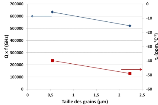
Figure II-6- Impact de la taille de grains sur les facteurs de qualité et température [51-52]
