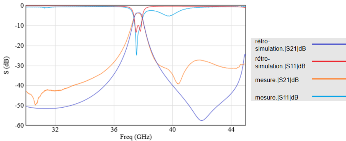
Figure IV-45- Rétro-simulation filtre deux pôles bande Q
