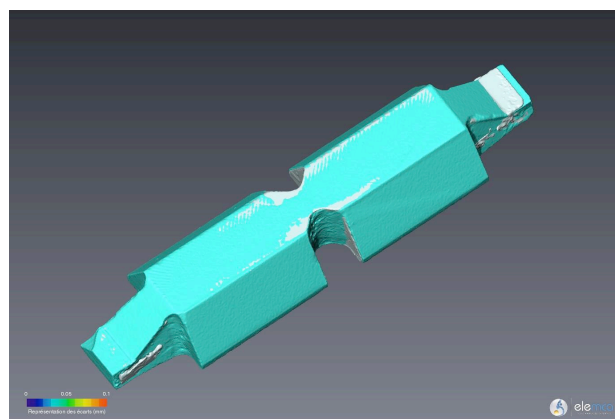
Figure IV-18- Alignement des surfaces de chaque objet
