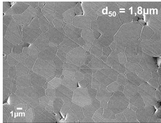
Figure II-22- Microstructure de la TM-DAR après frittage à 1525^{\circ}\text{C} ( 5^{\circ}\text{C}\cdot\text{min}^{-1} )
