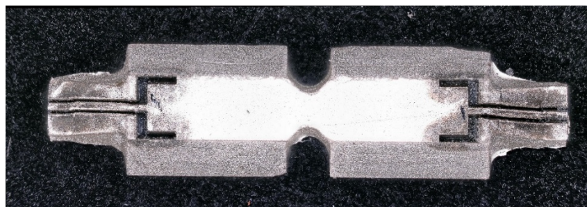
Figure IV-33- Métallisation argent et gravure des accès
