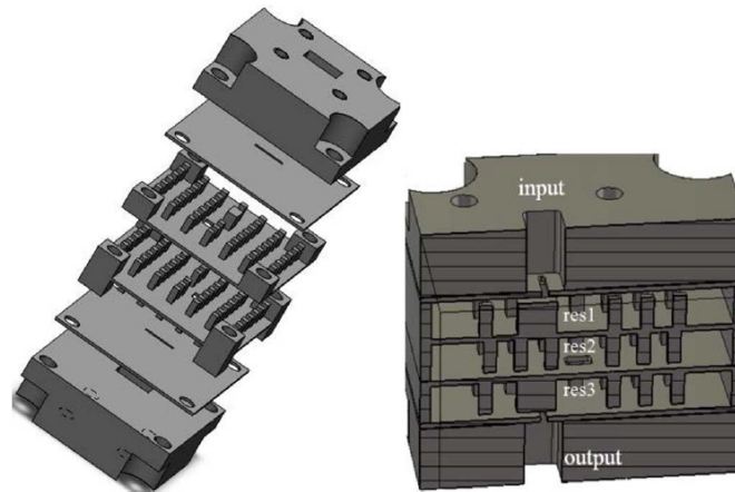
Figure I-32- Structure du filtre à base de résonateurs empilés [29]
