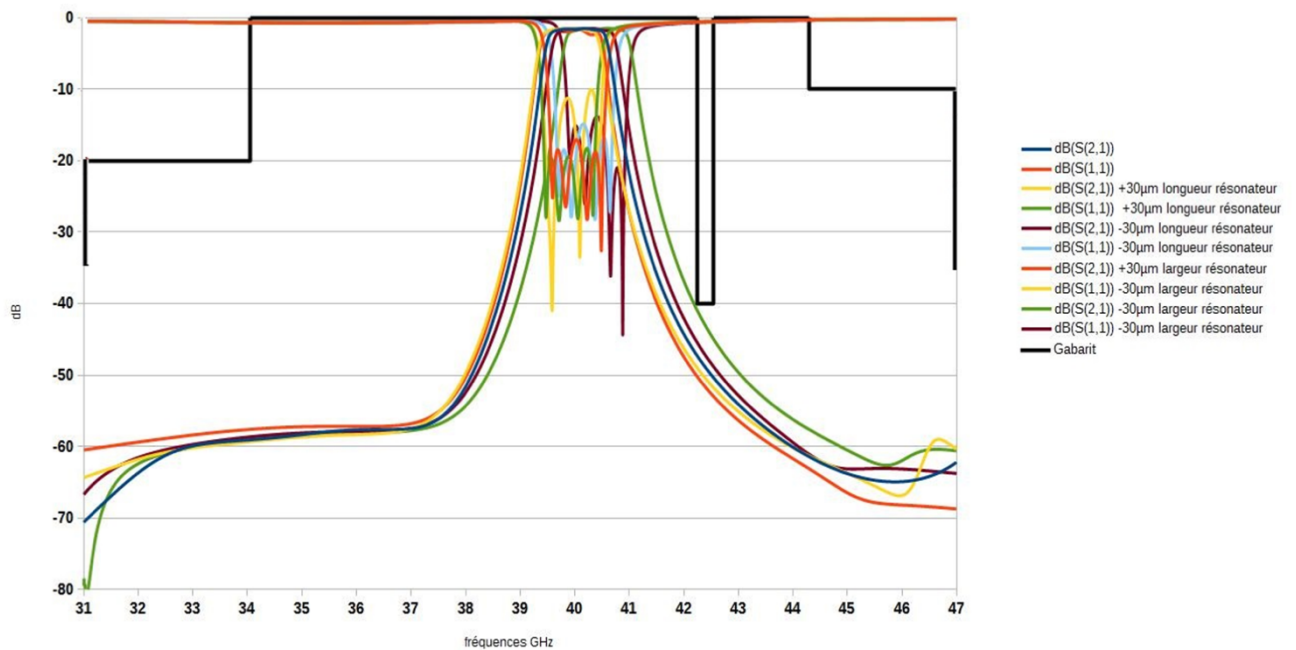
fig f- Dispersion dimensionnelle (Longueur-largeur des résonateurs) filtre bande Q excitation micro ruban
