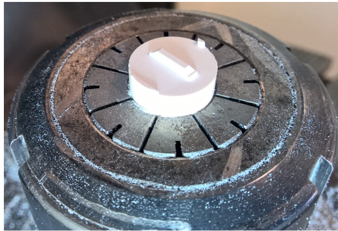
Ebauche de filtre après la première étape d'usinage.
