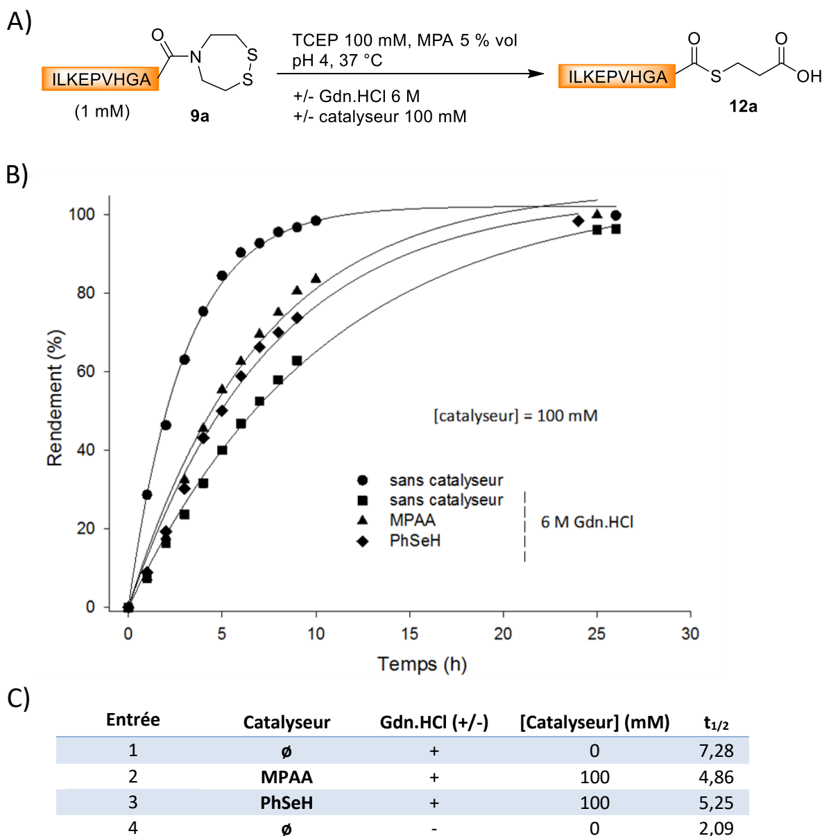
Figure 74 : A) Réaction d'échange du peptide 9a avec le MPA. B) Suivi cinétique HPLC ( \lambda = 215 nm) de la réaction d'échange. Les données sont corrélées par une loi d'ordre 1. C) Tableau des temps de demi-réaction pour les différentes conditions.
