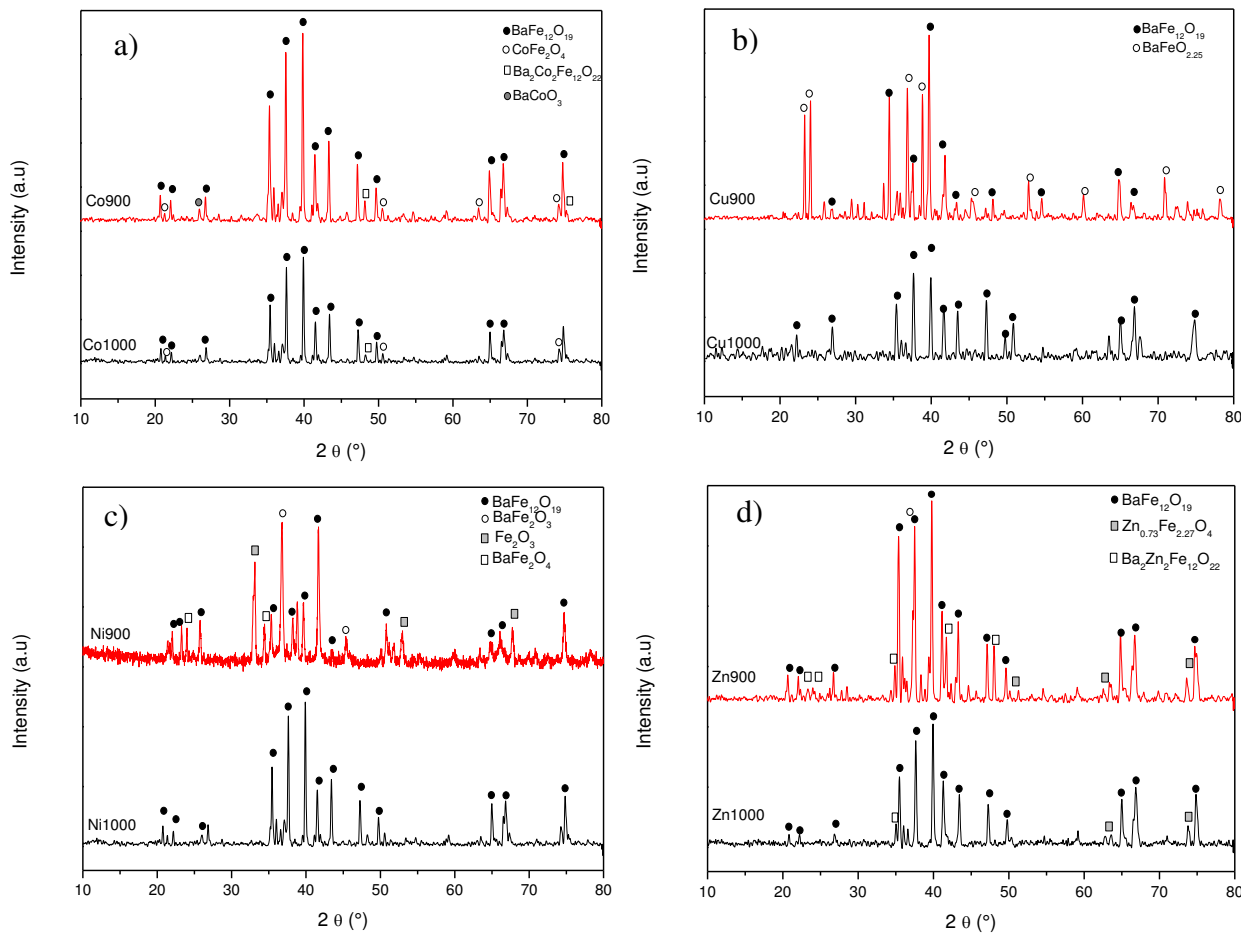
Figure III. 21. Diffractogrammes des rayons X des échantillons: a) BaCoFe 11 O 19 , b) BaCuFe 11 O 19 , c) BaNiFe 11 O 19 , et d) BaZnFe 11 O 19 calcinés à différentes températures
