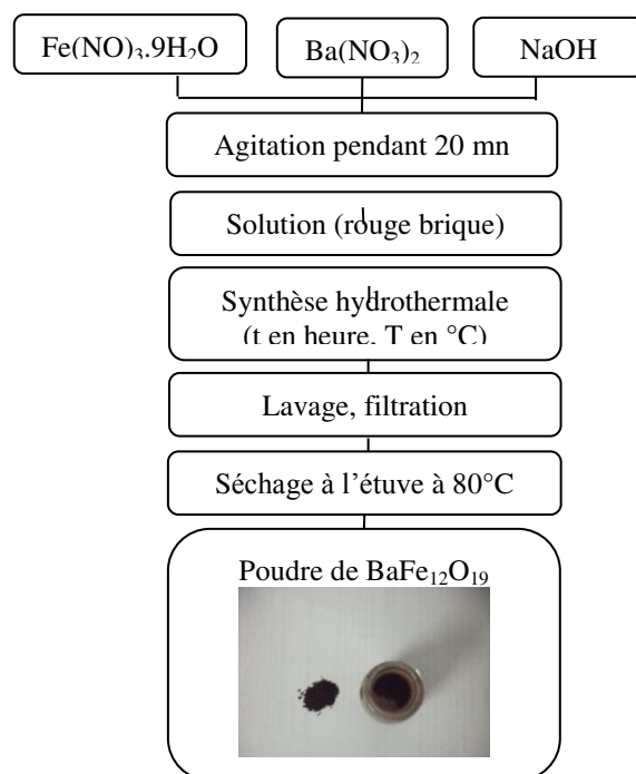
Figure III. 1. Organigramme de la synthèse du BaFe 12 O 19
