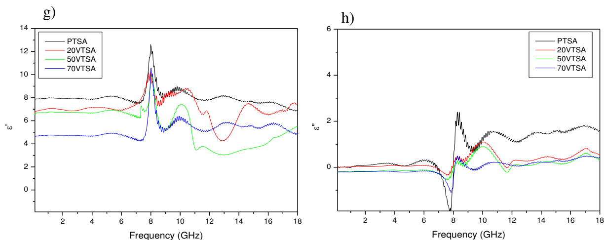
Figure V. 12. Évolution des spectres de permittivité réelle et imaginaire des composites Polyaniline/ \text{BaFe}_{12}\text{O}_{19} synthétisés en présence de HCl (a et b) ; CSA (c et d) ; NSA (e et f) et TSA (g et h)
