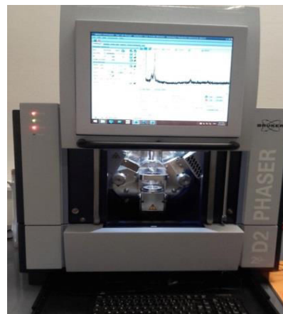
Figure II. 3. Diffractomètre Bruker D2 phaser 2 nd Gen
