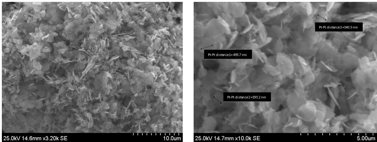
Figure III. 15. Images MEB du \text{BaFe}_{12}\text{O}_{19} synthétisée par voie hydrothermale dynamique Les spectres obtenus de l'analyse élémentaire quantitative EDX pour les échantillons préparés par voie statique et dynamique sont représentés sur les figures III. 16 et III. 17.
