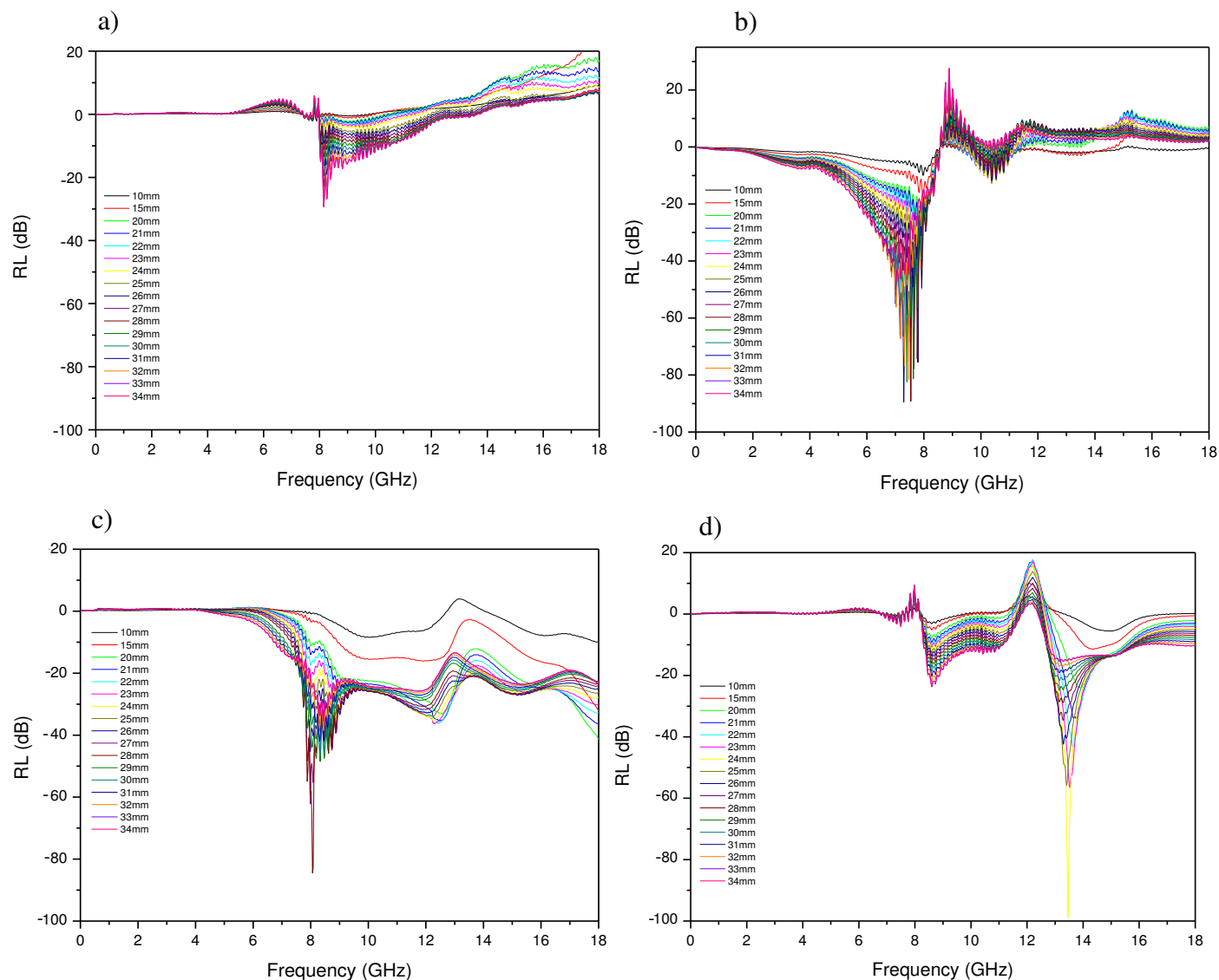
Figure V. 16. L'évolution du coefficient de réflexion en fonction de la fréquence de (a) PNSA, (b) 20VNSA, (c) 50VNSA et (d) 70VNSA
