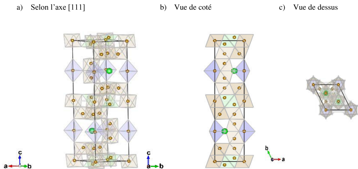
Figure I. 23. Représentation perspective de la structure hexagonale de BaFe_{12}O_{19}
