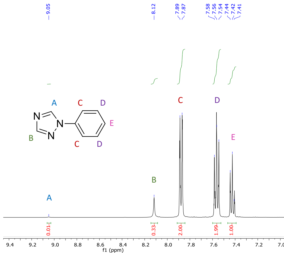
Figure A57 : Spectre RMN ^1\text{H} (400 MHz, \text{CDCl}_3 ) du 1-phenyl-1,2,4-triazole après 24 h de réaction à 55 °C dans le THF, sous 2 bars de \text{D}_2 avec les NPs de \text{Ni@IMes} .
