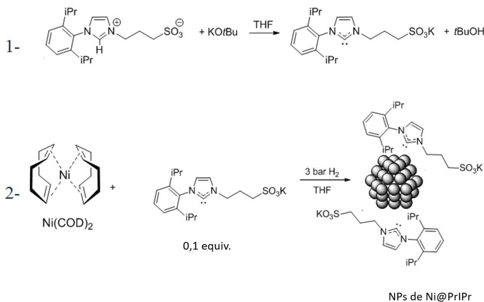
Figure 169 : Synthèse des NPs de Ni hydrosolubles par l'approche organométallique.
