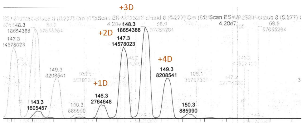
Figure A56 : Spectre MS du 2-phénylimidazole après 24 h de réaction à 55 °C dans le THF, sous 2 bars de \text{D}_2 avec les NPs de Ni@IMes.
