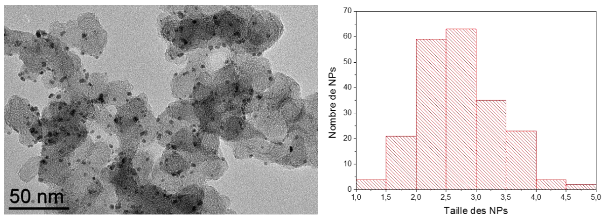
Figure 97 : Image MET des NPs de Ru/C (27 wt%) et l'historgramme correspondant.
