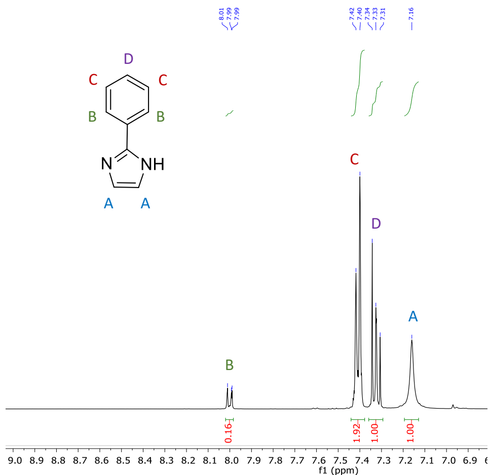
Figure A55 : Spectre RMN ^1\text{H} (400 MHz, \text{CDCl}_3 ) du 2-phénylimidazole après 24 h de réaction à 55 °C dans le THF, sous 2 bars de \text{D}_2 avec les NPs de Ni@IMes.
