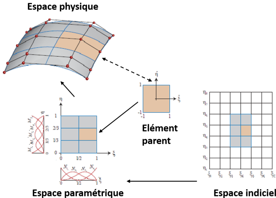
FIGURE 1.7 – Les différents espaces intervenant dans l'AIG pour un maillage constitué de 2 \times 3 éléments quadratiques (inspiré de [82]). L'espace indiciel est l'espace de définition des vecteurs nœuds tandis que les fonctions B-Splines sont définies dans l'espace paramétrique localisé sur l'ensemble du patch. L'intégration est réalisée sur un élément parent puis transmise dans le domaine physique.
