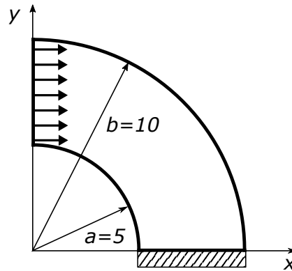
FIGURE 6.7 – Définition du problème et de ses conditions aux limites.
