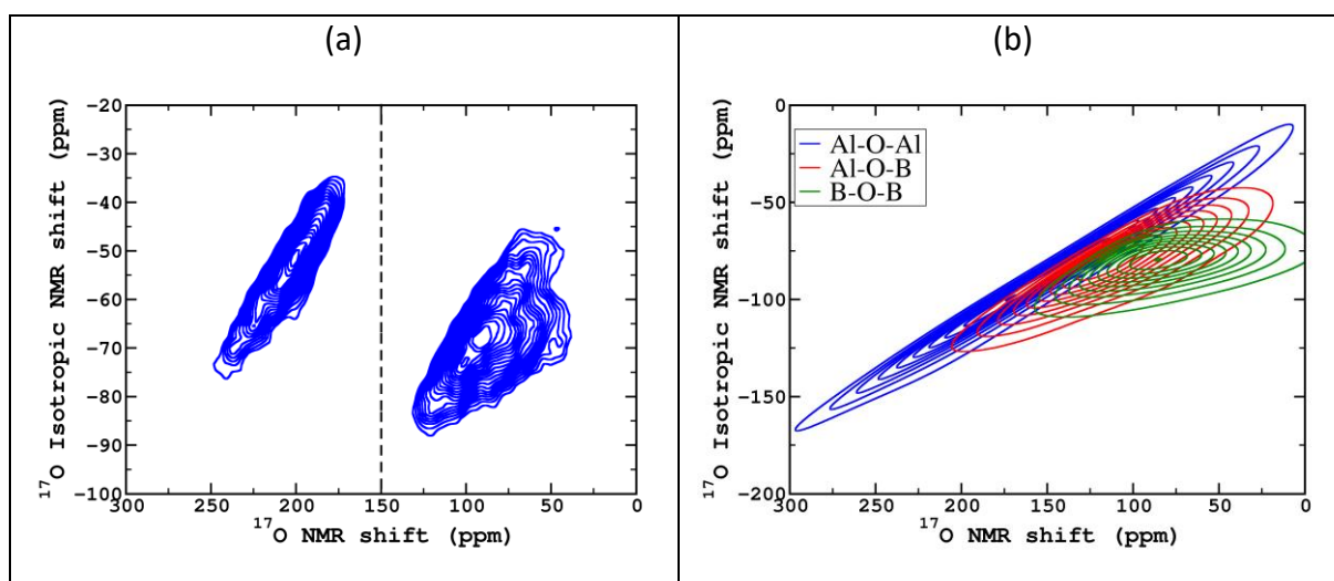
Figure V-14 : spectre MQMAS ^{17}\text{O} expérimental (a) ; ce même spectre simulé en distinguant les différents sites T-O-T (b)
