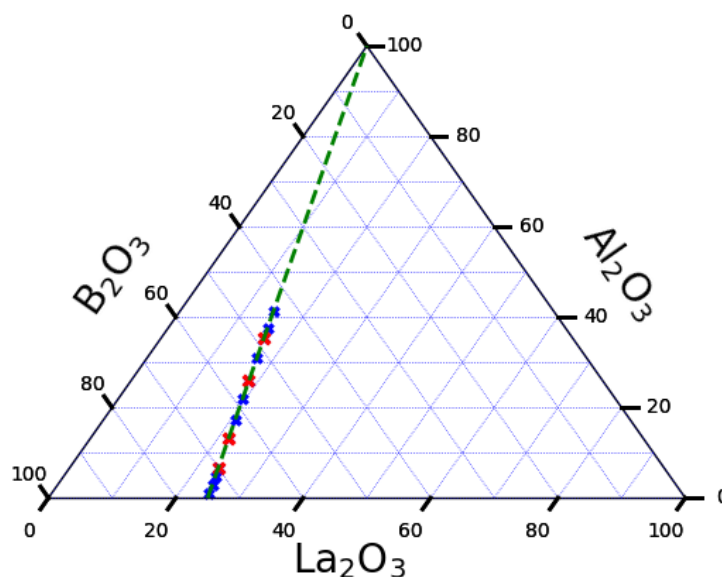
Figure IV-2: diagramme ternaire B_2O_3 - La_2O_3 - Al_2O_3 , la ligne verte représente la ligne de substitution étudiée, les croix bleues sont les verres synthétisés et les croix rouges sont les verres enrichis en oxygène-17
