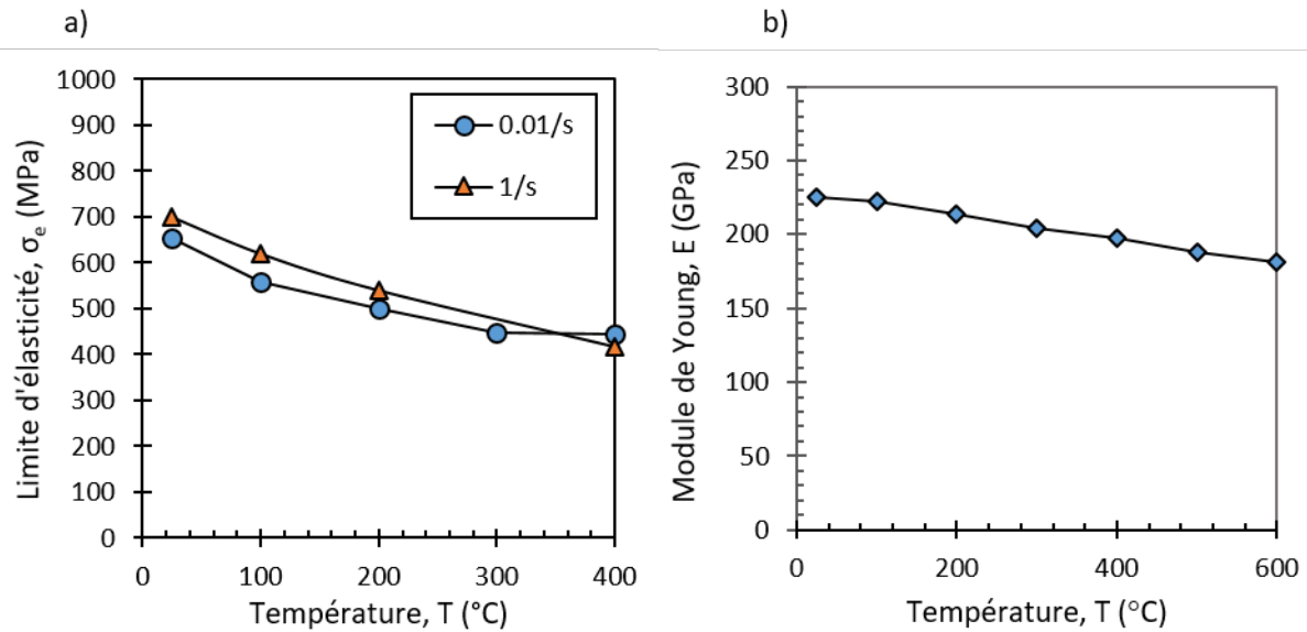
FIGURE 2.5 – a) Évolution de la limite d'élasticité du HS25 en fonction de la température pour deux taux de déformation ( 0.01\text{ s}^{-1} et 1\text{ s}^{-1} ), d'après [95]; b) évolution du module de Young en fonction de la température (d'après la documentation Haynes International [97])
