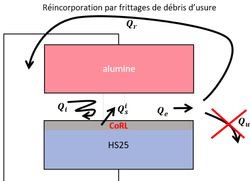
FIGURE 6.31 – Illustration du circuit tribologique appliqué à l'usure du contact HS25/alumine à haute température où une glaze layer efficace (CoRL) se forme à l'interface par tribo-frittage des débris d'usure. Q_s^i représente le débit source interne (formation de débris d'usure via la consommation de la couche d'oxyde), Q_i est le débit interne, Q_e est le débit externe, Q_u est le débit d'usure et Q_r est le débit de recirculation
