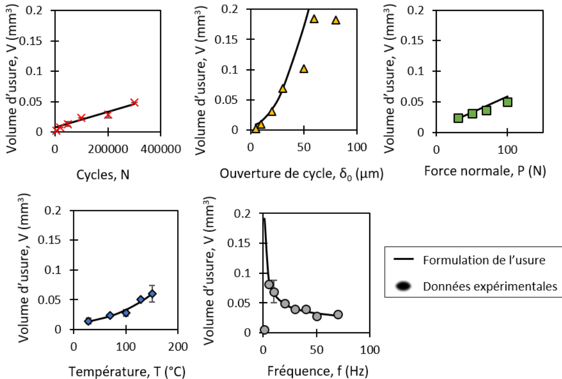
FIGURE 4.11 – Application de la formalisation analytique de l'usure présentée dans l'équation (4.29) à l'étude paramétrique réalisée dans le domaine I ( T < 150^\circ\text{C} ) et présentée en figure 4.1 ( \delta_{0,ref} = \pm 20\mu\text{m} , P_{ref} = 50\text{N} , N_{ref} = 200000 , f_{ref} = 50\text{Hz} , T_{ref} = 100^\circ\text{C} )
