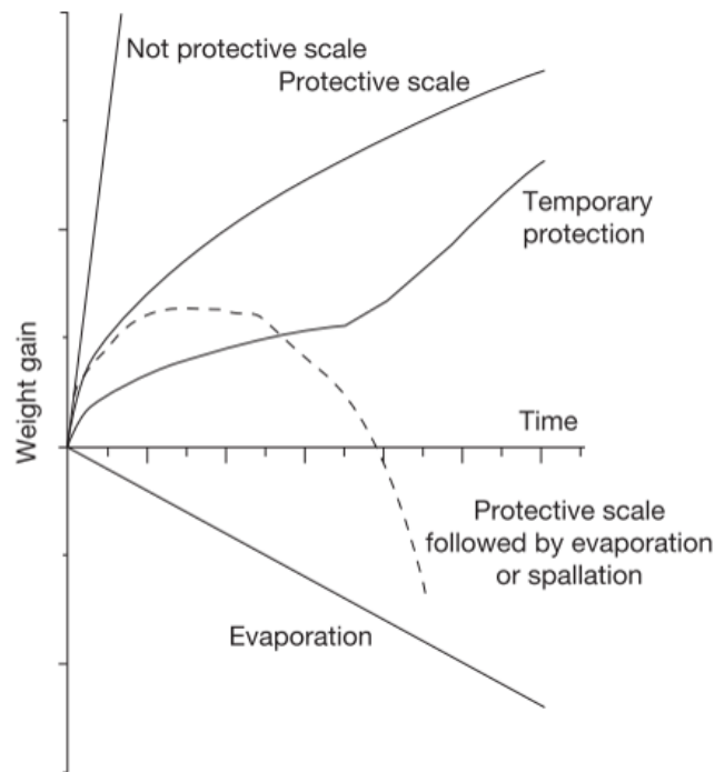
FIGURE 1.21 – Représentation schématique des cinétiques d'oxydation observées à haute température [67]
