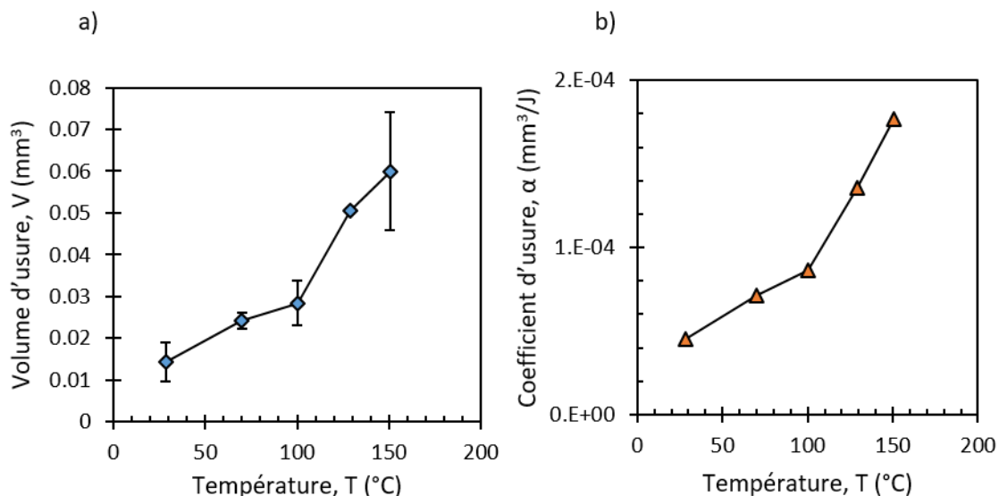
FIGURE 3.10 – Effet de la température sur : a) le volume d'usure ; b) le coefficient énergétique d'usure \alpha ( \delta_0 = \pm 20\mu m , N = 200000 , P = 50N , f = 50Hz )
