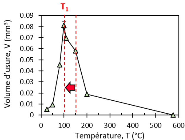
FIGURE 3.28 – Effet de la fréquence sur la transition T_1 : évolution du volume d'usure en fonction de la température à 5 Hz ( \delta_{0,ref} = \pm 20 \mu\text{m} , N_{ref} = 200000 , P_{ref} = 50\text{N} )
