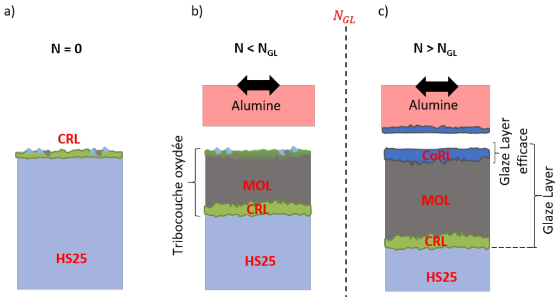
FIGURE 6.21 – Illustration schématique de l'évolution de l'interface sous sollicitation de fretting à 575°C
