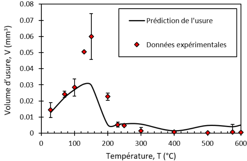
FIGURE 5.5 – Prédiction du volume d'usure en fonction de la température lorsque N_{GL} est formulé selon l'équation (5.7) ( \delta_0 = \pm 20\mu m , N = 200000 , P = 50N , f = 50Hz )
