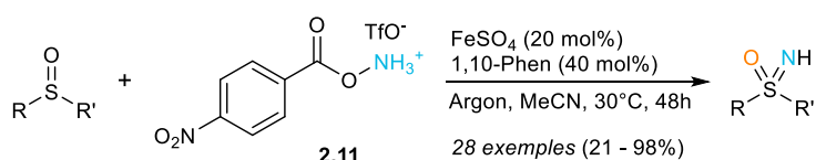
Schéma 2.15: Synthèse monotope de sulfoximines catalysées par le fer
