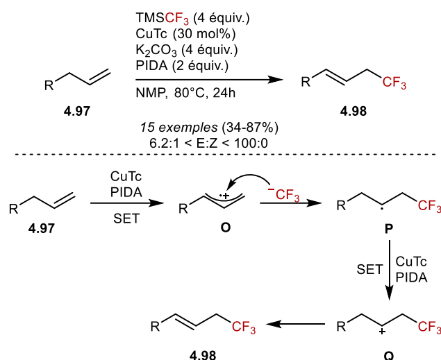
Schéma 4.44 : Trifluorométhylation allylique cupro-catalysée en présence de \text{TMSCF}_3
