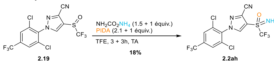
Schéma 2.22 : Synthèse de l'analogue sulfoximine du Fipronil®
