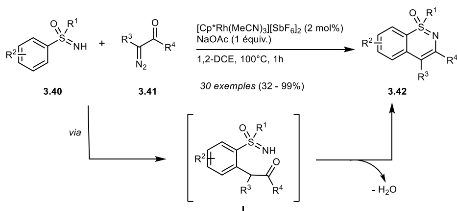
Schéma 3.17 : Synthèse régiosélective de 1,2-benzothiazines par activation de composés diazo
