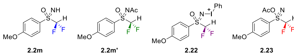
Figure 2.10 : Espèces identifiées au cours de l'étude mécanistique
