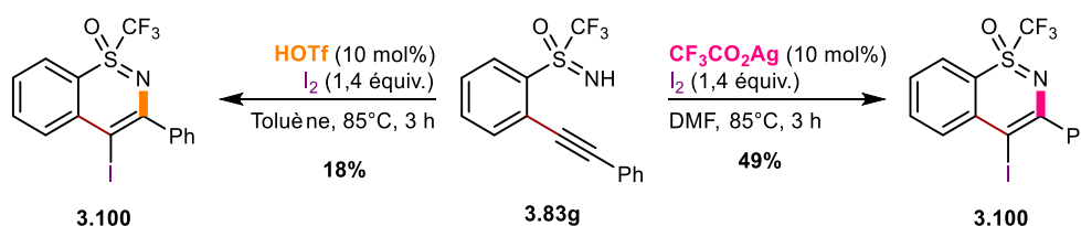
Schéma 3.44 : Iodo-cyclisation de 3.83g en présence d'acide triflique et de diiode
