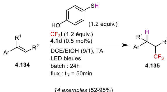
Schéma 4.62 : Hydro-trifluorométhylation en batch et en flux continu
