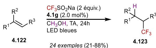
Schéma 4.57 : Hydro-trifluorométhylation d'alcènes non-activés et d'oléfines électro-déficientes
