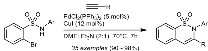
Schéma 3.39 : Synthèse monotopie de benzosultames via un couplage de Sonogashira
