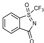
Figure 3.3 : Réactif de trifluorométhylation électrophile dit réactif d'Adachi
