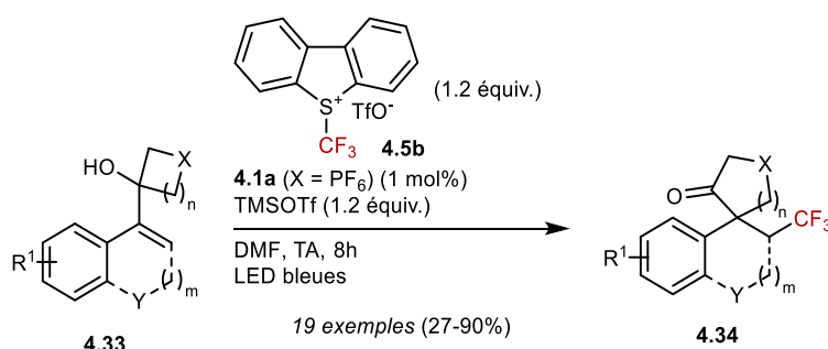
Schéma 4.13 : Trifluorométhylation/expansion de cycle photocatalysée
