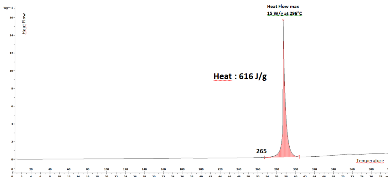
Figure 2.7: Analyse DSC de la sulfoximine N-acétylée 2.2a'
