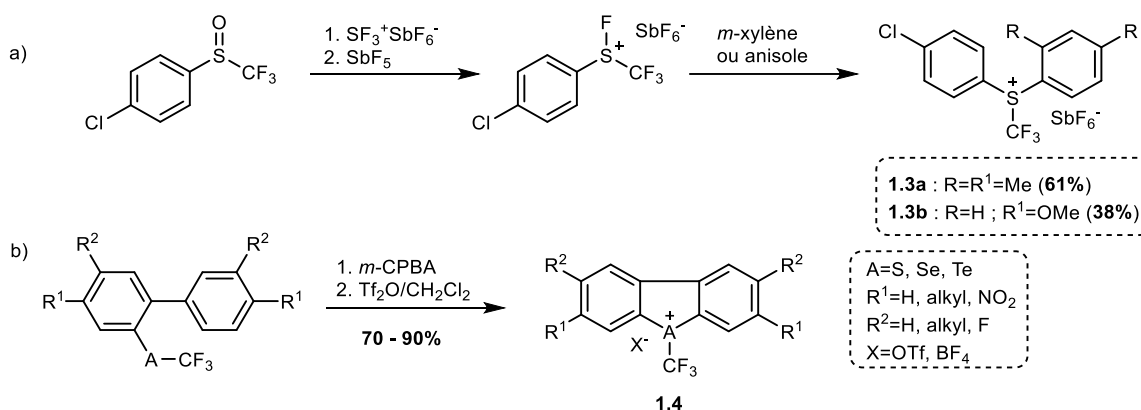
Schéma 1.2 : Synthèse des réactifs de Yagupol'skii et Umemoto
