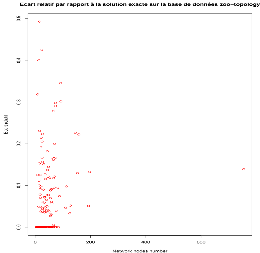
Figure 4.26 – Taille de la population: 50, nombre d’itérations: 100, Taux de mutation: 1%, Pression de sélection: 2
