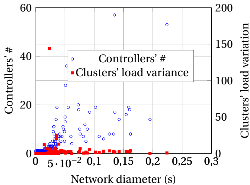
Figure 4.21 – Algorithme K-Hierarchique+ avec \alpha = 0.8 et \beta = 0.9
