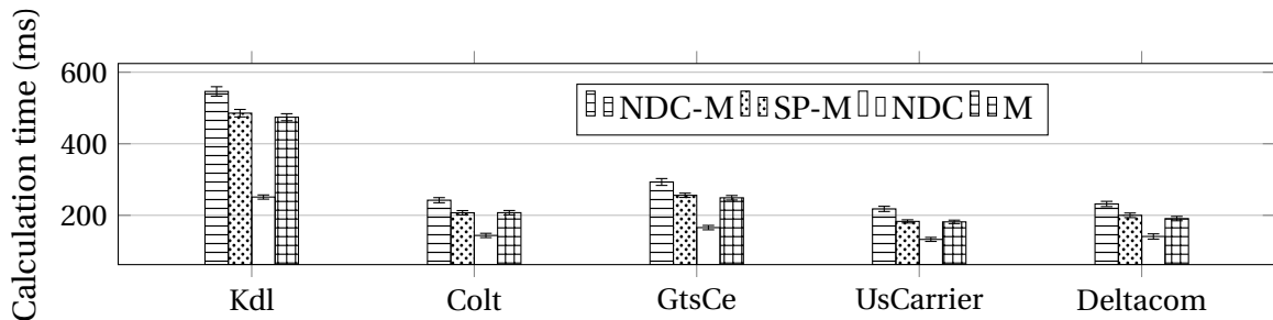
(b) Temps de calcul avec 20 individus et 120 générations
