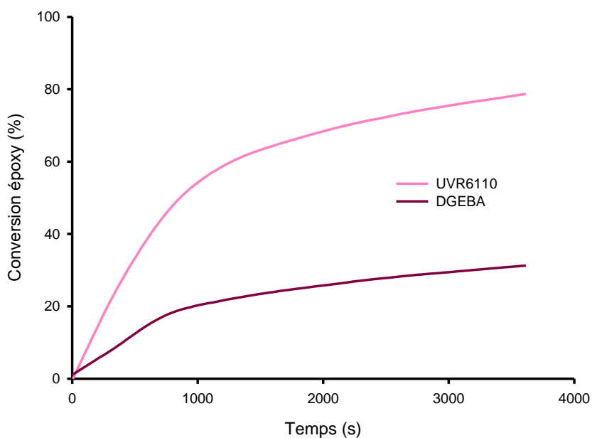
Figure 2 : Évolution des cinétiques de conversion des fonctions époxydes des résines UVR6110® et DGEBA en présence de PGB, T = 60 \text{ }^\circ\text{C} et I_0 = 63 \text{ mW/cm}^2 à 254 nm
