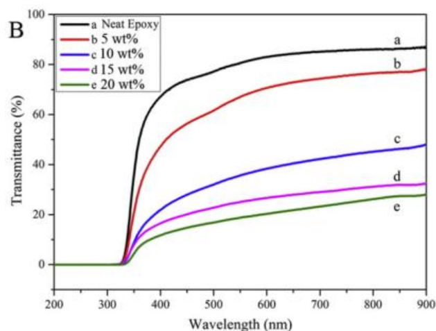
Figure 37 : Spectres de transmittance dans l'UV-visible de films époxydes non chargé (a) et à différents taux de charges (b,c,d,e) 11
