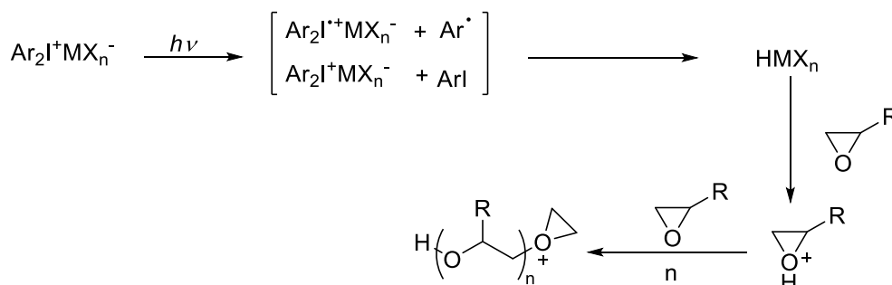
Figure 15 : Schéma réactionnel de la PCROP des époxydes 21
