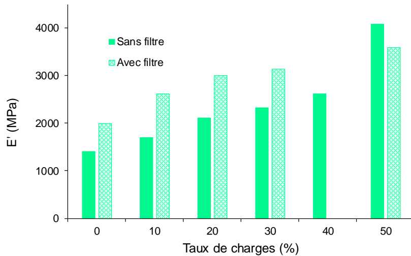
Figure 20 : Modules de conservation à 25 °C des photocomposites à matrice UVR6128® photopolymérisés avec ou sans filtre en fonction du taux de charges B
