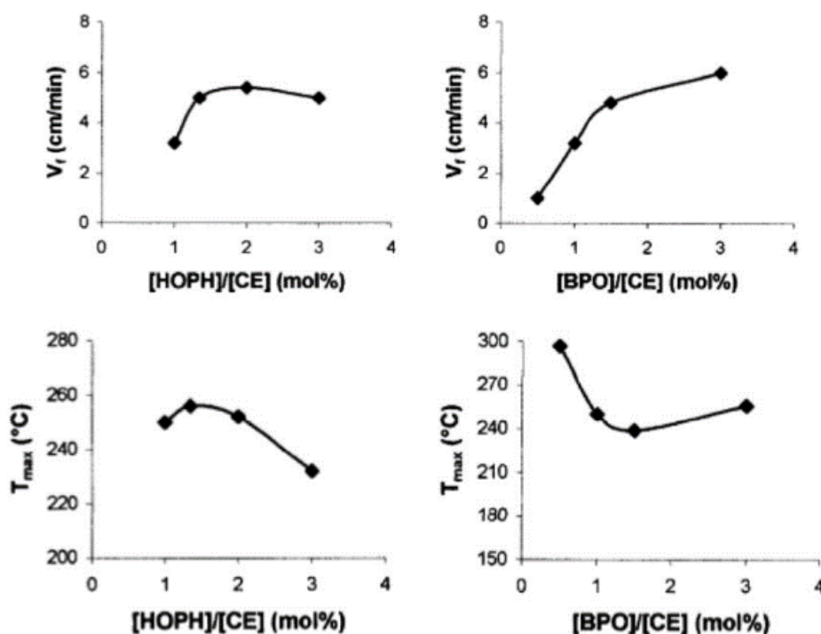
Figure 27 : Impact des ratio [HOPH]/[CE] et [BPO]/[CE] sur la vitesse ( V_r ) et la température maximale ( T_{max} ) du front de polymérisation lors de la RICFP 87
