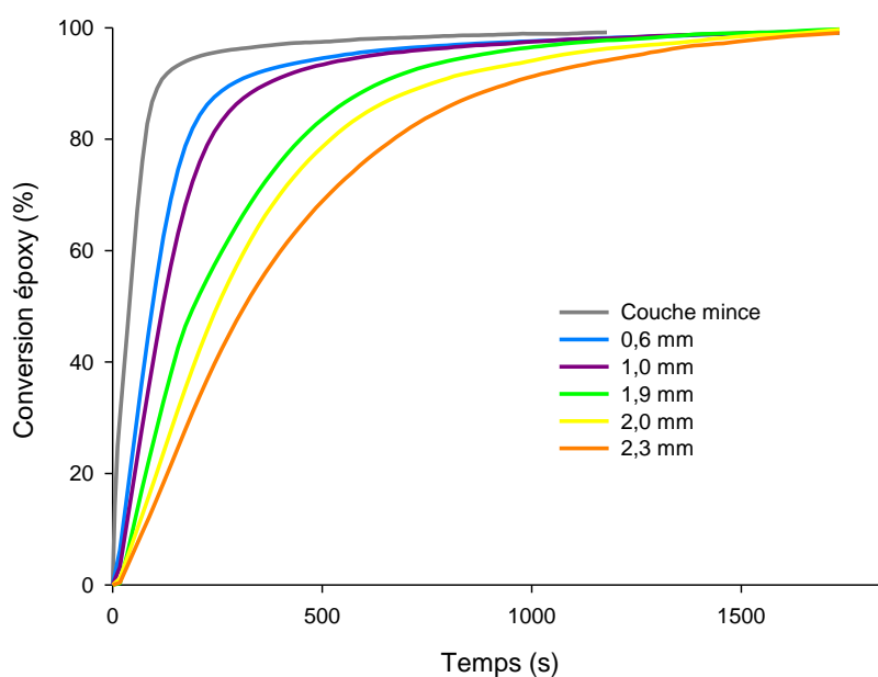
Figure 30 : Cinétiques de conversion en PCROP du TMPGE à différentes épaisseurs à T = 40\text{ °C} et I_0 = 63\text{ mW/cm}^2 à 254\text{ nm}
