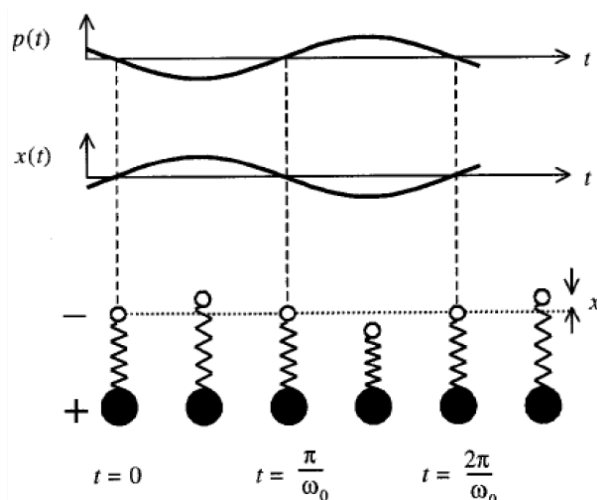
Figure I.9 : principe d'un dipôle oscillant assimilé à un ressort de masse réduite m et se déplaçant selon la direction x [source : cours de spectrométrie _université d'Amiens, master MNSI].
