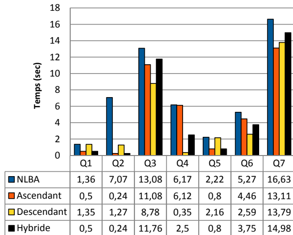
FIGURE 4.5 – Temps d'exécution (20M triplets, implémentation avec Jena TDB Quad Filter )
