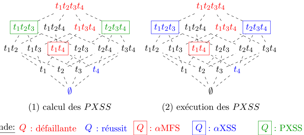
FIGURE 3.3 – Illustration de la découverte des \alpha XSS
