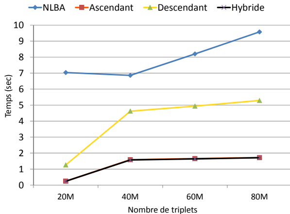
FIGURE 4.7 – Temps d'exécution vs Taille des données (Seuils {0, 2, 0, 4, 0, 6, 0, 8}, implémentation avec Jena TDB Quad Filter)
