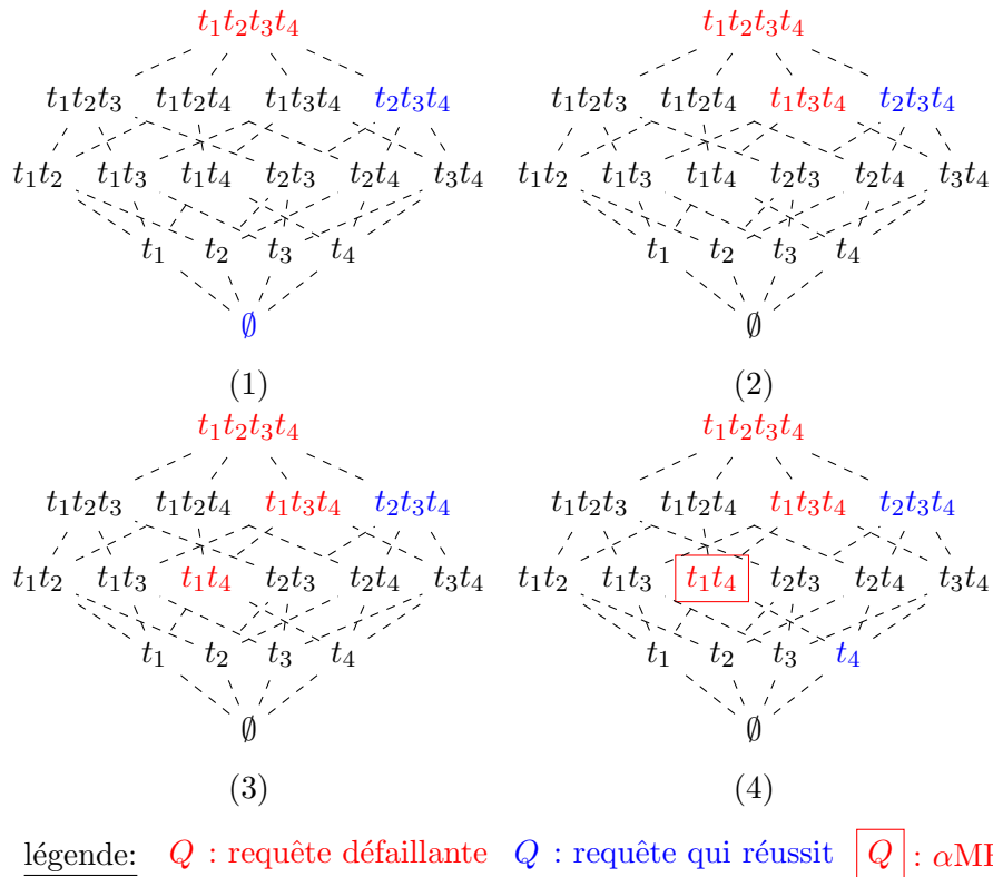
FIGURE 3.2 – Illustration de l'algorithme TrouverUne \alpha MFS
