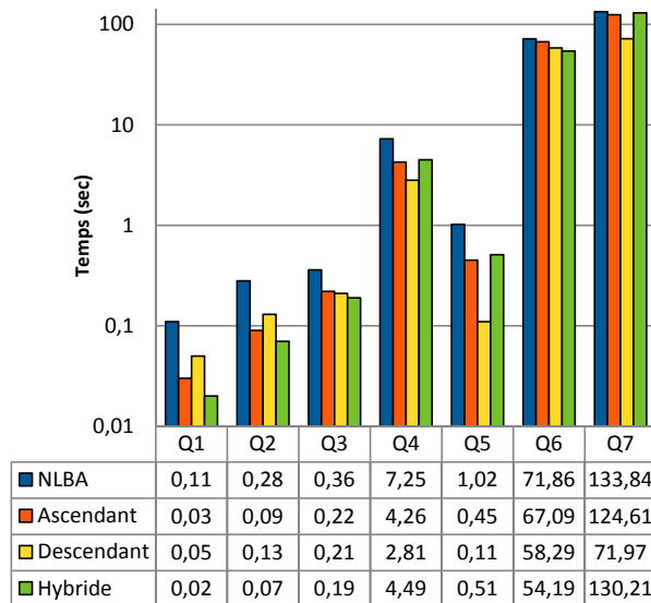
FIGURE 4.13 – Temps d’exécution (20K triplets, Jena TDB, réification)
