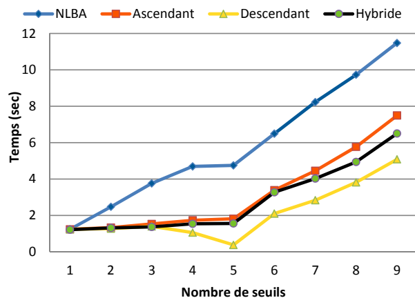
FIGURE 4.8 – Temps d'exécution vs Nombre de seuils \alpha (20M triplets, implémentation avec Jena TDB Quad Filter)
