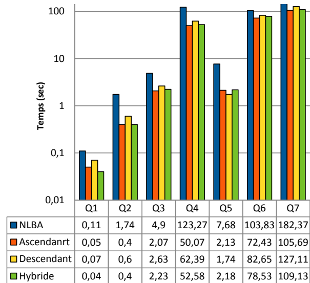
FIGURE 4.14 – Temps d’exécution (20K triplets, Virtuoso, réification)
