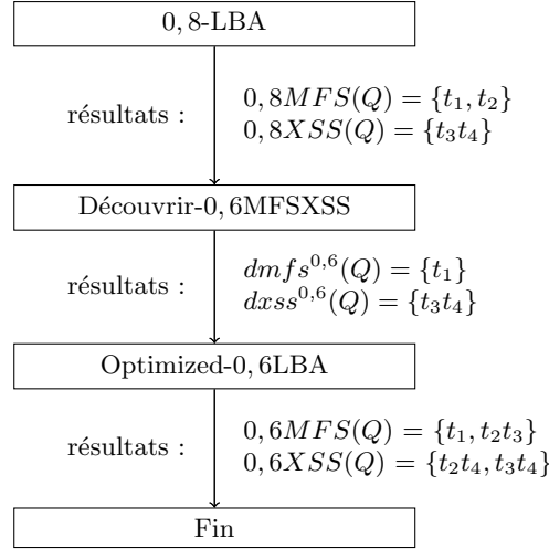
FIGURE 4.3 – Illustration de l’approche descendante pour deux seuils (0,8 et 0,6)
