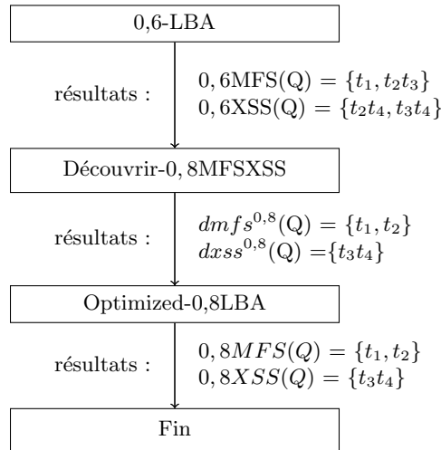
FIGURE 4.2 – Illustration de l'approche ascendante pour deux seuils (0,6 et 0,8)
