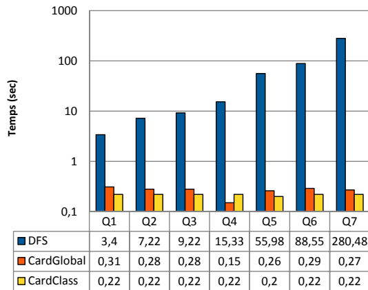
FIGURE 5.11 – Temps d’exécution (32M triplets)
