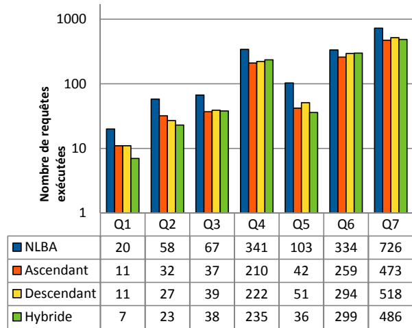
FIGURE 4.12 – # Requêtes exécutées (20K triplets, implémentation avec Jena TDB et Virtuoso, réification )
