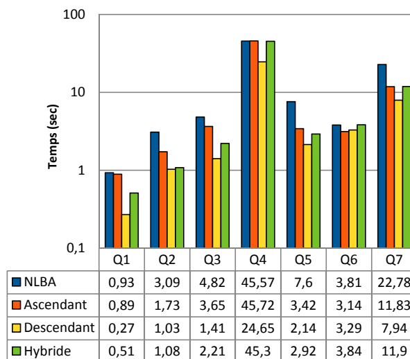
FIGURE 4.10 – Temps d’exécution (100K triplets, implémentation avec Virtuoso Graphes Nommés )
