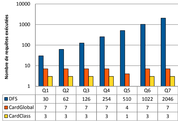
FIGURE 5.12 – # Nombre de requêtes exécutées
