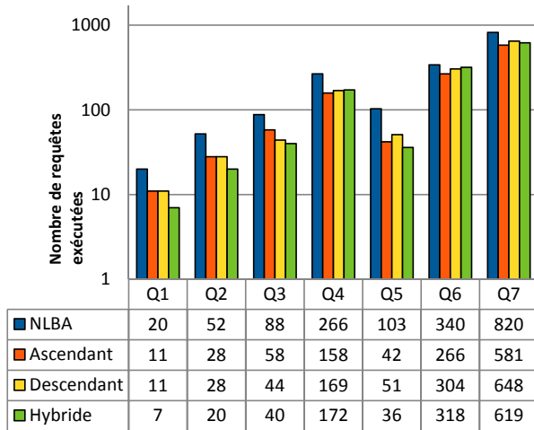
FIGURE 4.11 – Requêtes exécutées (100K Triplets, implémentation avec Jena TDB et Virtuoso, Graphes Nommés )
