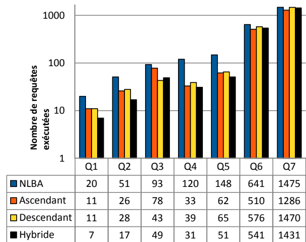
FIGURE 4.6 – # Requêtes exécutées (20M triplets, implémentation avec Jena TDB Quad Filter )
