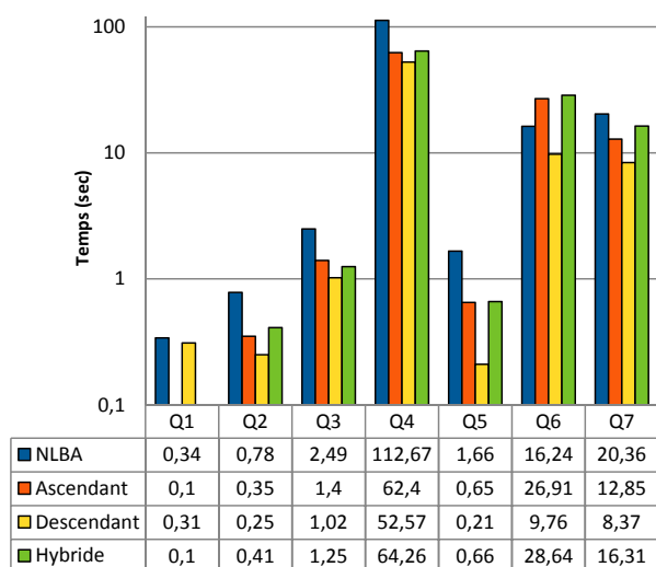
FIGURE 4.9 – Temps d’exécution (100K triplets, implémentation avec Jena TDB Graphes Nommés )
