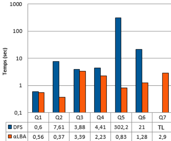
FIGURE 3.5 – Temps d’exécution (20M triplets, implémentation avec Jena TDB Quad Filter )
