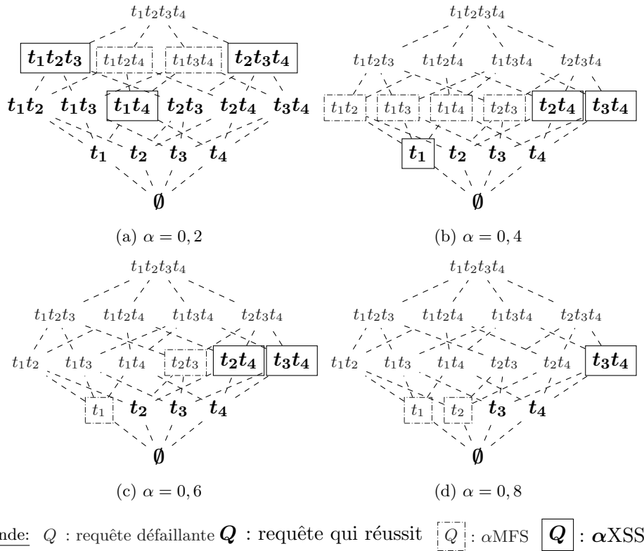
FIGURE 4.1 – Treillis de sous-requêtes de Q pour différents \alpha
