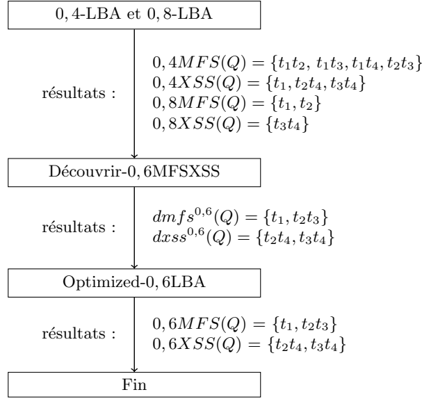
FIGURE 4.4 – Illustration de l’approche hybride pour trois seuils (0,4, 0,8 et 0,6)
