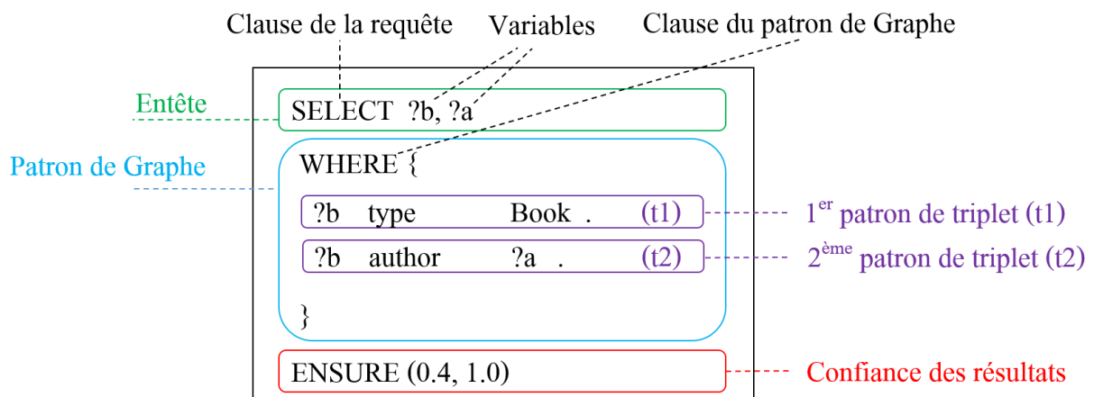
FIGURE 1.10 – Exemple de requête TSPARQL
