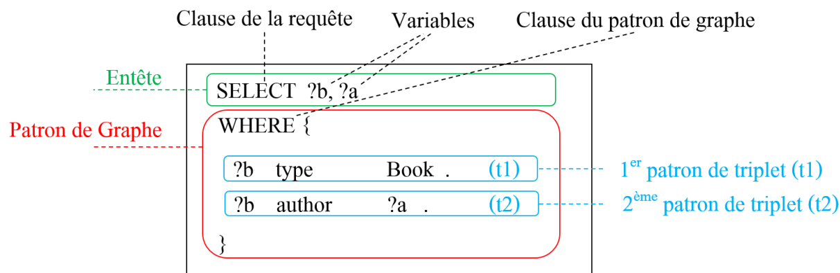
FIGURE 1.6 – Exemple de requête SPARQL
