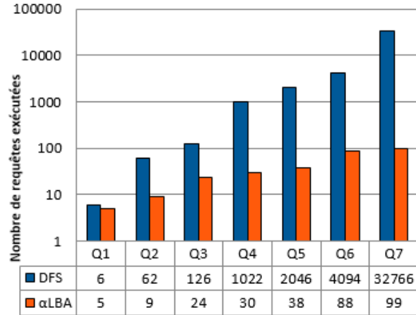
FIGURE 3.6 – # Requêtes exécutées (20M triplets, implémentation avec Jena TDB Quad Filter )
