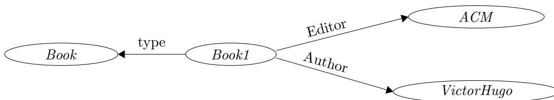
FIGURE 1.3 – Graphe de données RDF
