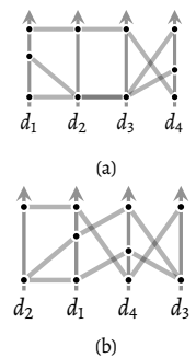
FIGURE 5.3: Les quatre axes ne permettent pas de représenter tous les sous-espaces 2D à la fois. (a) Vue initiale. (b) Vue après déplacement des axes d_1 et d_2 , et d_3 et d_4 .
