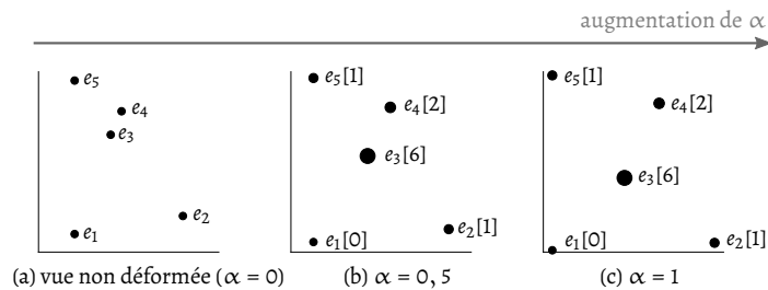
FIGURE 3.16 – Effet de l’augmentation du paramètre d’interpolation \alpha ( doi entre crochets, h = 1/8 , noyau rectangulaire).
