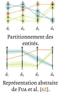
FIGURE 5.21: Agrégation des entités et représentation par rubans polygonaux.
