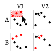
FIGURE 3.1: Broissage (A) et lien (B) sur deux vues liées (V1 et V2). Le lien fonctionne ici par la surbrillance (couleur rouge).
