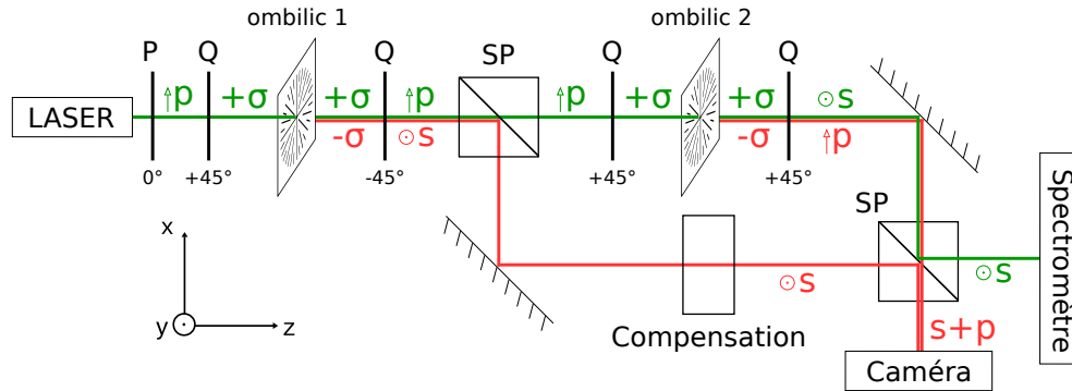
FIGURE 4.10 – Schéma du dispositif expérimental. Les faisceaux représentés en vert correspondent aux composantes non-vortex, ceux en rouge aux composantes vortex. L'état de polarisation est indiqué après chaque élément, les polarisations linéaires sont nommées s et p relativement aux plans d'incidence sur les cubes séparateurs polarisants (SP). Les orientations des lames quart-d'onde ( Q ) sont indiquées relativement à la polarisation ( P ) initiale du faisceau.
