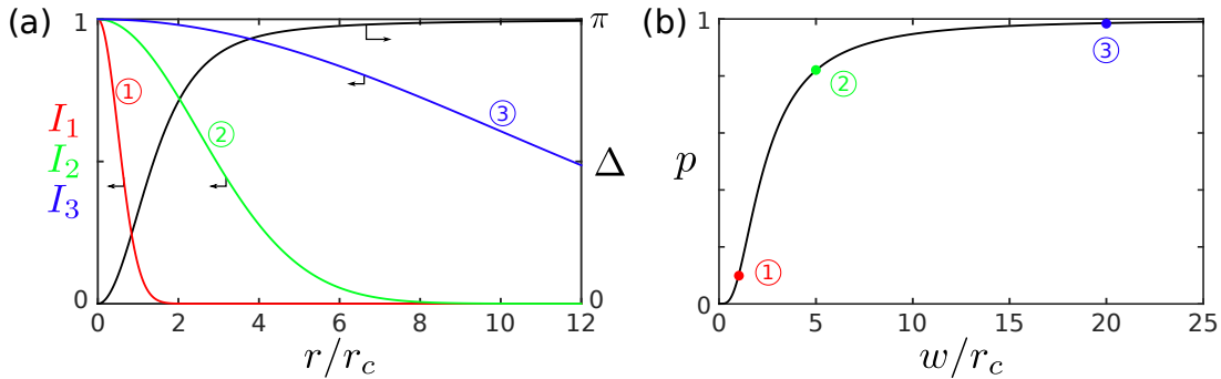
FIGURE 4.5 – Influence du rayon du cœur r_c sur l'efficacité. (a) En noir (ordonnée à droite), représentation du retard \Delta = \pi a^2 , a étant intégré numériquement à partir de l'équation (4.14), en fonction de la distance au centre normalisée, r/r_c , en couleurs (ordonnées à gauche) profils en intensité normalisée de trois exemples de faisceaux gaussiens incidents sur l'ombilic w_1/r_c = 1 , w_2/r_c = 5 et w_3/r_c = 20 . (b) Pureté, calculée selon éq. (4.10) en fonction du rapport w/r_c , les points correspondent aux profils gaussiens illustrés sur (a).
