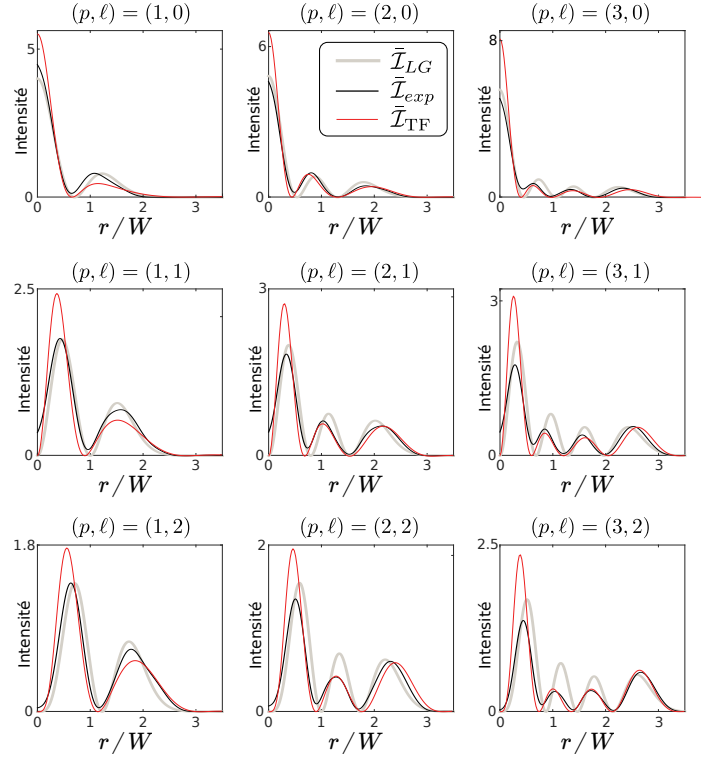
FIGURE 3.13 – Profil radial en intensité normalisée du champ lointain, \bar{I} = I/\sqrt{\int_0^\infty I^2 r dr} pour les modes (p, \ell) \in \{1, 2, 3\} \times \{0, 1, 2\} . Les courbes noires correspondent aux profils expérimentaux, les courbes grises au recouvrement de Laguerre-Gauss optimal et les courbes rouges à la simulation du profil en champ lointain d'un faisceau d'intensité gaussienne de rayon optimal et de phase laguerre-gaussienne en champ proche.
