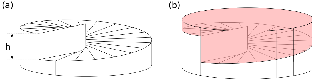
FIGURE 1.14 – (a) Lentille spiralée simple, inspirée de [24] et lentille spiralée achromatique inspirée de [25].
