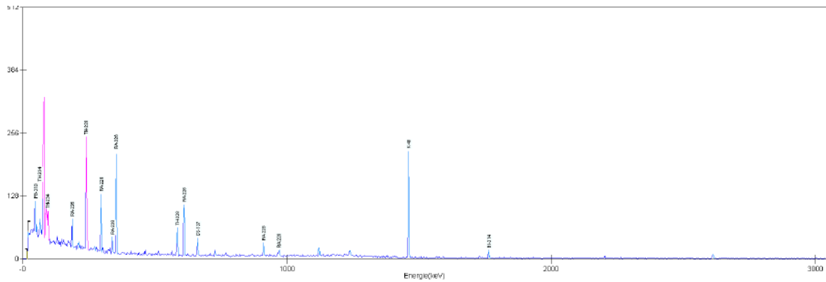
FIGURE 4.10 – Exemple de spectre de 30 à 3000 keV avec des pics de 210 Pb, 234 Th, 226 Ra, 228 Th, 228 Ra, 137 Cs, 40 K, 214 Bi
