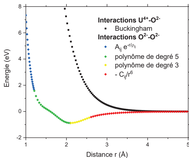
Figure 113 Représentation des interactions interatomiques de faible portée du potentiel de Nicoll des paires d'ions O 2- -O 2- et U 4+ -O 2- en fonction de la distance entre les atomes.
