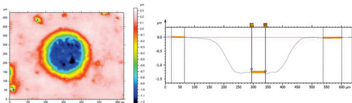
Figure 43 Cartographie d'un cratère SIMS obtenu par interférométrie optique à gauche, où l'échelle de couleur correspond à une échelle en profondeur. A droite, le profil en profondeur correspondant.
