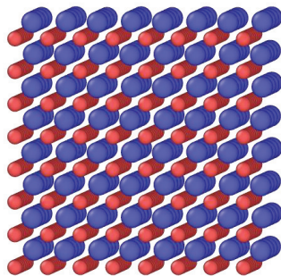
Figure 114 Visualisation de la structure d'UO 2 créée. Il s'agit d'une boîte 4x4x4 contenant 768 atomes. Les atomes d'uranium sont représentés en bleu, et ceux d'oxygène en rouge.
