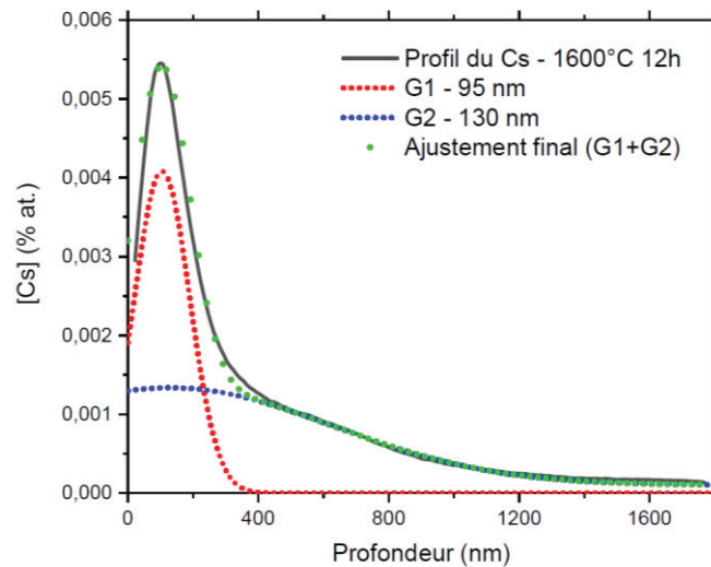
Figure 73 Ajustement du profil de concentration du Cs de l'échantillon implanté à 2 \times 10^{14} Cs/cm 2 et recuit à 1600 °C pendant 12 h. Deux gaussiennes suffisent dans ce cas car il n'y a pas de pic en surface.
