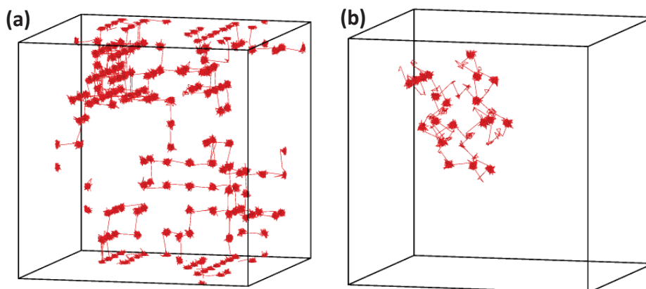
Figure 127 Trajectoire de V_{\text{O}} en (a) et de I_{\text{O}} en (b), à 2300 K.
