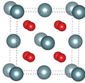
Figure 8 Structure du dioxyde d'uranium. En bleu les atomes d'uranium et en rouge le sous-réseau oxygène.
