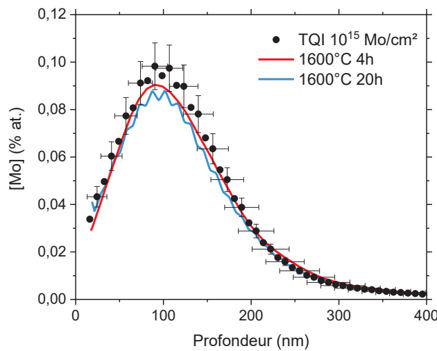
Figure 93 Profils de concentration du Mo après recuit à 1600 °C sous atmosphère réductrice pendant 4 et 20 heures (Sarrasin, 2018).
