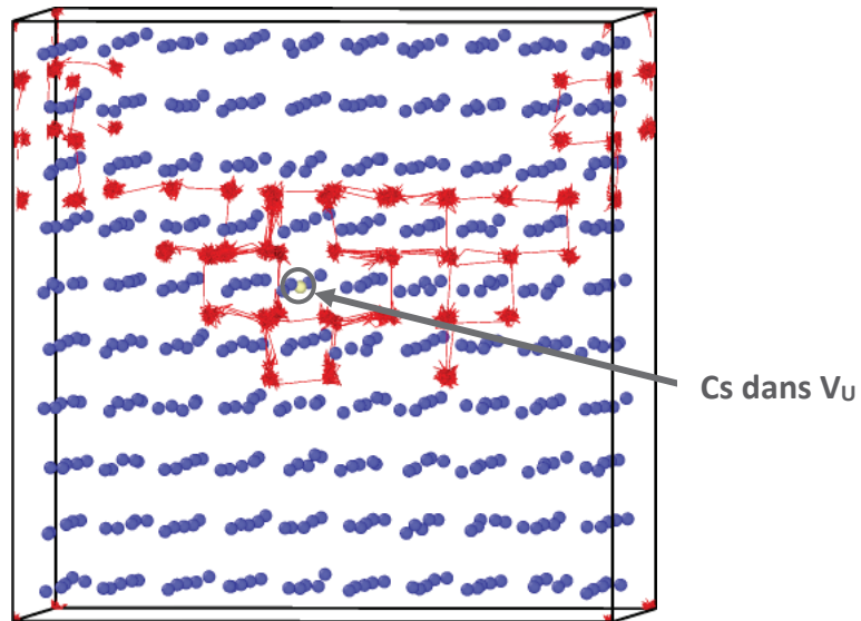
Figure 135 Trajectoires des lacunes d'oxygène (rouge) autour du Cs (en jaune) incorporé dans V_U à 2300 K. Les atomes en bleu représentent les atomes d'uranium et les atomes d'oxygène ne sont pas représentés pour plus de clarté.
