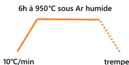
Figure 33 Protocole d'oxydation. Le plateau à 950 °C est atteint après une rampe de montée en température de 10 °C/min.
