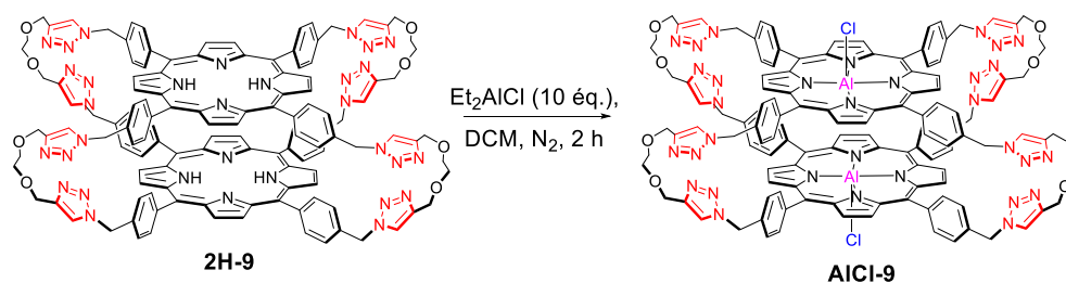
Figure IV-24 : Synthèse de la cage \text{Al}(\text{Cl}) -9.
