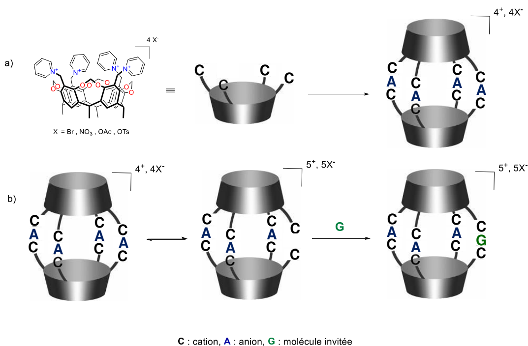
Figure I-11 : a) Formation d'une capsule auto-assemblée par interactions entre trois ions à partir d'un cavitant pyridinium ; b) Equilibre entre la capsule et une hémicapsule et formation d'un complexe hémicapsule-molécule invitée. 62
