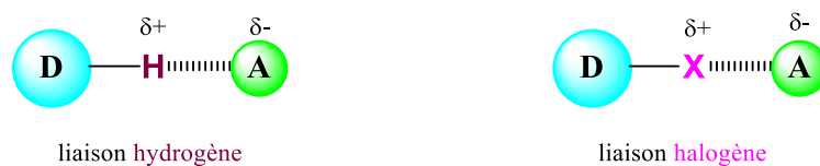
Figure I-12 : Analogie entre la liaison hydrogène et la liaison halogène. 63
