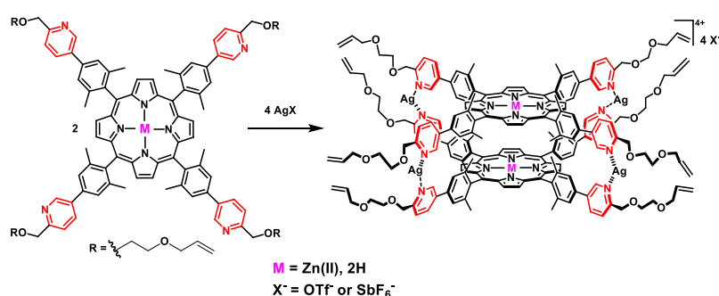
Figure I-31 : Cage de coordination bis-porphyrinique obtenue par coordination des ions argent(I) sur des ligands pyridine périphériques. 87
