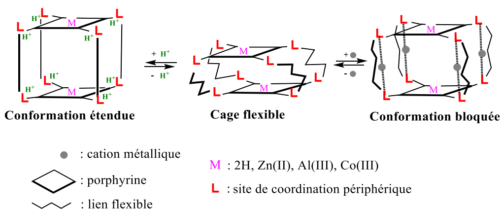
Figure III-1 : Principe des commutateurs moléculaires développés dans cette thèse.
