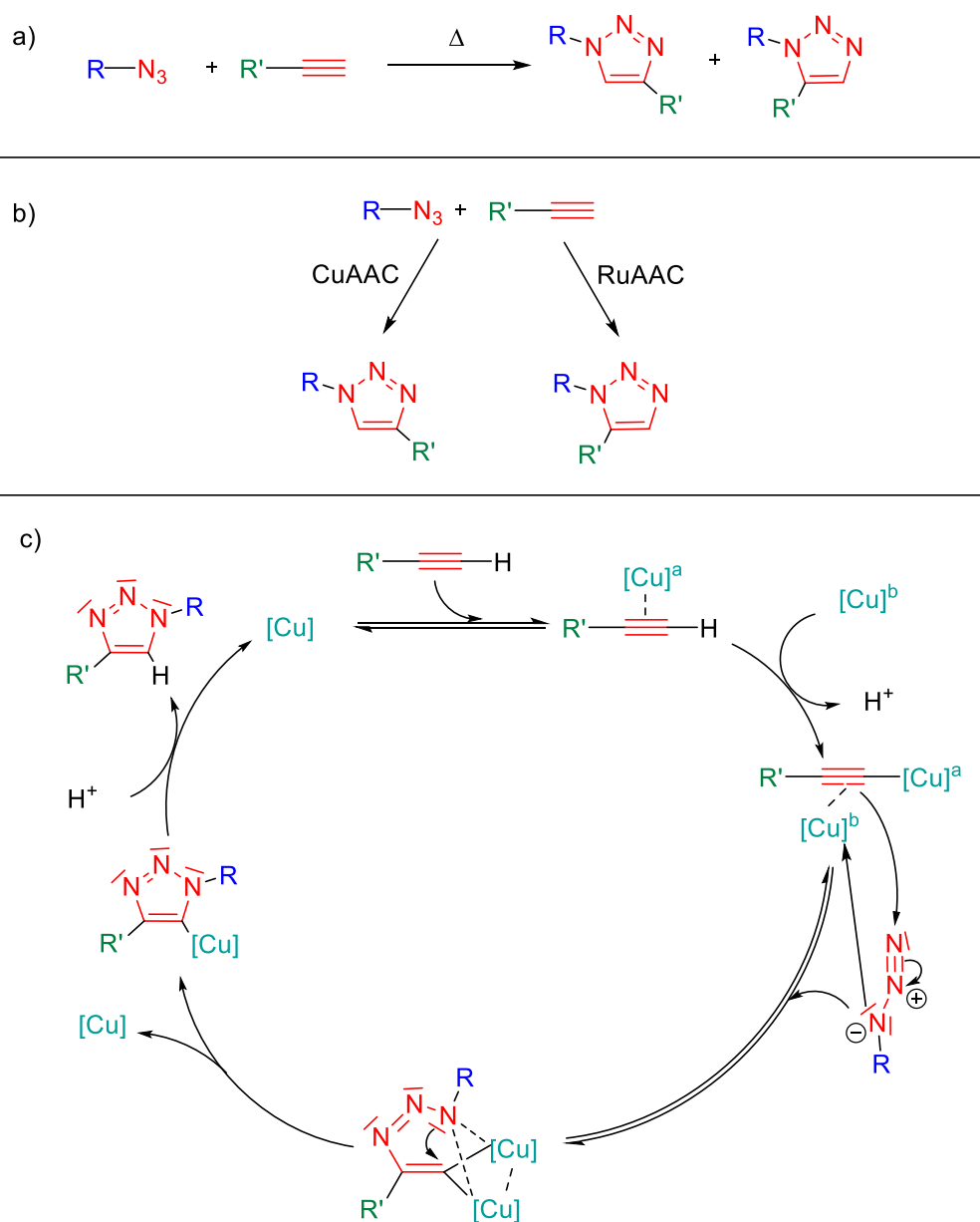
Figure II-3 : Cycloaddition 1,3-dipolaire entre un alcyne et un azoture a) non catalysée 91,92 ; b) catalysée et produisant sélectivement le 1,4- 93,94 et le 1,5-triazole 95 ; c) Mécanisme bimétallique pour la CuAAC proposé par Fokin en 2013. 96
