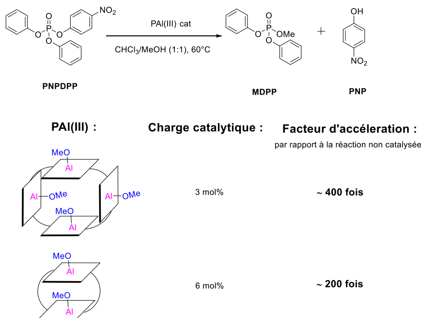
Figure IV-17: Méthanolysé du PNPDPDP catalysée par des macrocycles bis- et tétraporphyriniques incorporant des porphyrines d'aluminium(III) décrite par le groupe de Hupp. 115,116
