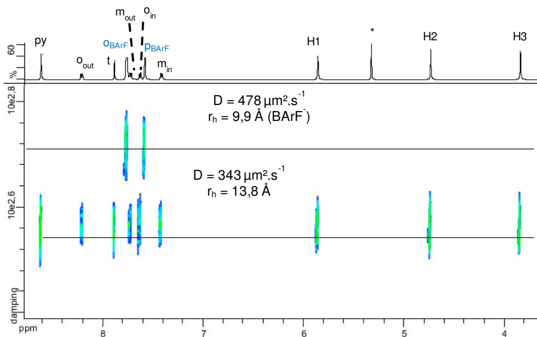
Figure III-16 : Spectre RMN DOSY ( \text{CD}_2\text{Cl}_2 , 600 MHz, 298 K) du complexe [\text{Ag}_4\cdot(\text{Zn-9})](\text{BArF})_4 , * solvants résiduels.
