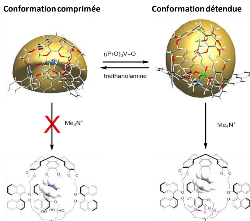
Figure I-22 : Cage covalente à taille de cavité variable sous l'action d'un stimulus chimique. 73
