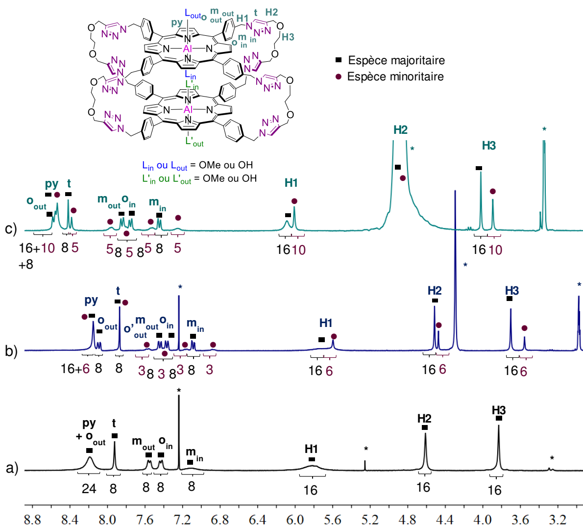
Figure IV-5: Spectres RMN ^1\text{H} (300 MHz, 298K) de la cage Al(OMe)-9 dans a) \text{CDCl}_3 + 5\% \text{CD}_3\text{OD} ; b) \text{CDCl}_3/\text{CD}_3\text{OD} (1:1) ; c) \text{CD}_3\text{OD} , * solvants résiduels.
