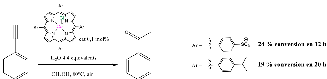
Figure V-21 : Hydratation du phénylacétylène en acétophénone. 175,176
