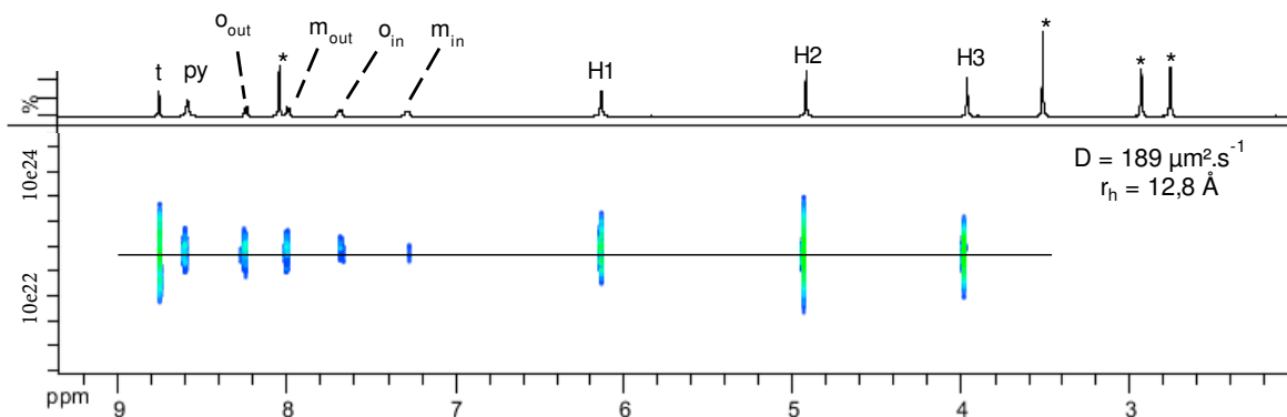
Figure III-5 : Spectre RMN DOSY ( \text{DMF-}d_7 , 600 MHz, 298 K) du complexe [\text{Ag}_4 \cdot (\text{2H-9})](\text{OTf})_4 , * solvants résiduels.
