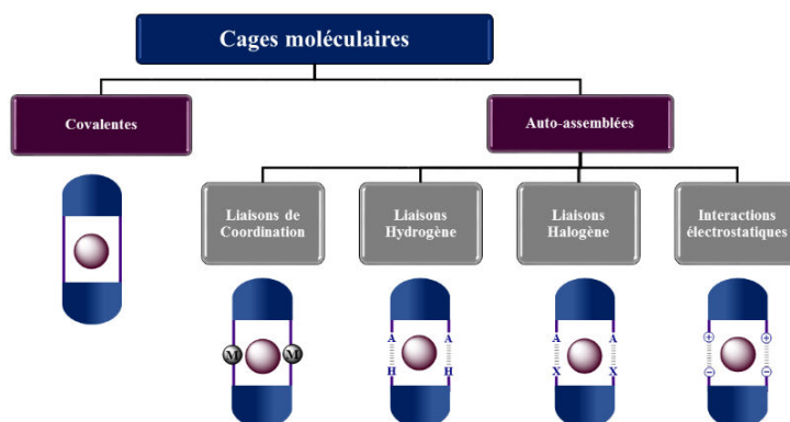
Figure I-7 : Capsules moléculaires covalentes ou auto-assemblées de diverses manières, incorporant une molécule invitée.
