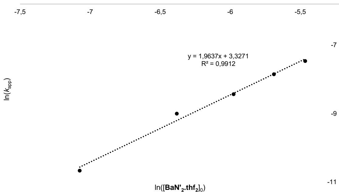
Figure 2.28. Tracé logarithmique de la constante de vitesse apparente ( k_{app} ) en fonction de la concentration initiale en pré-catalyseur pour le couplage déshydrogénant de HOB{CH(SiMe 3 ) 2 } 2 ( A ) et PhSiH 3 catalysé [Ba{N(SiMe 3 ) 2 } 2 .thf 2 ]. Conditions: {(Me 3 Si) 2 CH} 2 BOH (36 mg, 0.102 mmol), PhSiH 3 (13 \mu L, 0.102 mmol), [BaN' 2 .thf 2 ] = 8.47·10 -4 M, 1.69·10 -3 M, 2.54·10 -3 M, 3.39·10 -3 M et 4.23·10 -3 M, T = 333 K, solvant C 6 D 6 (0.6 mL).
