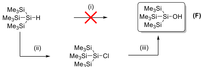
Schéma 3.1. Synthèse du silanol F . Conditions réactionnelles: (i) m-CPBA, thf, -30\text{ }^\circ\text{C} , 2 h; (ii) \text{CCl}_4 , \text{CHCl}_3 , reflux, 12 h, 98 %; (iii) éther de pétrole, \text{NEt}_3 , \text{H}_2\text{O} , 25\text{ }^\circ\text{C} , 24 h, 94 %.
