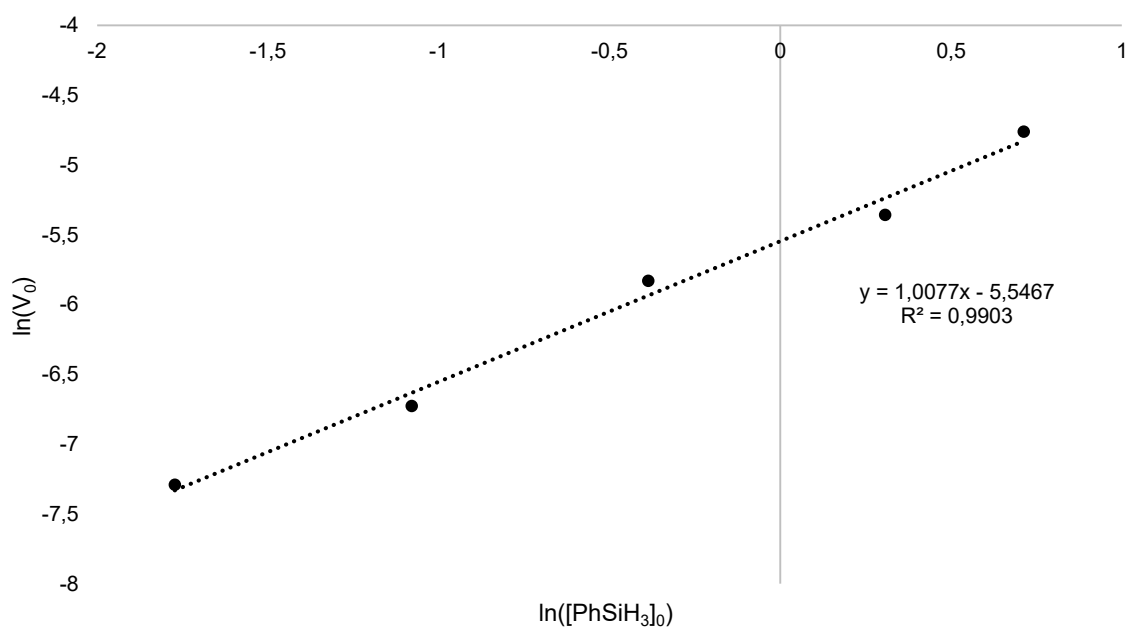
Figure 2.26. Tracé de \ln(V_0) = x\ln([PhSiH_3]_0) pour le couplage déshydrogénant de HOB\{CH(SiMe_3)_2\}_2 (A) et PhSiH_3 catalysé [Ba\{N(SiMe_3)_2\}_2.thf_2] ( BaN'2.thf2 ), montrant un ordre cinétique partiel de un pour la concentration en silane. Conditions: \{(Me_3Si)_2CH\}_2BOH (36 mg, 0.102 mmol), [BaN'2.thf_2] = 3.39 \cdot 10^{-3} M, [PhSiH_3] = 1.70 \cdot 10^{-1} M, 3.40 \cdot 10^{-1} M, 6.80 \cdot 10^{-1} M, 1.36 M et 2.04 M, T = 333 K, solvant C_6D_6 (0.6 mL).
