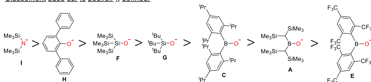
Figure 4.21. Classement des différents ligands étudiés selon leur pouvoir \sigma donneur, leur pouvoir \pi .
