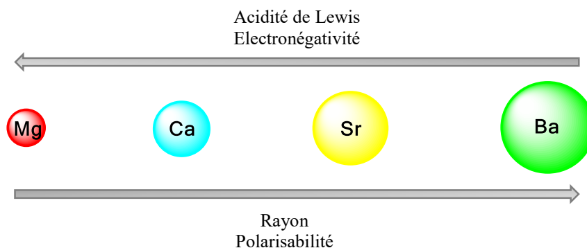
Figure 1.1. Différence entre les propriétés des métaux alcalino-terreux.
