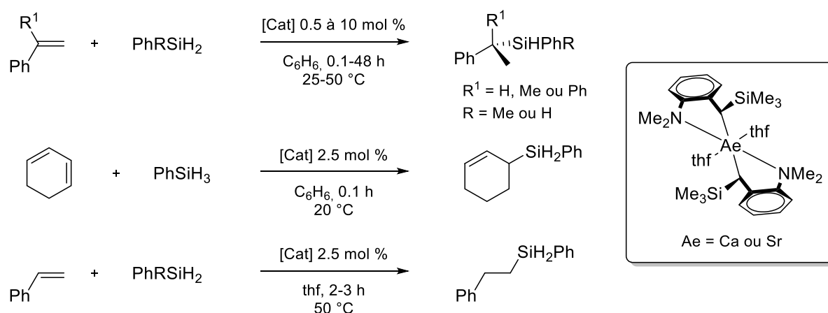
Figure 1.14. Réactions d'hydrosilylation sélectives d'alcènes.
