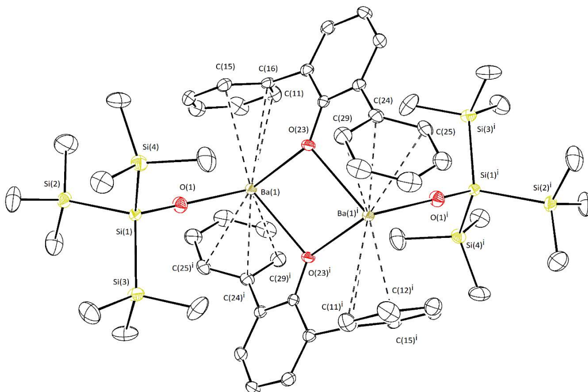
Figure 4.13. Représentation moléculaire ORTEP du complexe [\text{Ba}\{\mu_2\text{-O}(2,6\text{-Ph-C}_6\text{H}_3)\}\{\text{OSi}(\text{SiMe}_3)_3\}]_2 ( 15 ) à l'état solide. Niveau de probabilité des ellipsoïdes à 50%. Les hydrogènes CH ont été éliminés pour plus de clarté. Distance (Å) et angles (°) sélectionnés : Ba1-O1 = 2.356(1), Ba1-O23 = 2.715(1), Ba1 i -O23 = 2.673(1), Si1-O1 = 1.620(2), Ba1-C11 = 3.348(2), Ba1-C15 = 3.199(2), Ba1-C16 = 3.203(2), Ba1-C24 i = 3.120(2), Ba1-C25 i = 3.252(2), Ba1-C29 i = 3.273(2), O1-Ba1-O23 i = 107.11(5), O1-Ba1-O23 = 111.75(5), O23-Ba1-O23 i = 78.87(4), Ba1-O1-Si1 = 166.69(9).
