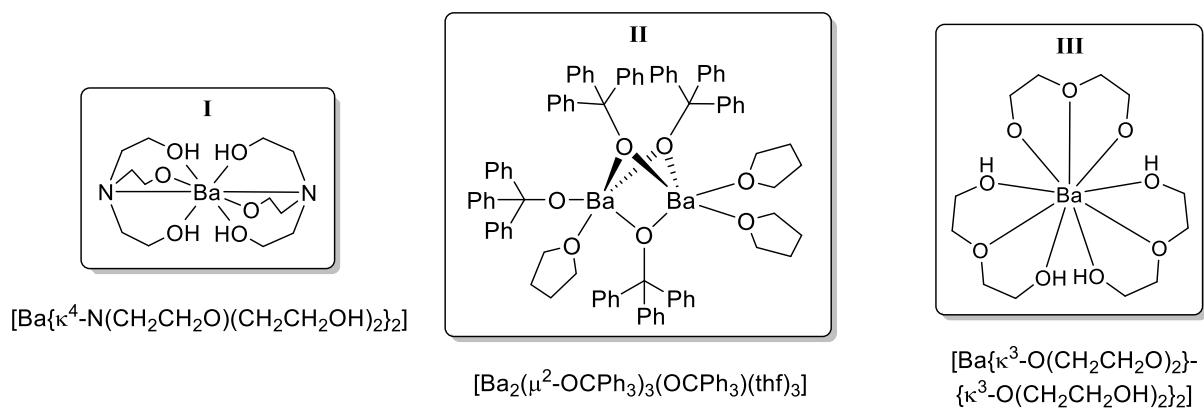
Figure 4.1. Exemple de complexes moléculaires baryum-alcoolates solubles. [3-5]
