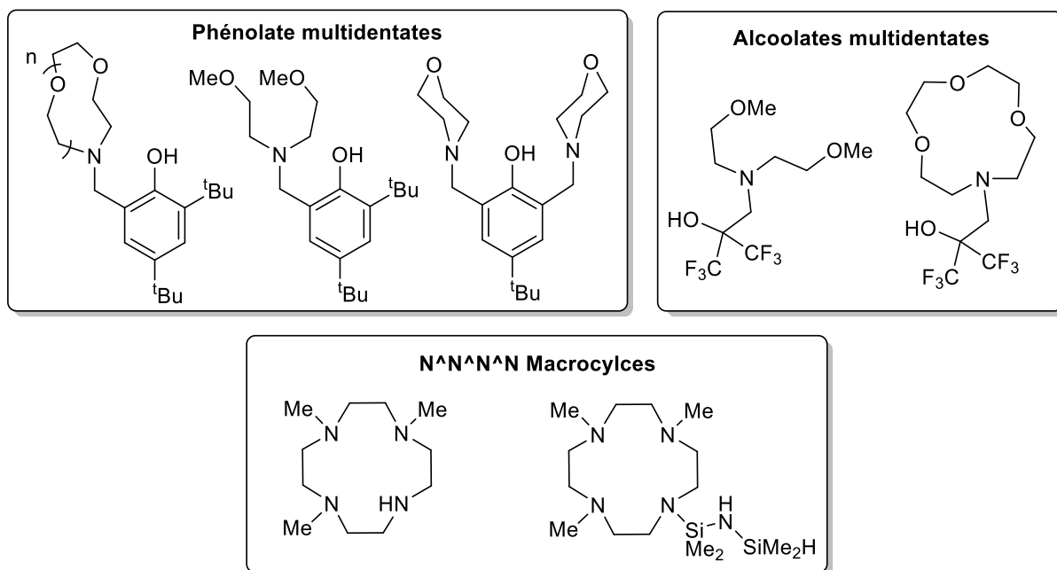
Figure 1.6. Ligands multidentates utilisés pour la stabilisation des complexes hétéroleptiques d'alcalino-terreux.
