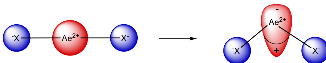
Figure 2.9. Effet de la polarisation des métaux alcalino-terreux sur l'angle X-Ae-X permettant une interaction favorable entre les ligands anioniques et la partie positive du dipôle.
