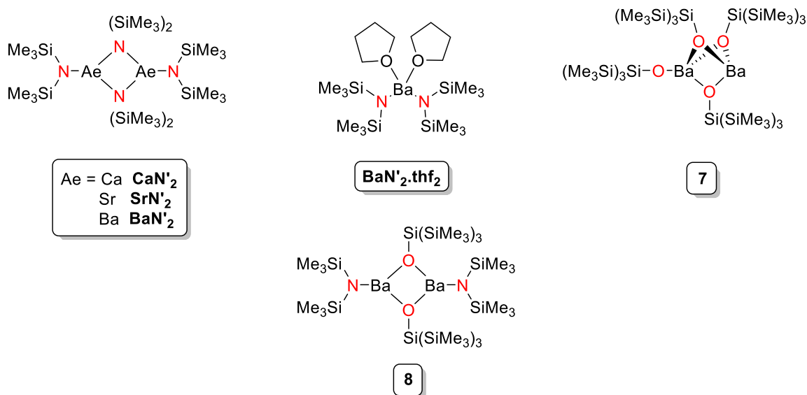
Figure 3.13. Complexes d'alcalino-terreux utilisés comme précatalyseurs pour le couplage déshydrogénant SiO–H/H–Si.
