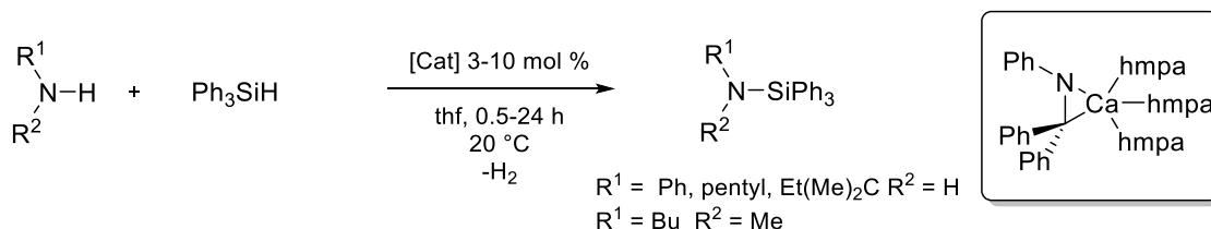
Figure 1.20. Réactions de couplage déshydrogérant catalysé par [\text{Ca}(\text{hmpa})_3(\eta^2\text{-Ph}_2\text{CNPh})] . [90]
