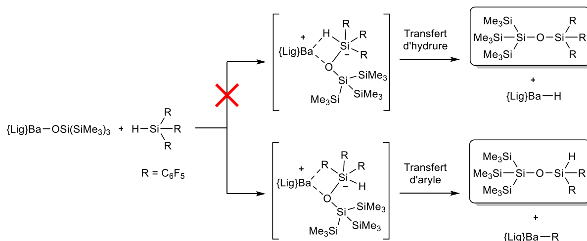
Figure 3.23. Hypothèse sur la réactivité de \text{HSi}(\text{C}_6\text{F}_5)_3 dans les réactions de couplage déshydrogénéant.
