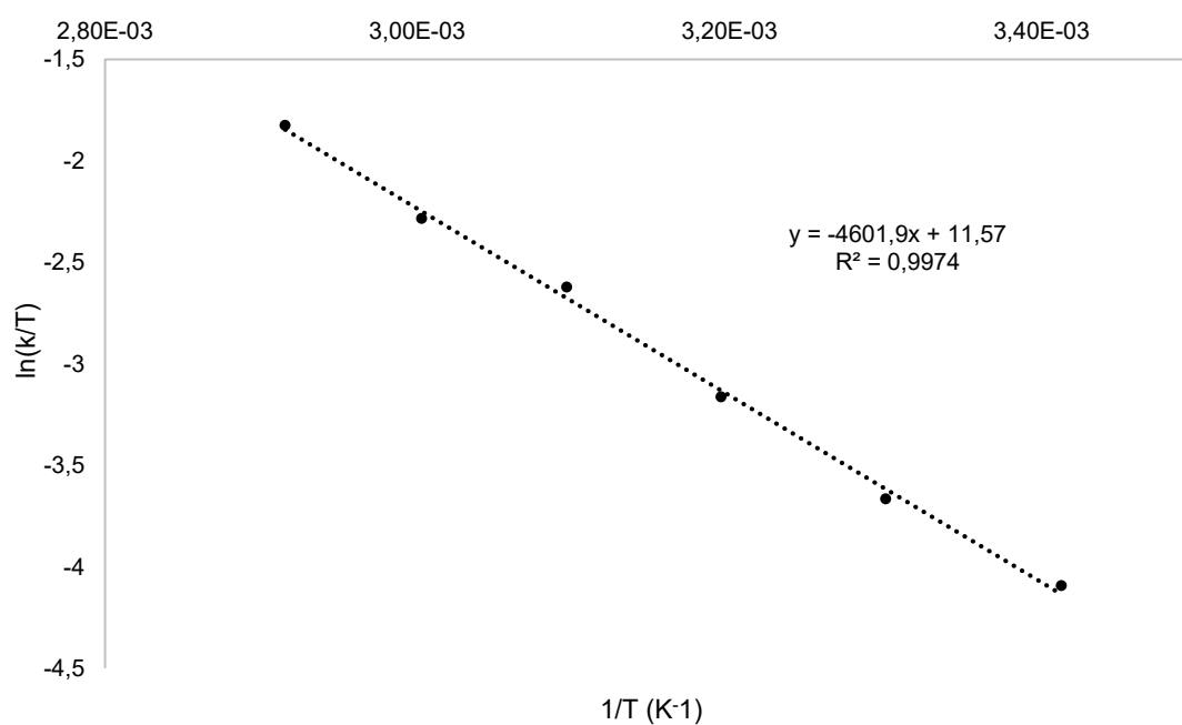
Figure 2.32. Graphique d'Eyring pour le couplage déshydrogénant de \text{HOB}\{\text{CH}(\text{SiMe}_3)_2\}_2 (A) et \text{PhSiH}_3 catalysé [\text{BaN}'_2.\text{thf}_2] . Conditions: \{(\text{Me}_3\text{Si})_2\text{CH}\}_2\text{BOH} (36 mg, 0.102 mmol), \text{PhSiH}_3 (13 \mu\text{L} , 0.102 mmol), [\text{BaN}'_2.\text{thf}_2] = 3.39 \cdot 10^{-3} M, T = 293 à 343 K, solvant \text{C}_6\text{D}_6 (0.6 mL).
