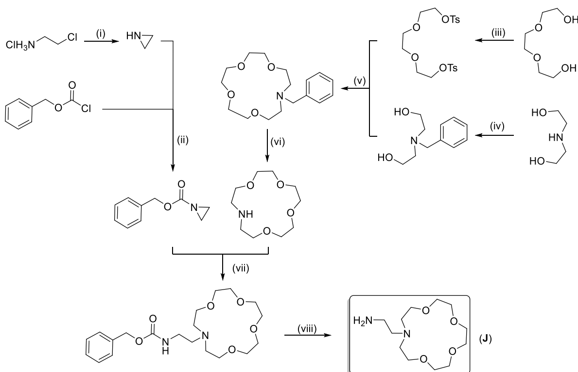
Schéma 5.1. Synthèse du fragment 2-(1-aza-15-crown-5)-ethan-1-amine ( J ). Conditions réactionnelles: (i) NaOH, H 2 O, 50 °C, 4 h, 75%; (ii) Et 2 O, NEt 3 , 0 to 20 °C, 12 h, 51%; (iii) TsCl, DMAP, NEt 3 , CH 2 Cl 2 , 0 to 20 °C, 12 h, 85%; (iv) BnBr, Na 2 CO 3 , acétone, reflux, 4 h, 80%; (v) NaOH, n Bu 4 NBr, toluène, 70 °C, 10 h, 82%; (vi) H 2 , Pd/C, MeOH, 20 °C, 12 h, 80%; (vii) CH 3 CN/toluène (1:1 v/v), reflux, 24 h, 70%; (viii) H 2 , Pd/C, MeOH, 20 °C, 15 h, 97%.
