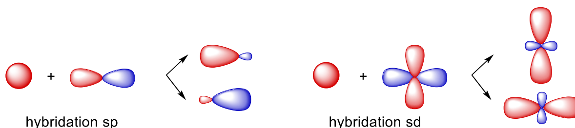
Figure 2.10. Représentation des orbitales hybridées sp et sd.
