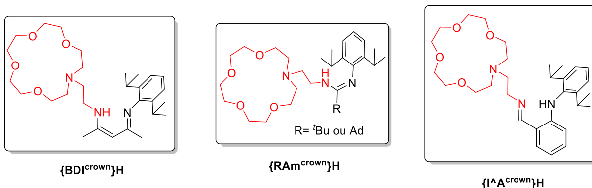
Figure 5.4. Proligands cibles comprenant un fragment encombrant (noir) et un fragment multidentate polyoxygéné (rouge).
