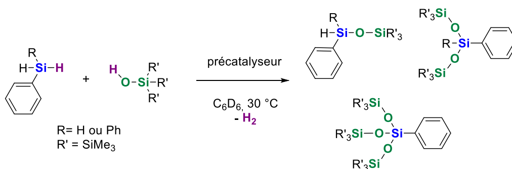
Schéma 3.5. Réaction modèle pour l'étude du couplage déshydrogénant SiO–H/H–Si.
