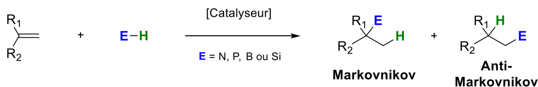
Figure 1.10. Réactions d'hydroélémentation intermoléculaire d'oléfines.
