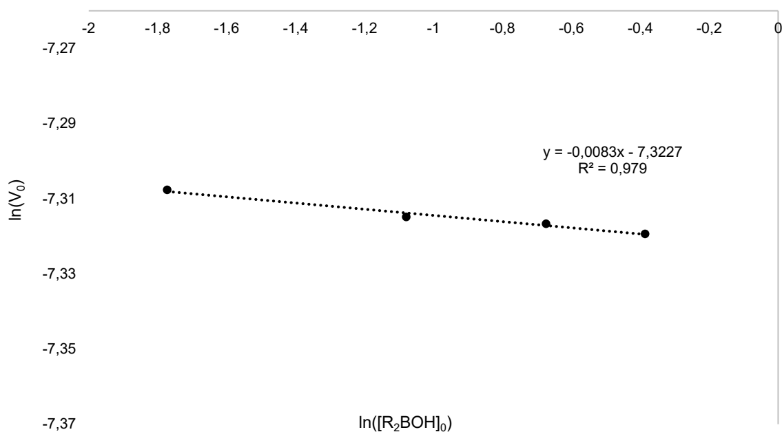
Figure 2.25. Tracé de \ln(V_0) = x\ln([R_2BOH]_0) pour le couplage déshydrogénant de de HOB\{CH(SiMe_3)_2\}_2 (A) et PhSiH_3 catalysé [Ba\{N(SiMe_3)_2\}_2.thf_2] ( BaN'2.thf2 ), montrant un ordre cinétique partiel de zéro pour la concentration en acide borinique. Conditions: PhSiH_3 (13 \mu L, 0.102 mmol), [BaN'2.thf_2] = 3.39 \cdot 10^{-3} M, [(Me_3Si)_2CH]_2BOH = 1.70 \cdot 10^{-1} M, 3.40 \cdot 10^{-1} M, 5.10 \cdot 10^{-1} M and 6.80 \cdot 10^{-1} M, T = 333 K, solvant C_6D_6 (0.6 mL).
