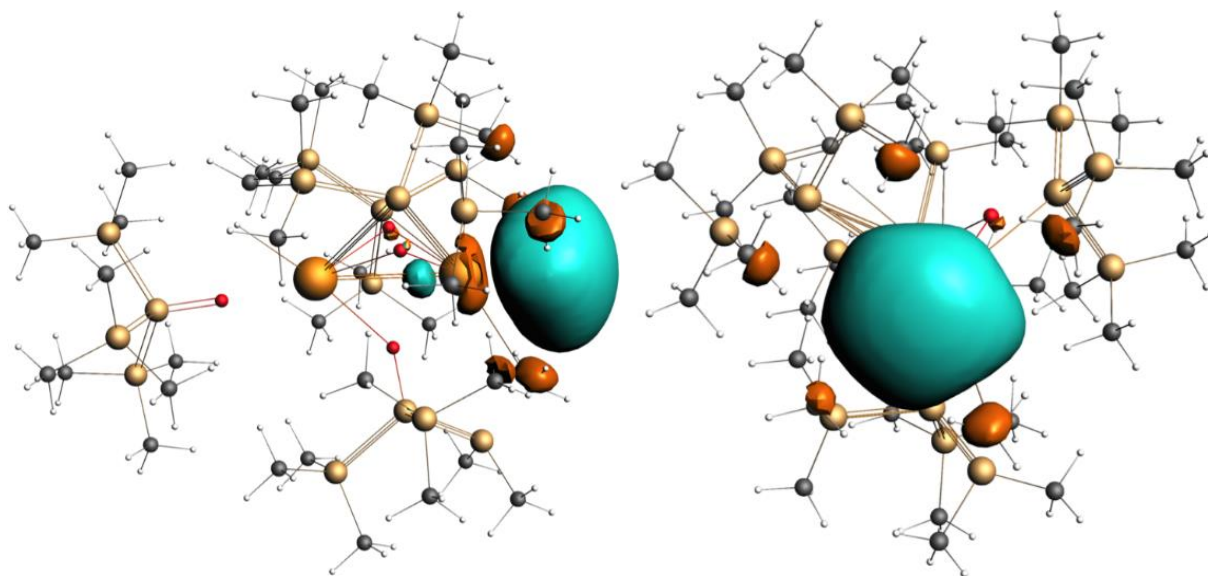
Figure 3.6. Représentation de la LUMO du complexe [\text{Ba}_2\{\mu_2\text{-OSi}(\text{SiMe}_3)_3\}_3\{\text{OSi}(\text{SiMe}_3)_3\}] ( 7 ).
