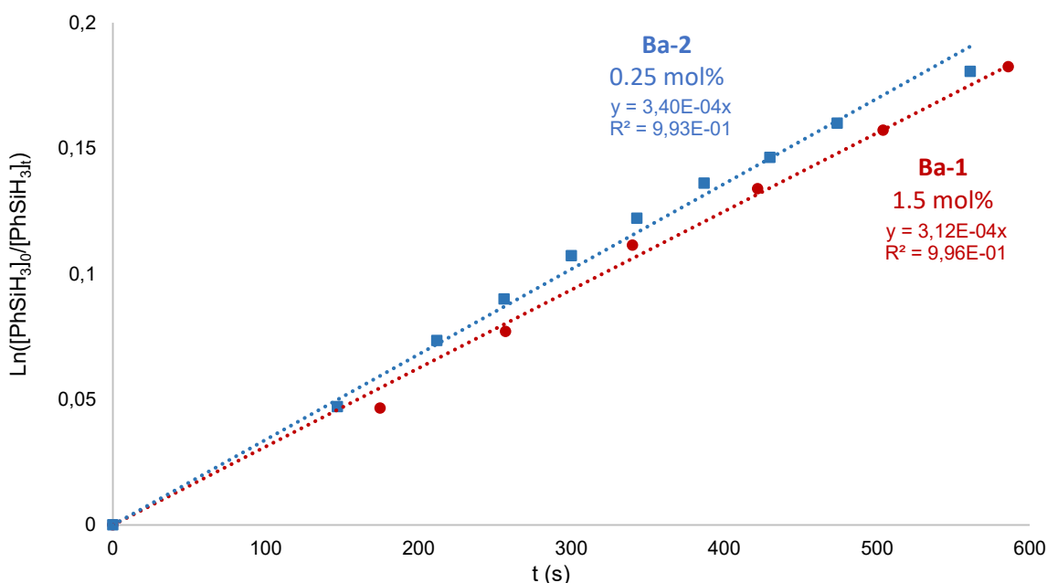
Figure 2.20. Tracé de \ln([PhSiH_3]_0/[PhSiH_3]_t) = k_{app} t en fonction du temps de réaction pour le couplage déshydrogénéant de HOB\{CH(SiMe_3)_2\}_2 ( A ) et PhSiH_3 catalysé par différents complexes : [Ba\{N(SiMe_3)_2\}_2]_2 = 0.42 \cdot 10^{-3} \text{ M} (■), [Ba\{N(SiMe_3)_2\}_2 \cdot 2.thf_2] = 2.54 \cdot 10^{-3} \text{ M} (●). Conditions: \{(Me_3Si)_2CH\}_2BOH (36 mg, 0.102 mmol), PhSiH_3 (13 \mu\text{L} , 0.102 mmol), T = 333 \text{ K} , solvant C_6D_6 (0.6 mL).
