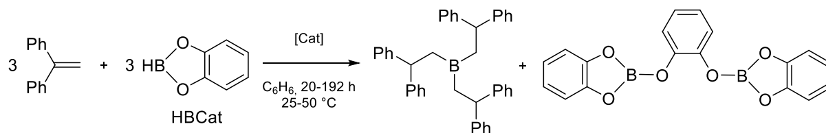
Figure 1.16. Réactions d'hydroboration d'alcènes. [73]
