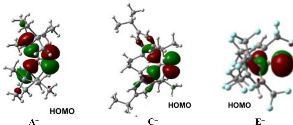
Figure 4.18. Représentation des orbitales frontières \pi (HOMO) pour les fragments borylates A^- , C^- et E^- .
