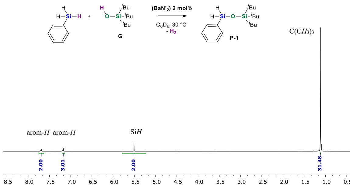
Annexe 7.4. Spectre RMN ^1H ( C_6D_6 , 298 K, 400 MHz) de la réaction de couplage déshydrogénant entre G et PhSiH_3 catalysée par BaN'_2 montrant la formation exclusive du produit de monocouplage.
