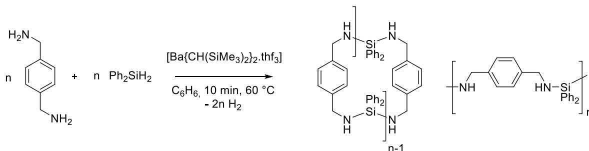
Figure 1.23. Déshydropolymérisation du diphenylsilane avec la p-xylylènediamine par catalysées [\text{Ba}\{\text{CH}(\text{SiMe}_3)_2\}_2 \cdot (\text{thf})_3] .
