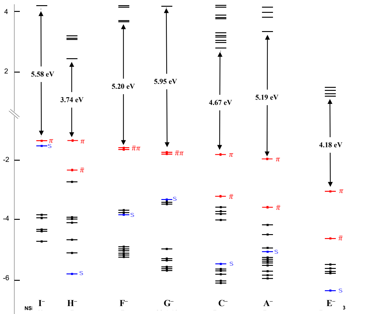
Figure 4.16. Diagramme d'orbitales moléculaires des ligands anioniques étudiés (Energies en eV).
