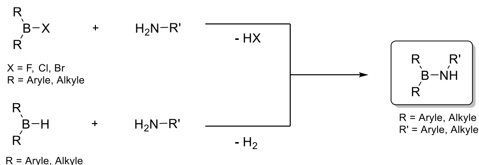
Schéma 6.3. Voies de synthèses proposées pour la formation d'amino-boranes.
