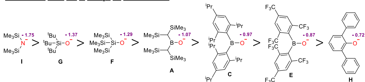
Figure 4.22. Classement des différents ligands étudiés selon la charge de leur hétéroatome.
