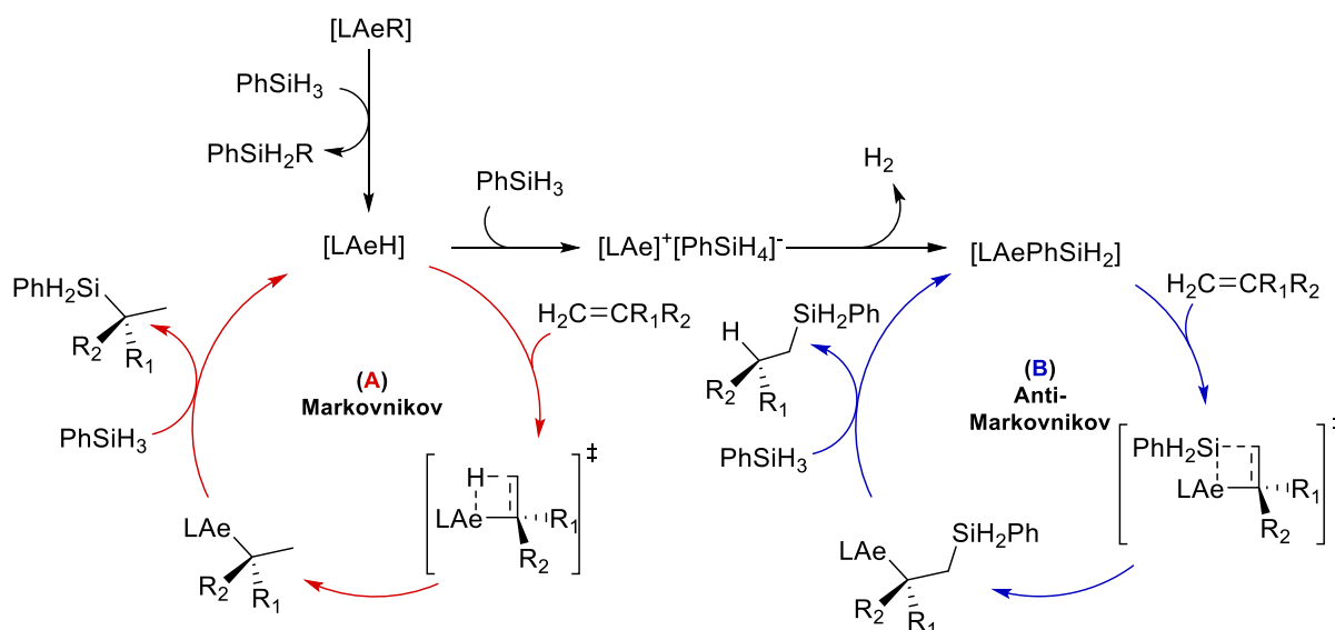
Figure 1.15. Mécanismes réactionnels proposés pour l'hydrosilylation d'alcènes dans des solvants apolaires ( A ) et des solvants polaires ( B ).
