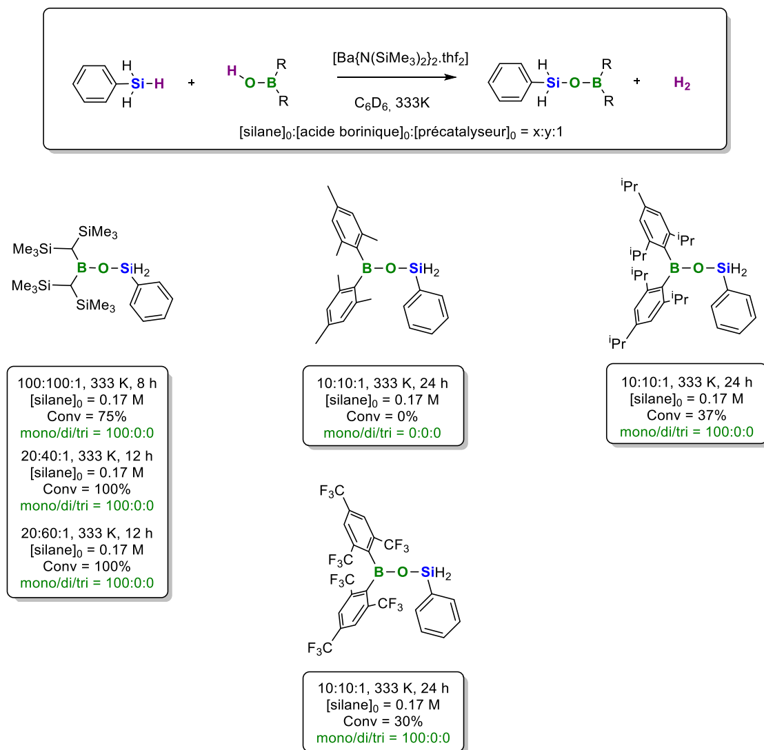
Figure 2.22. Couplage déshydrogénéant de différents acides boriniques avec le phénylsilane. Les réactions ont été réalisées dans C_6D_6 avec le précatalyseur BaN'_2.tfh_2 . Pour chaque réaction, le ratio [silane]_0/[acide\ borinique]_0/[précatalyseur]_0 , la température, la conversion en silane et le chimiosélectivité entre produit mono-, di- et tricouplé sont indiqués.
