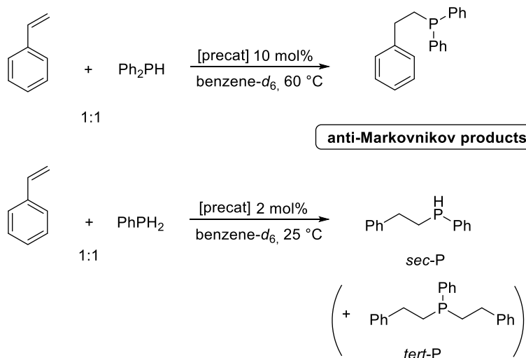
Schéma 5.6. Réaction d'hydrophosphination anti-Markovnikov du styrène par \text{HPPH}_2 ou \text{PhPH}_2 en présence des précatalyseurs [\{\text{I}^{\text{A}^{\text{crown}}}\}\text{BaN}(\text{SiMe}_2\text{H})_2] ( 16 ) et [\{\text{AdAm}^{\text{crown}}\}\text{BaN}(\text{SiMe}_2\text{H})_2] ( 17 ).
