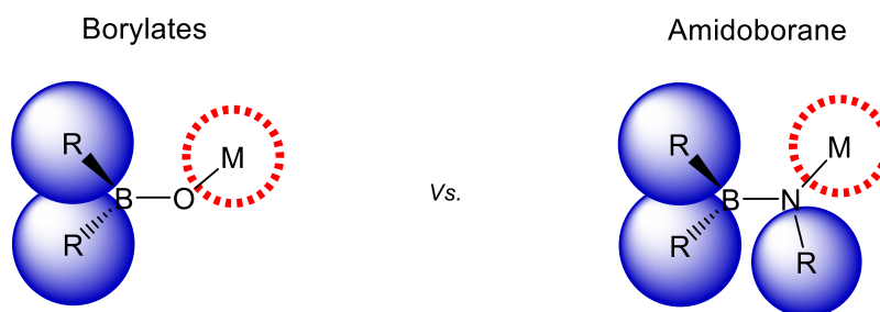
Figure 6.1. Représentation schématique des différences stériques entre borylates et amidoborane.
