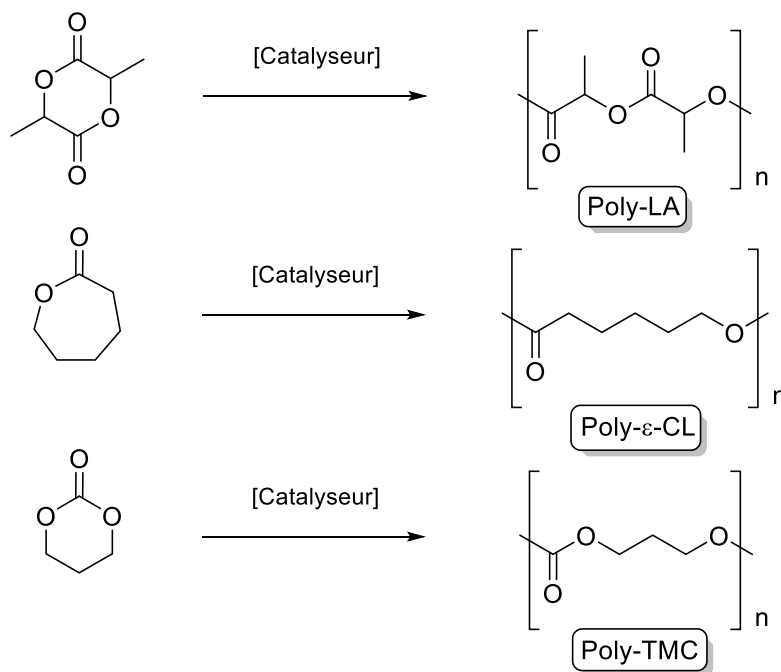
Figure 1.8. La synthèse catalytique de polylactide (Poly-LA), de polycaprolactone (Poly- \epsilon -CL) et de polycarbonate (Poly-TMC).
