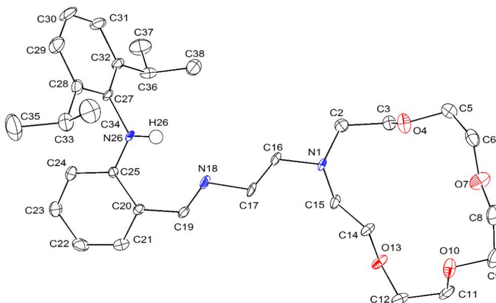
Figure 5.6. Représentation moléculaire ORTEP du proligand \{I^A^{crown}\}H à l'état solide. Niveau de probabilité des ellipsoïdes fixé à 50%. Seulement une des deux molécules de l'unité asymétrique est représentée. Tous les hydrogènes CH ont été supprimés pour plus de clarté.
