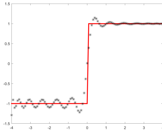
Figure 40 : Développement de X(\mathbf{U}) = \chi_{[0,4]}(\mathbf{U}) - \chi_{[-4,0]}(\mathbf{U}) dans une base trigonométrique à 85 termes pour \mathbf{U} exponentielle sur [-4; 4]
