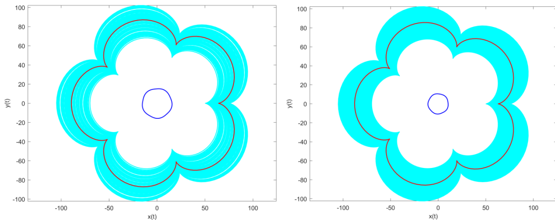
a) 100 épistrochoïdes
