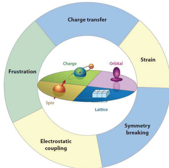
Figure I-14 : Représentation schématique des degrés de liberté des oxydes de métaux de transition et effets pouvant modifier l'interaction entre ces degrés de liberté. [56]
