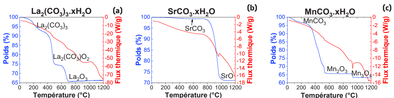
Figure III-2 : Analyses thermogravimétriques (en bleu) et calorimétrie différentielle à balayage (en rouge) des carbonates utilisés comme précurseurs. Le carbonate de lanthane hydraté (a), le carbonate de strontium hydraté (b) et le carbonate de manganèse hydraté (c).
