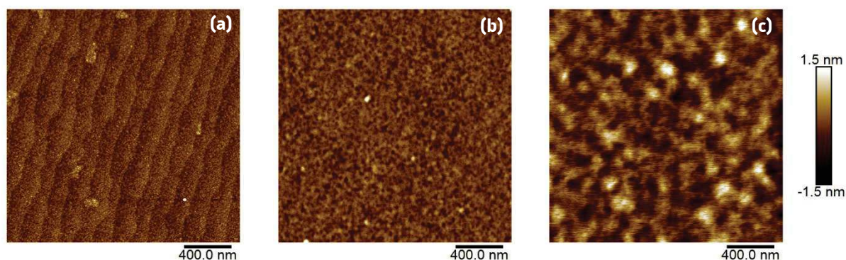
Figure V-5 : Exemples d'images topographiques d'AFM obtenus sur des couches minces de LSMO de 6 nm (a), 9 nm (b) sous une pression de 0,5 mbar en O_2 et de 24 nm sous une pression de 0,3 mbar en O_2 déposés sur LAO(001).
