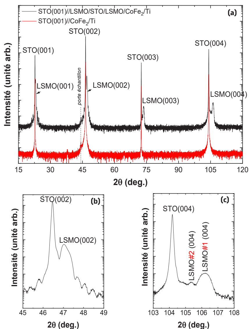
Figure IV-7 : Diffractogrammes en configuration \theta - 2\theta de l'hétérostructure J-1 composée de LSMO#1|STO|LSMO#2|CoFe 2 |Ti déposée sur STO(001) et d'un dépôt de CoFe 2 |Ti sur STO(001) (a). Zoom entre 45 et 49 ° autour du LSMO(002) illustrant la présence de franges de Pendellösung (b). Zoom aux hauts angles entre 103 et 108 ° du \theta - 2\theta de l'hétérostructure J-1 montre distinctement deux pics de diffraction entre 105 et 107 °, un pour chaque couche de LSMO (c).
