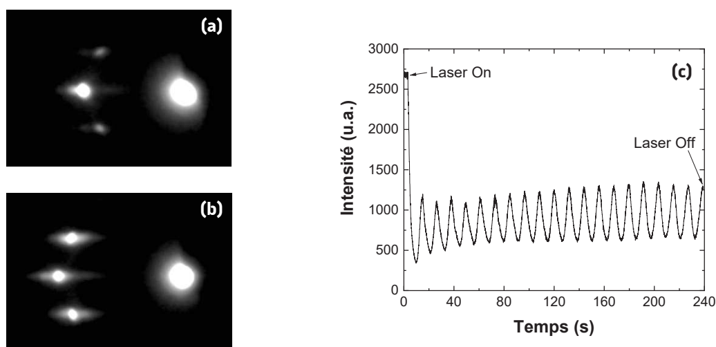
Figure III-13 : Clichés RHEED enregistrés sur un substrat commercial de STO(001) traité par une attaque acide au BHF pendant 30 s (a) et après la croissance homoépitaxiale de 20 couches de STO (b). Oscillations RHEED enregistrées pendant la croissance des films de STO. Une période correspond à 11,8 s (c).
