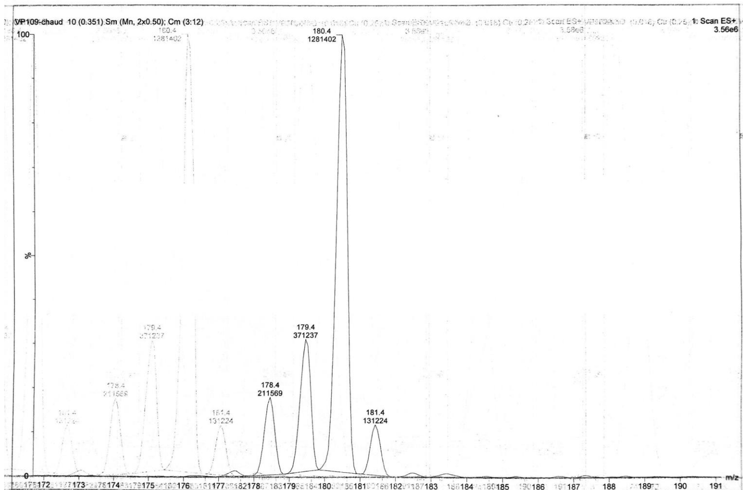
ESI spectrum of 15
