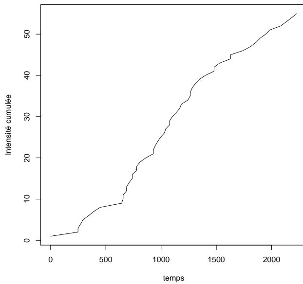
FIGURE 4 : Représentation de l'intensité empirique cumulée pour un orage (Valence, 10 avril 2008)
