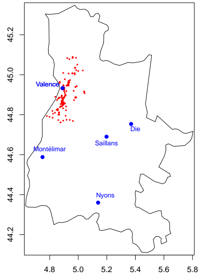
FIGURE 3 : Représentation spatiale d'un orage (Valence, 10 avril 2008)
