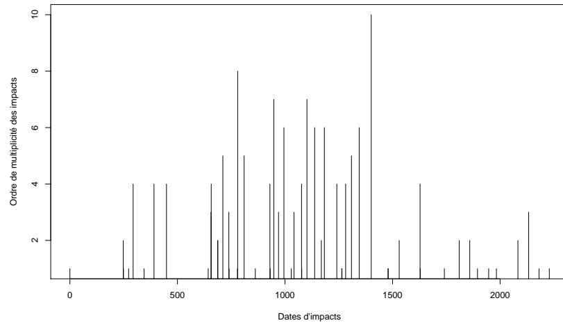
FIGURE 5 : Représentation de la charge des impacts d'un orage (Valence, 10 avril 2008)
