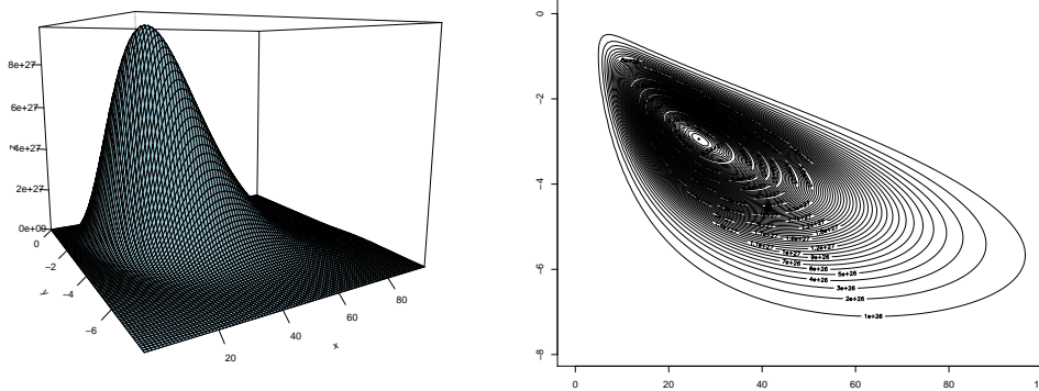
FIGURE 2 : Densité de la loi de probabilité Gamma-Gumbel modifiée de paramètres a = 10 , b = 10 , c = 2 , d = 1 et m = 0
