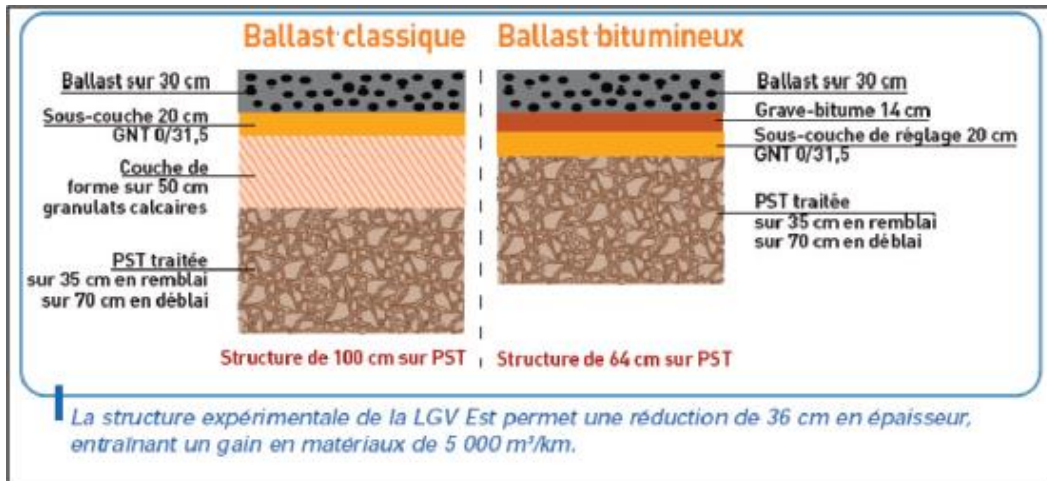
Figure I.26 - Section de la LGV Est avec sous couche classique et sous couche bitumineuse (Bitume Info, 2005)
