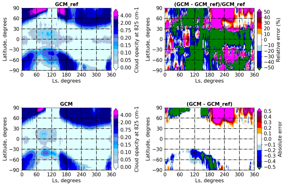
FIGURE 4.16 – Gauche, Haut : Moyenne zonale de l'opacité nuageuse contenue dans le GCM pour une simulation GCM de référence selon Navarro et al. (2014b). Gauche, Bas : Même figure pour une simulation GCM avec la nouvelle méthode d'injection et de contrôle de l'opacité de poussière (avec C_{inj} = 0.25 ), la paramétrisation de l'entraînement de la poussière par vents de pente au-dessus de la topographie sous-maille (avec x_{mons} = 0.5 ), ainsi que la paramétrisation des rocket dust storm (avec une injection entre 10 :00 et 12 :00 et C_{det} = 0.05 ). Droite, Haut : erreur relative entre les deux figes de gauche. Droite, Bas : erreur absolue entre les deux figes de gauche.
