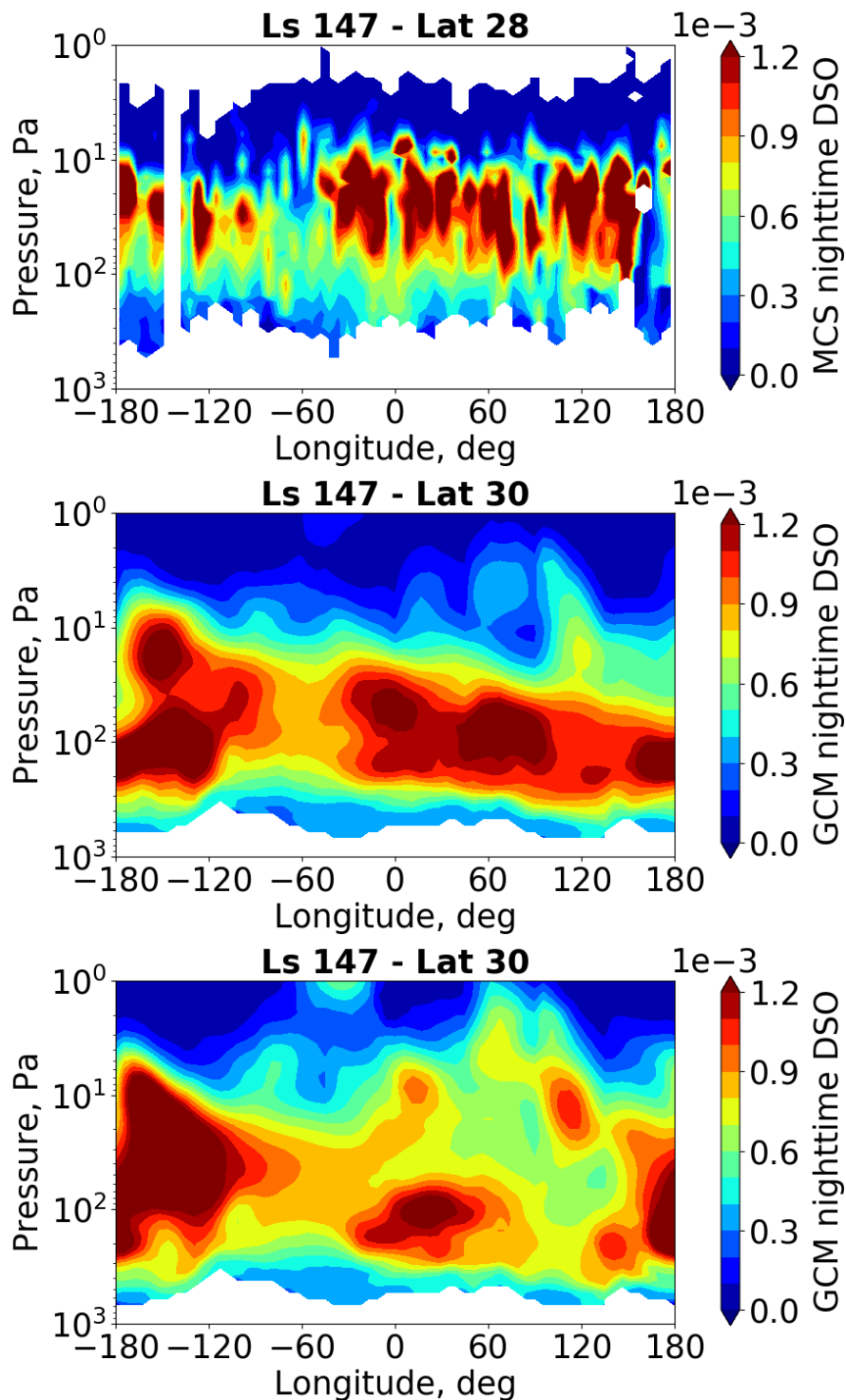
FIGURE 3.33 – Coupe verticale (Pression - Longitude) à L_s \sim 150^\circ de la Density Scaled Opacity (DSO) à la latitude de 30^\circ N . Haut : Données MCS. Milieu : simulation GCM avec la paramétrisation des Rocket Dust Storm telle que \Delta t_{inj} = [10:00; 12:00] et C_{detr} = 0 . Bas : simulation GCM avec la paramétrisation des Rocket Dust Storm telle que \Delta t_{inj} = [8:00; 10:00] et C_{detr} = 0 .
