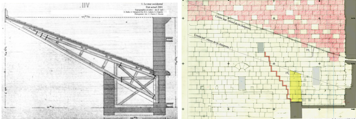
(a) Proposition de restitution de la couverture de la scène par A. Caristie.
