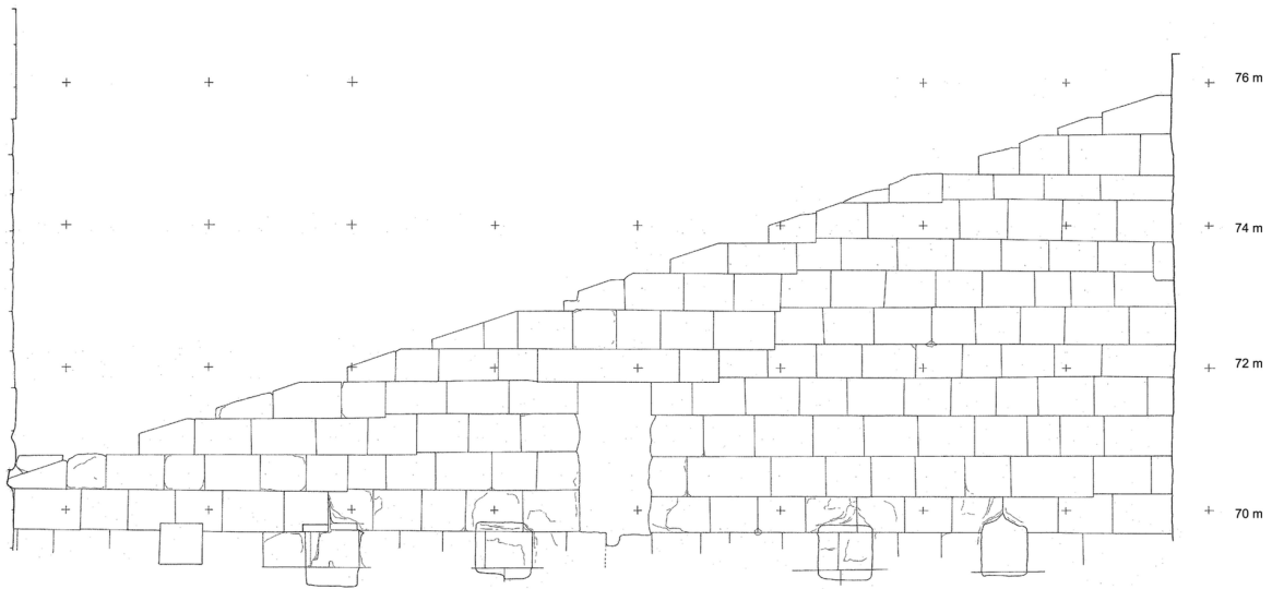
FIGURE A.6 – Elévation de la partie sommitale de la basilique occidentale 6 .
