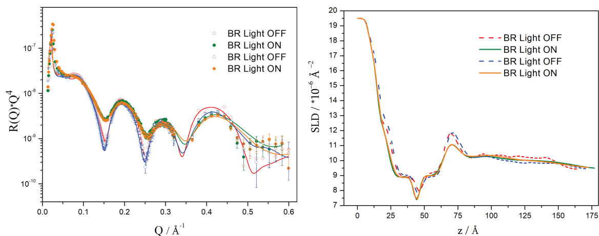
Figure VI.1.2 – (a) Courbes de réflectivité spéculaire de rayons X (synchrotron SOLEIL) pour une double bicouche de DSPC à 25 °C avant et après l’incorporation de la BR, avec et sans illumination. (b) Profils SLD correspondant aux meilleurs ajustements.
