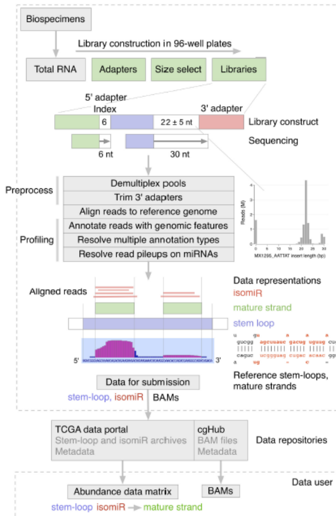
FIGURE 1.9 – Workflows de séquençage, d'alignement de reads et de quantification d'expression suivis par le GDC pour quantifier l'expression de miARN (CHU et al., 2016).
