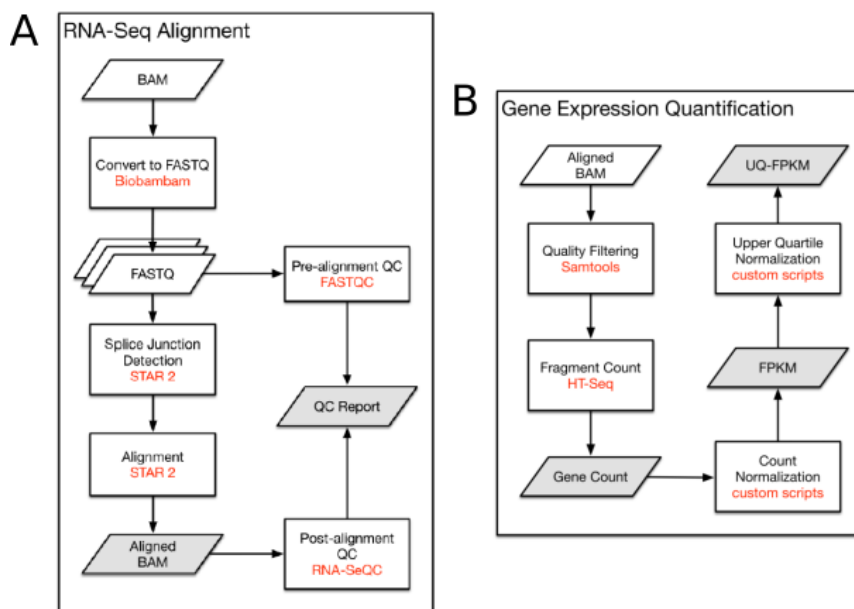
FIGURE 1.7 – Workflows d'alignement de reads (A) et de quantification d'expression (B) suivis par le GDC pour quantifier l'expression de gènes à partir du séquençage d'échantillons ( https://docs.gdc.cancer.gov/Data/Bioinformatics_Pipelines/Expression_mRNA_Pipeline/ ).
