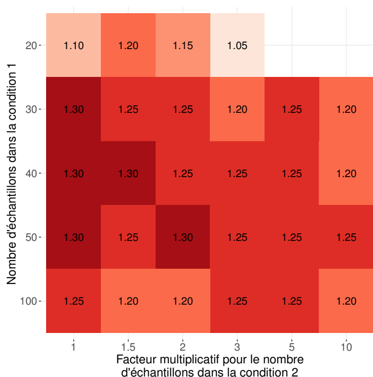
FIGURE 4.15 – Valeurs de seuil de fold-change de moyenne à utiliser pour filtrer les gènes différentiellement exprimés permettant d'obtenir un FDR pour la détection de différence de dispersion inférieur à 0,05 en fonction de l'ensemble des tailles de population d'échantillons considérées. Les cases vides sont dues au fait qu'il n'est pas possible d'obtenir un FDR pour la détection de différence de dispersion inférieur à 0,05 avec les tailles de population d'échantillons correspondantes, quelle que soit la valeur de seuil de fold-change de moyenne (voir figure 4.12).
