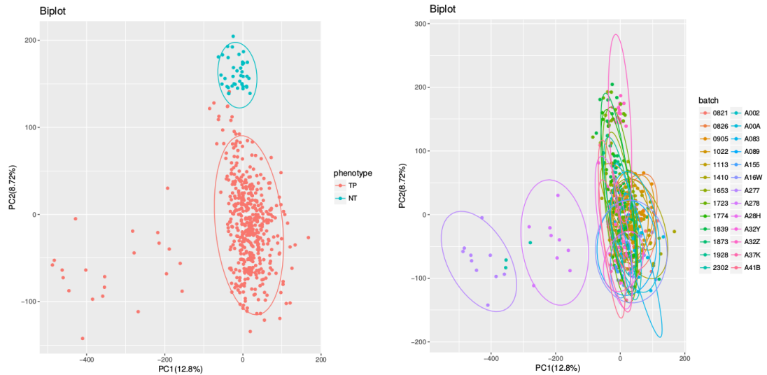
FIGURE 3.8 – ACP des données d'expression du cancer du colon (TCGA-COAD) avant l'application de la méthode de correction d'effets batch ComBat. Graphique de gauche : les échantillons sont colorés en fonction de leur appartenance aux catégories biologiques d'intérêt (échantillons sains en bleu, échantillons tumoraux en rouge). Graphique de droite : les échantillons sont colorés en fonction des expériences de séquençage les ayant générés. Des ellipses ont été ajoutées pour chaque groupe d'échantillons ainsi définis pour pouvoir mieux les distinguer.
