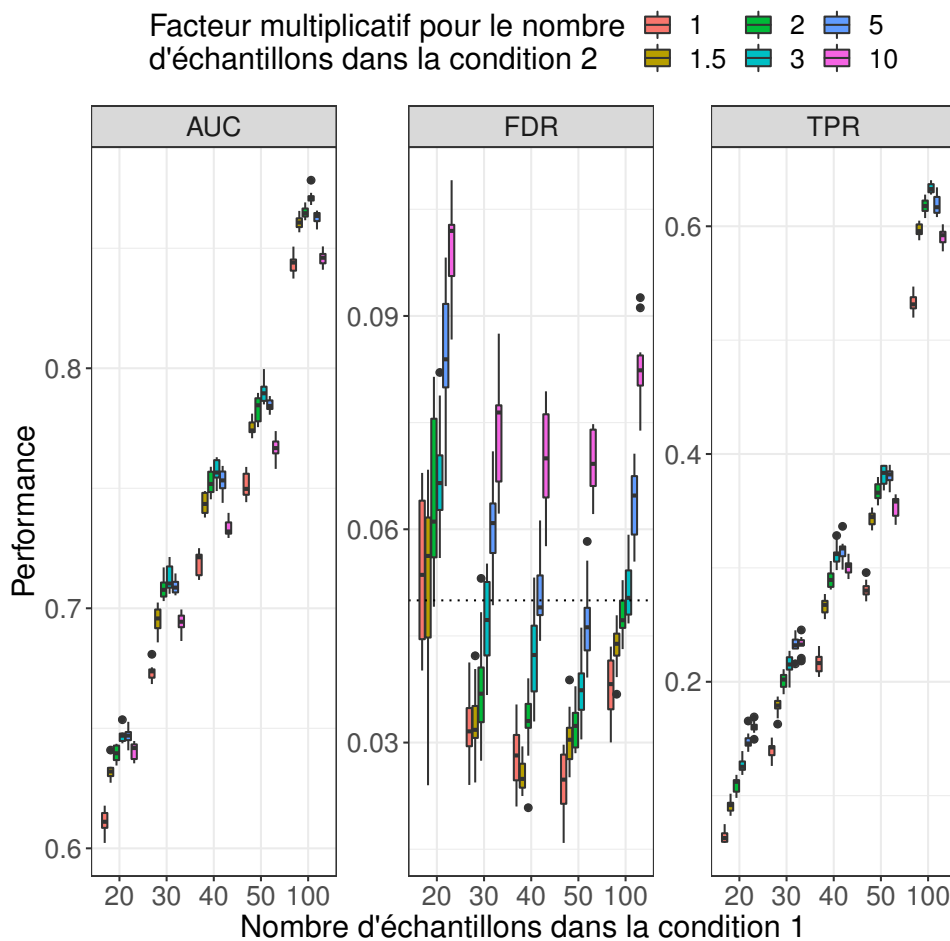
FIGURE A.3 – Performances obtenues avec MDSeq pour la détection de différence de dispersion avec des jeux de données simulées composés de populations d'échantillons de tailles inégales. La taille de la population de la seconde condition peut prendre différentes valeurs, de 1,5 à 10 fois plus grande que la population de la première condition. Paramètres de simulation : 10 000 gènes, 50% de gènes différentiellement dispersés avec une différence de dispersion d'au moins 50%, les gènes non différentiellement dispersés ont la même valeur de dispersion pour les deux populations, les fold-changes de moyenne sont limités par une valeur maximale de 1,4, présence d'un outlier pour 10% des gènes. Les performances ont été mesurées à l'aide de 10 réplicats pour chaque jeu de paramètres. La fonction de retrait d' outliers de MDSeq a été appliquée. Les gènes différentiellement dispersés ont été identifiés à l'aide d'un seuil de fold-change égal à 1.
