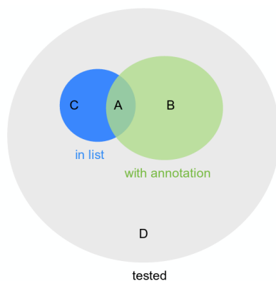
FIGURE 2.7 – Représentation schématique du test d'enrichissement d'un terme Gene Ontology représenté par le cercle vert (« with annotation ») parmi un ensemble de gènes d'intérêt représenté par le cercle bleu (« in list »). Les gènes d'intérêt ont été identifiés parmi un ensemble de gènes testés représenté par le cercle gris (« tested »).
