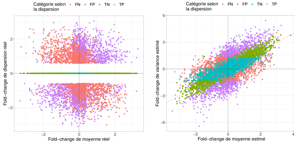
FIGURE 4.4 – Valeurs réelles de fold-changes de moyenne et de dispersion d’un jeu de données simulées composé de 50 échantillons par population (à gauche). Valeurs de fold-changes de moyenne et de variance estimées par MDSeq sur ce même jeu de données simulées. Les couleurs des points correspondent aux résultats de test de différence de variance réalisés par MDSeq avec un fold-change de 1 (à droite). La droite rouge en pointillés représente la diagonale y = x .
