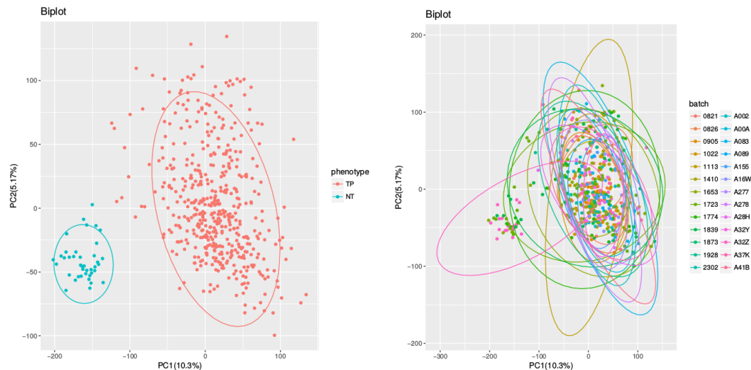
FIGURE 3.9 – ACP des données d’expression du cancer du colon (TCGA-COAD) après l’application de la méthode de correction d’effets batch ComBat. Les mêmes groupes d’échantillons sont définis sur ces deux graphiques que pour la figure 3.8.
