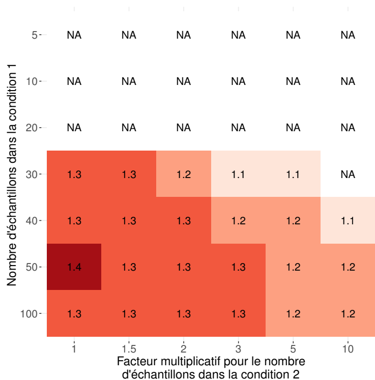
FIGURE 4.16 – Valeurs maximales de fold-change de moyenne permettant d’obtenir un FDR pour la détection de différence de dispersion inférieur à 0,05 dans l’ensemble des réplicats de simulation en fonction de l’ensemble des tailles de population d’échantillons considérées. Les jeux de données sont constitués de 30% de gènes différentiellement dispersés. Une valeur « NA » indique qu’il n’est pas possible d’obtenir un FDR inférieur à 0,05 avec les tailles de population d’échantillons correspondantes, quelle que soit la valeur maximale de fold-change de moyenne.
