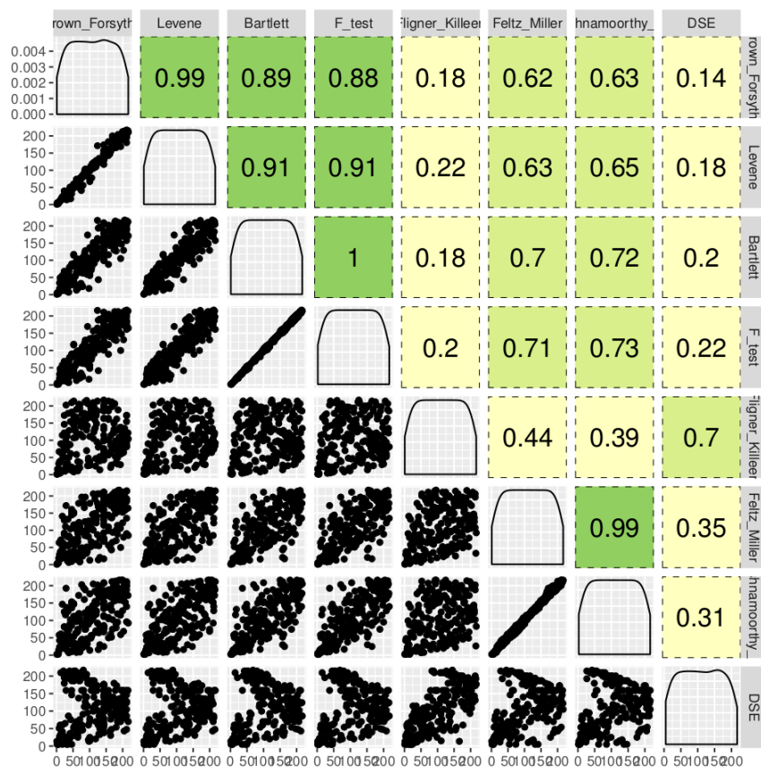
FIGURE 3.1 – Nuage de points des rangs de p-valeur obtenues pour chaque paire de tests statistiques (partie inférieure de la matrice) pour la comparaison des valeurs normalisées d’expression de miARN des échantillons tumoraux et des échantillons sains pour le cancer de la prostate. Corrélation de Pearson des rangs de p-valeur pour chaque paire de tests statistiques (partie supérieure de la matrice).
