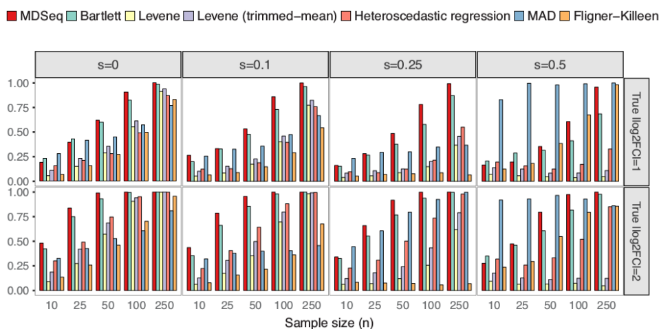
FIGURE 3.12 – Puissances de MDSeq et différents tests de différence de variabilité obtenues à l’aide de données simulées présentant des différences de variance d’expression ( \log_2FC ) entre deux populations d’échantillons de tailles égales (figure 2 de RAN et DAYE, 2017). Différentes tailles de populations ( sample size ) et différentes proportions de valeurs nulles ( s ) dans les valeurs d’expression de chaque gène ont été évaluées.
