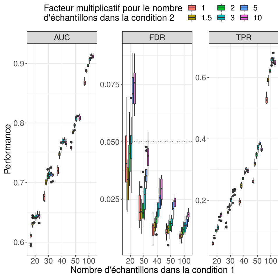
FIGURE A.2 – Performances obtenues avec MDSeq pour la détection de différence de dispersion avec des jeux de données simulées composés de populations d'échantillons de tailles inégales. La taille de la population de la seconde condition peut prendre différentes valeurs, de 1,5 à 10 fois plus grande que la population de la première condition. Paramètres de simulation : 10 000 gènes, 50% de gènes différentiellement dispersés avec une différence de dispersion d'au moins 50%, les gènes non différentiellement dispersés ont la même valeur de dispersion pour les deux populations, les fold-changes de moyenne sont limités par une valeur maximale de 1,2, présence d'un outlier pour 10% des gènes. Les performances ont été mesurées à l'aide de 10 réplicats pour chaque jeu de paramètres. La fonction de retrait d' outliers de MDSeq a été appliquée. Les gènes différentiellement dispersés ont été identifiés à l'aide d'un seuil de fold-change égal à 1.
