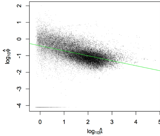
FIGURE 2.4 – Estimateurs \hat{\mu}_i de la moyenne et \hat{\phi}_i de la dispersion par maximum de vraisemblance à partir du jeu de données de PICKRELL et al., 2010 (figure issue de PICKRELL et al., 2010).
