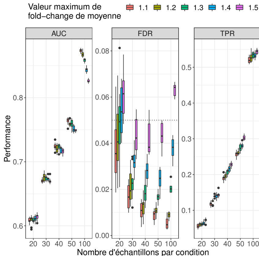
FIGURE 4.9 – Performances obtenues avec MDSeq pour la détection de différence de dispersion avec des jeux de données simulées composés de populations d'échantillons de tailles égales. Paramètres de simulation : 10 000 gènes, 50% de gènes différentiellement dispersés avec une différence de dispersion d'au moins 50%, les gènes non différentiellement dispersés ont la même valeur de dispersion pour les deux populations, les fold-changes de moyenne sont limités par différentes valeurs maximales comprises entre 1,1 et 1,5, présence d'un outlier pour 10% des gènes. Les performances ont été mesurées à l'aide de 10 réplicats pour chaque jeu de paramètres. La fonction de retrait d' outliers de MDSeq a été appliquée. Les gènes différentiellement dispersés ont été identifiés à l'aide d'un seuil de fold-change égal à 1.
