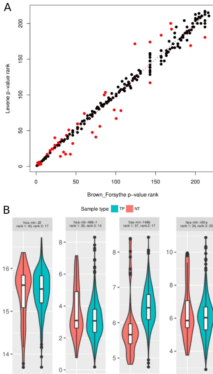
FIGURE 3.6 – A : Comparaison des rangs des p-valeurs obtenues avec les tests de Brown-Forsythe et de Levene à partir des données d’expression normalisées de miARN du cancer de la prostate. Les points rouges représentent les miARN les plus discordants selon la formule 2.3. B : Boxplots des valeurs d’expression parmi les échantillons tumoraux (TP) et sains (NT) de quelques miARN discordants. Rang 1 : rang de p-valeur selon le test de Brown-Forsythe, rang 2 : rang de p-valeur selon le test de Levene.
