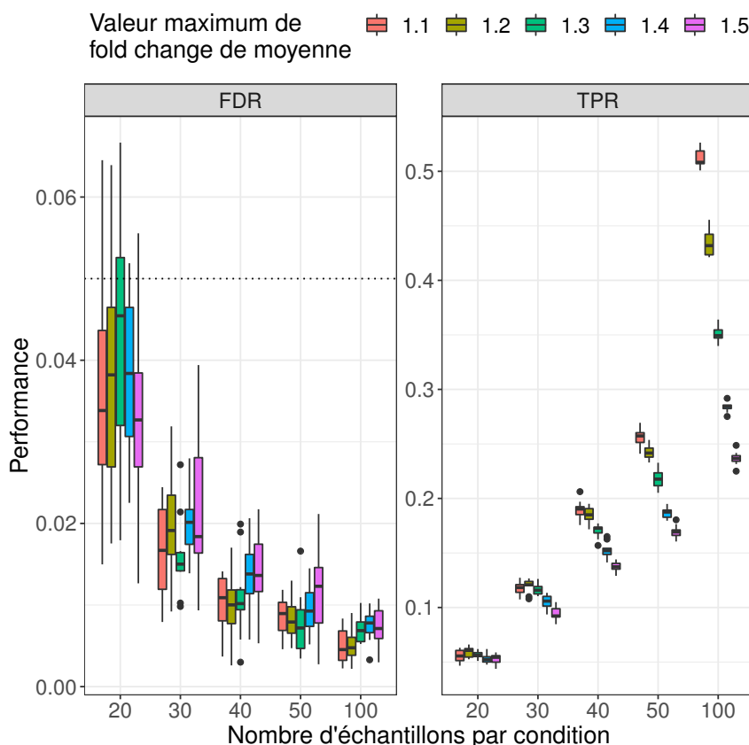
FIGURE 4.13 – Performances obtenues avec MDSeq pour la détection de différence de dispersion avec des jeux de données simulées composés de populations d'échantillons de tailles égales. Paramètres de simulation : 10 000 gènes, 50% de gènes différentiellement dispersés avec une différence de dispersion d'au moins 50%, les gènes non différentiellement dispersés ont la même valeur de dispersion pour les deux populations, les fold-changes de moyenne sont limités par différentes valeurs maximales comprises entre 1,1 et 1,5, présence d'un outlier pour 10% des gènes. Les performances ont été mesurées à l'aide de 10 réplicats pour chaque jeu de paramètres. La fonction de retrait d' outliers de MDSeq a été appliquée. Les gènes différentiellement dispersés ont été identifiés par une p-valeur supérieure à 0,05 pour le test de différence de moyenne et une p-valeur inférieure à 0,05 pour le test de différence de variance avec des valeurs de seuil de fold-change égales à 1.
