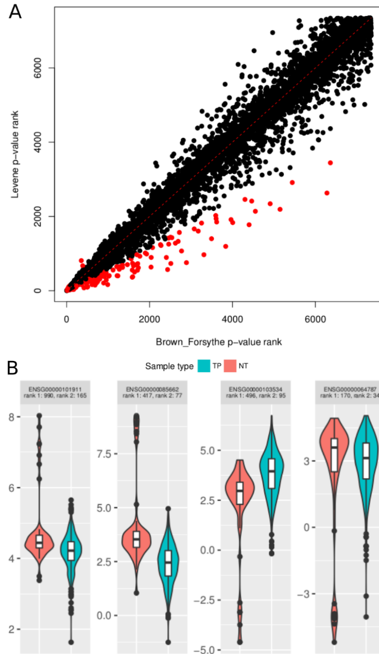
FIGURE 3.7 – A : Comparaison des rangs des p-valeurs obtenues avec les tests de Brown-Forsythe et de Levene à partir des données d’expression normalisées d’ARNm du cancer de la prostate. Les points rouges représentent les ARNm les plus discordants selon la formule 2.3. B : Boxplots des valeurs d’expression parmi les échantillons tumoraux (TP) et sains (NT) des quatre ARNm les plus discordants. Rang 1 : rang de p-valeur selon le test de Brown-Forsythe, rang 2 : rang de p-valeur selon le test de Levene (B).
