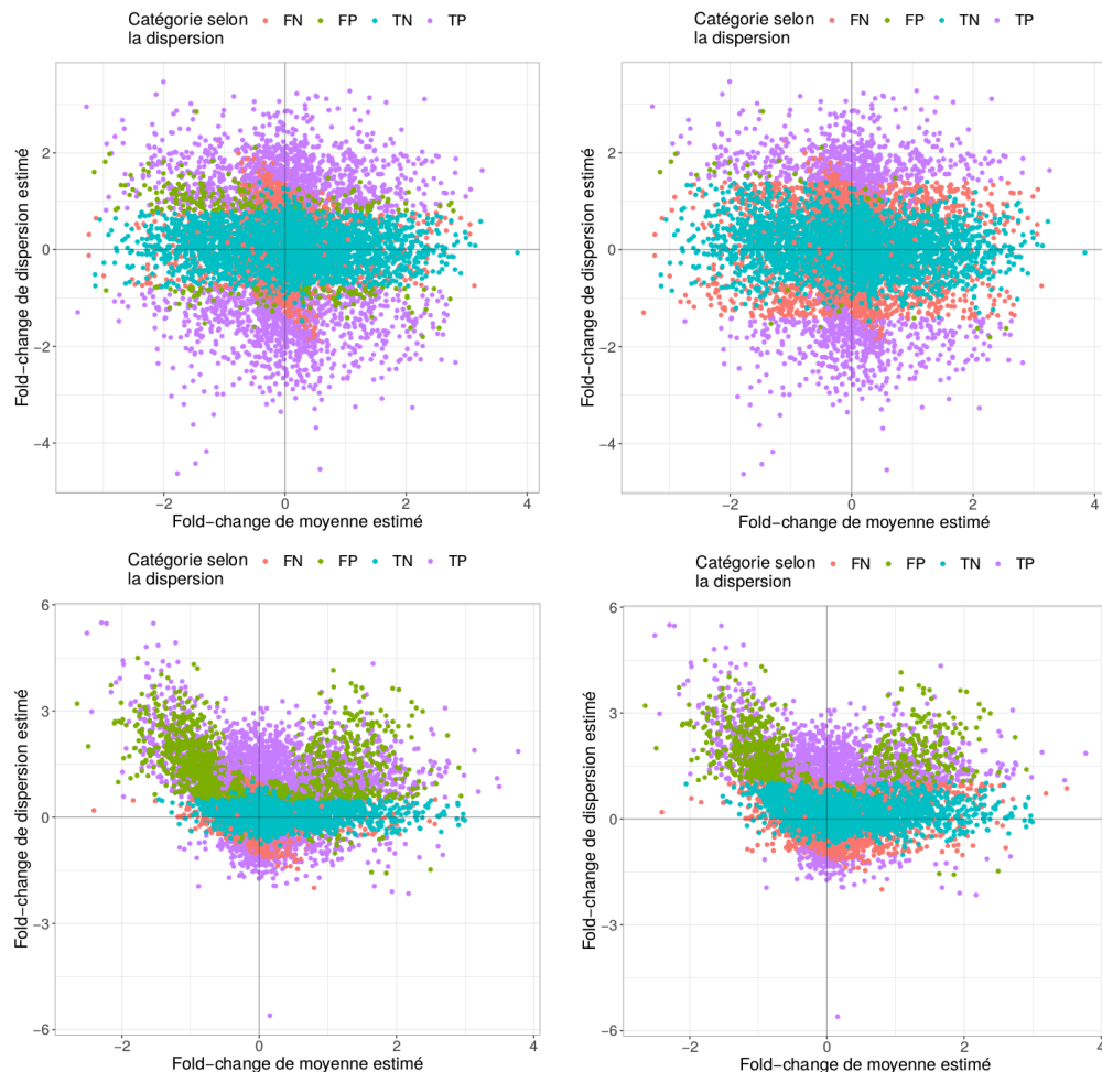
FIGURE 4.17 – Valeurs de fold-changes de moyenne et de dispersion estimées par MDSeq pour un jeu de données simulées composé de 50 échantillons par population, le même que pour la figure 4.5 (en haut). Les couleurs des points correspondent aux résultats de tests de différence de moyenne et de variance réalisés par MDSeq avec un seuil de fold-change de 1 pour les gènes non différentiellement exprimés. Pour les gènes différentiellement exprimés, les gènes différentiellement dispersés sont identifiés à l’aide d’un seuil de fold-change de dispersion fixé à la valeur minimale de fold-change de dispersion parmi les gènes différentiellement variants et non différentiellement exprimés (en haut à gauche) ou de la moyenne des 50 plus faibles valeurs de fold-change de dispersion parmi les gènes différentiellement variants et non différentiellement exprimés (en haut à droite). Graphiques équivalents avec des populations de 50 et 500 échantillons au bas de la figure, utilisation du même jeu de données simulées que pour la figure 4.11 (en bas).
