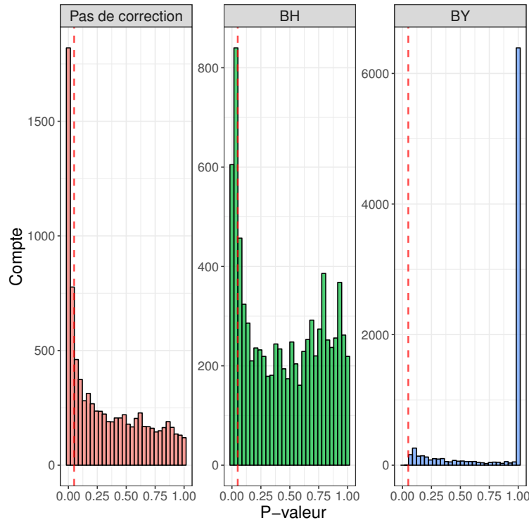
FIGURE 4.2 – Histogrammes des p-valeurs non corrigées et corrigées selon les méthodes de Benjamini-Hochberg (BH) et de Benjamini-Yekutieli (BY) obtenues avec DiPhiSeq pour la détection de différence de dispersion sur le même jeu de données simulées que pour la figure 4.1. Les nombres de reads ont été normalisés selon la méthode TMM et les gènes dont la moyenne d’expression est inférieure à 1 CPM ont été filtrés. La ligne rouge en pointillés représente le seuil de p-valeur à 0,05.
