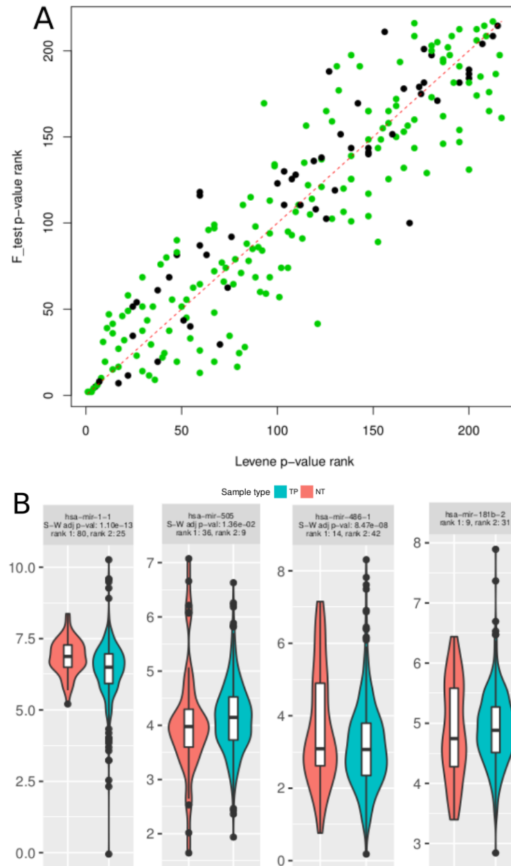
FIGURE 3.3 – A : Nuage de points des rangs de p-valeur obtenues avec le test de Levene et le test de Fisher à partir des données d’expression normalisées des miARN des échantillons tumoraux et sains du cancer de la prostate. Les points verts représentent des miARN dont la p-valeur du test de Shapiro-Wilk est inférieure à 0,05 pour au moins l’un des deux groupes d’échantillons. B : Boxplots des valeurs d’expression de quatre miARN dont l’expression ne suit pas la loi normale pour au moins l’un des deux groupes d’échantillons et dont les rangs de p-valeur sont discordants selon le test de Levene et le test de Fisher. Rang 1 : rang de p-valeurs selon le test de Levene, rang 2 : rang de p-valeurs selon le test de Fisher.
