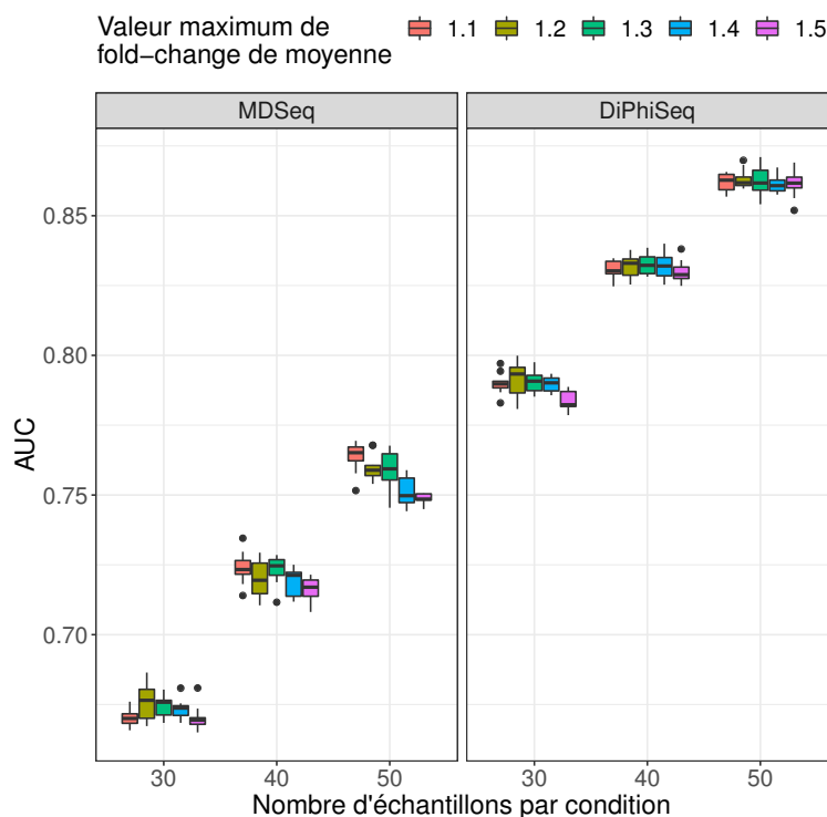
FIGURE 4.6 – AUC obtenues avec MDSeq et DiPhiSeq pour la détection de différence de dispersion avec des jeux de données simulées composés de populations d'échantillons de tailles égales. Paramètres de simulation : 10 000 gènes, 50% de gènes différentiellement dispersés avec une différence de dispersion d'au moins 50%, les gènes non différentiellement dispersés ont la même valeur de dispersion pour les deux populations, les fold-changes de moyenne sont limités par différentes valeurs maximales comprises entre 1,1 et 1,5, présence d'un outlier pour 10% des gènes. Les performances ont été mesurées à l'aide de 10 réplicats pour chaque jeu de paramètres. La fonction de retrait d' outliers de MDSeq a été appliquée. Les gènes différentiellement dispersés ont été identifiés à l'aide d'un seuil de fold-change égal à 1 pour les deux méthodes.
