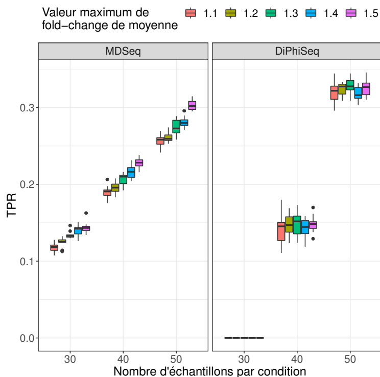
FIGURE 4.8 – Sensibilités, ou TPR, obtenues avec MDSeq et DiPhiSeq pour la détection de différence de dispersion avec des jeux de données simulées composés de populations d'échantillons de tailles égales. Les mêmes jeux de données simulés que pour la figure 4.6 ont été utilisés.
