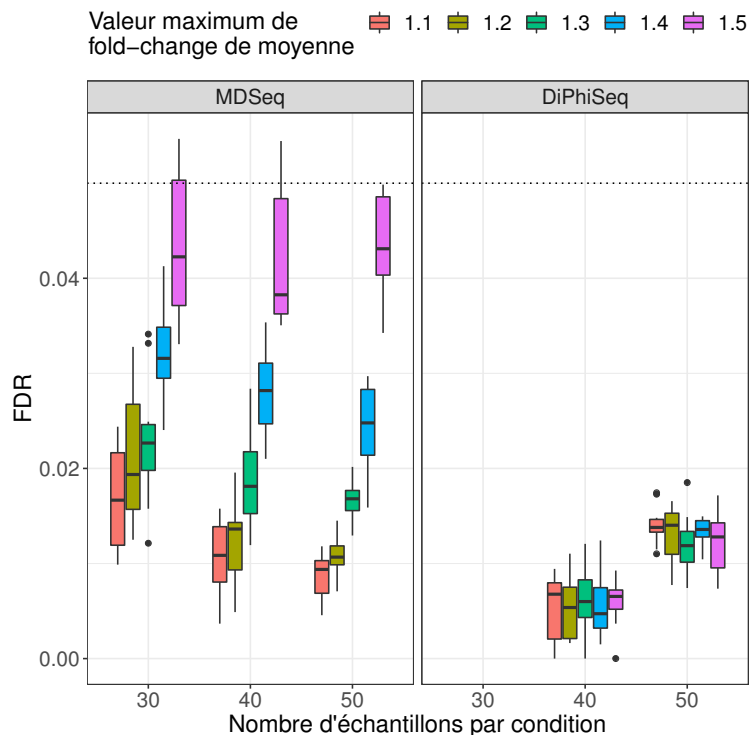
FIGURE 4.7 – FDR obtenus avec MDSeq et DiPhiSeq pour la détection de différence de dispersion avec des jeux de données simulées composés de populations d'échantillons de tailles égales. Les mêmes jeux de données simulées que pour la figure 4.6 ont été utilisés.
