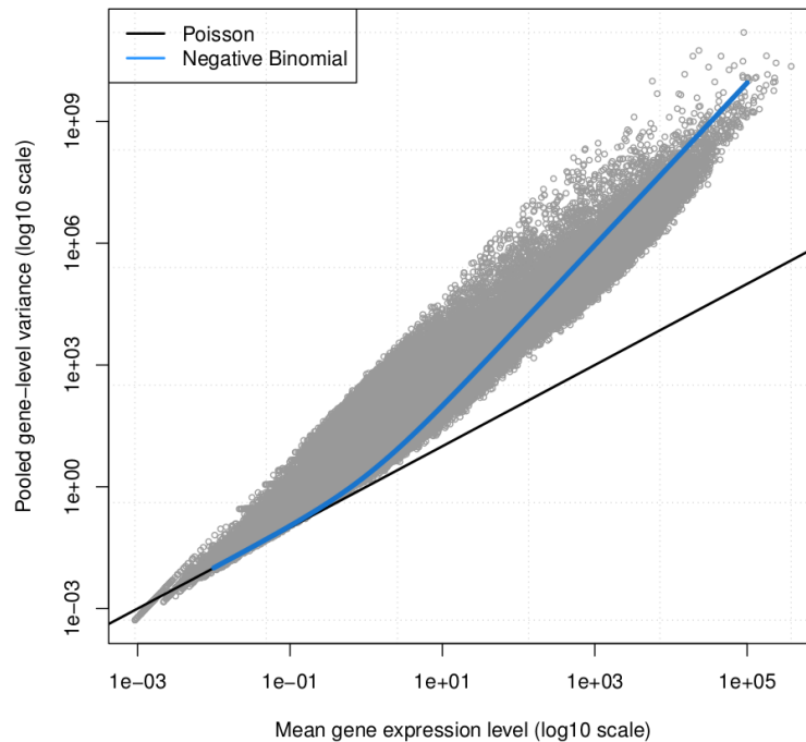
FIGURE 2.2 – Moyennes et variances de nombres de reads et ajustements d'une distribution de Poisson et d'une distribution binomiale négative.
