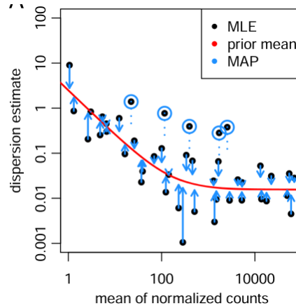
FIGURE 2.3 – Illustration de l’approche d’estimation de la dispersion développée dans le package DESeq2 (LOVE, HUBER et ANDERS, 2014). Les points représentent les estimateurs du maximum de vraisemblance de la dispersion obtenus à l’aide des nombres de reads de chaque gène respectivement. La courbe rouge est la courbe d’ajustement des estimateurs pour capturer la tendance entre la moyenne et la dispersion. Elle est utilisée comme a priori d’une seconde estimation de la dispersion consistant à ajuster les estimateurs de la dispersion propres à chaque gène à la tendance globale. Cet ajustement est représenté par les flèches bleues. Certains estimateurs sont considérés comme des valeurs aberrantes et ne sont pas modifiés par la tendance globale (cercles bleus).
