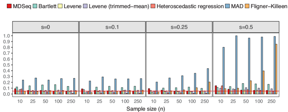
FIGURE 3.11 – Proportions d’erreurs de type I de MDSeq et différents tests de différence de variabilité obtenues à l’aide de données simulées ne présentant pas de différence de variance d’expression entre deux populations d’échantillons de tailles égales (figure 1 de RAN et DAYE, 2017). Différentes tailles de populations ( sample size ) et différentes proportions de valeurs nulles ( s ) dans les valeurs d’expression de chaque gène ont été évaluées.
