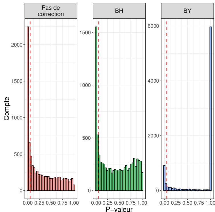
FIGURE 4.1 – Histogrammes des p-valeurs non corrigées et corrigées selon les méthodes de Benjamini-Hochberg (BH) et de Benjamini-Yekutieli (BY) obtenues avec MDSeq pour la détection de différence de dispersion sur un jeu de données simulées composé de deux populations de 50 échantillons. Paramètres de simulations : 10 000 gènes, 50% de gènes différentiellement dispersés avec une différence de dispersion d’au moins 50%, fold-changes de moyenne contenues entre 1 et 1,3, introduction d’un outlier pour 10% des gènes. Les nombres de reads ont été normalisés selon la méthode TMM et les gènes dont la moyenne d’expression est inférieure à 1 CPM ont été filtrés, la fonction de retrait d’ outliers de MDSeq a été appliquée. Les gènes différentiellement dispersés ont été identifiés à l’aide d’un seuil de fold-change égal à 1. La ligne rouge en pointillés représente le seuil de p-valeur à 0,05.
