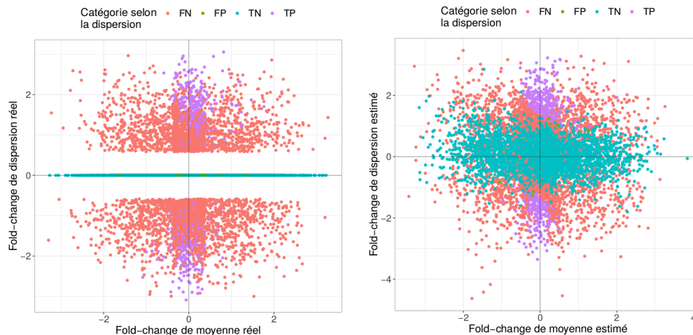
FIGURE 4.5 – Valeurs réelles de fold-changes de moyenne et de dispersion d'un jeu de données simulées composé de 50 échantillons par population (le même jeu de données que pour la figure 4.4, à gauche). Valeurs de fold-changes de moyenne et de dispersion estimées par MDSeq sur ce même jeu de données simulées. Les couleurs des points correspondent aux résultats de test de différence de variance réalisés par MDSeq avec un fold-change de 1 (à droite).
