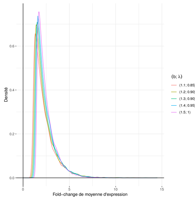
FIGURE 2.5 – Courbes de densité de 10 000 valeurs de fold-changes obtenues avec différentes paires de paramètres b et \lambda .
