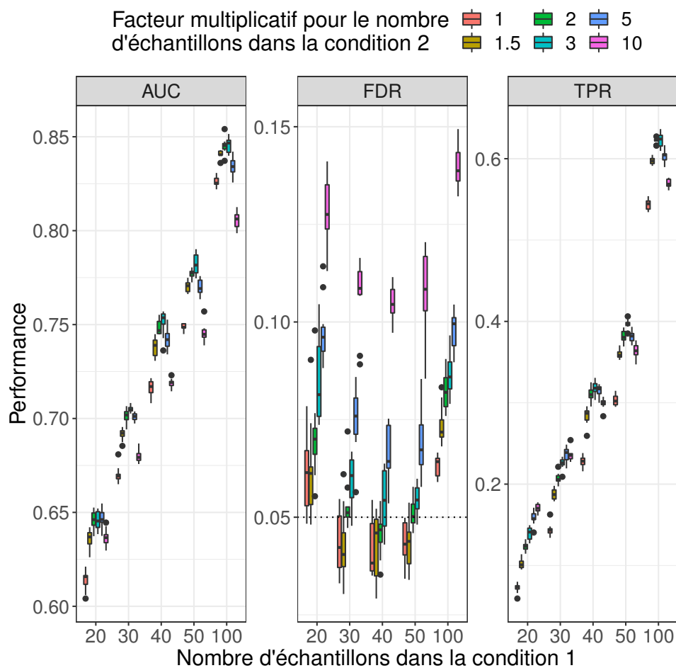
FIGURE A.4 – Performances obtenues avec MDSeq pour la détection de différence de dispersion avec des jeux de données simulées composés de populations d'échantillons de tailles inégales. La taille de la population de la seconde condition peut prendre différentes valeurs, de 1,5 à 10 fois plus grande que la population de la première condition. Paramètres de simulation : 10 000 gènes, 50% de gènes différentiellement dispersés avec une différence de dispersion d'au moins 50%, les gènes non différentiellement dispersés ont la même valeur de dispersion pour les deux populations, les fold-changes de moyenne sont limités par une valeur maximale de 1,5, présence d'un outlier pour 10% des gènes. Les performances ont été mesurées à l'aide de 10 réplicats pour chaque jeu de paramètres. La fonction de retrait d' outliers de MDSeq a été appliquée. Les gènes différentiellement dispersés ont été identifiés à l'aide d'un seuil de fold-change égal à 1.
