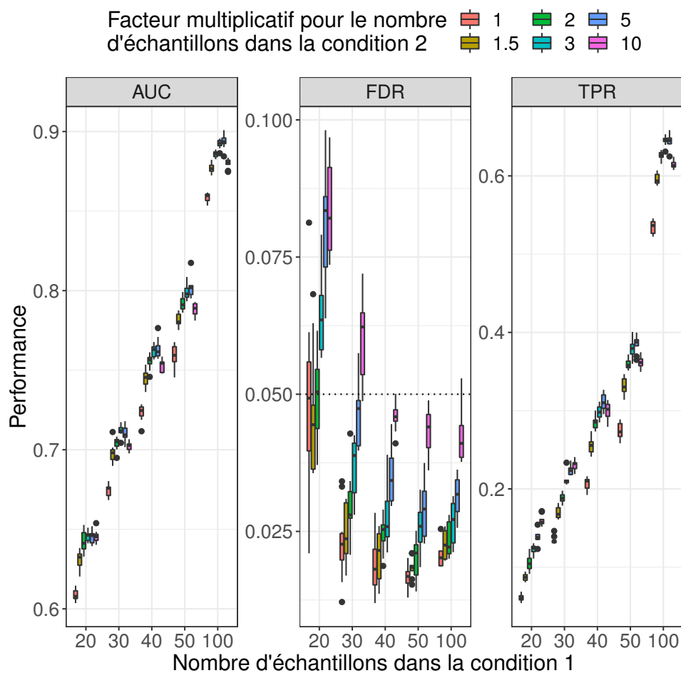
FIGURE 4.10 – Performances obtenues avec MDSeq pour la détection de différence de dispersion avec des jeux de données simulés composés de populations d'échantillons de tailles inégales. La taille de la population de la seconde condition peut prendre différentes valeurs, de 1,5 à 10 fois plus grande que la population de la première condition. Paramètres de simulation : 10 000 gènes, 50% de gènes différentiellement dispersés avec une différence de dispersion d'au moins 50%, les gènes non différentiellement dispersés ont la même valeur de dispersion pour les deux populations, les fold-changes de moyenne sont limités par une valeur maximale de 1,3, présence d'un outlier pour 10% des gènes. Les performances ont été mesurées à l'aide de 10 réplicats pour chaque jeu de paramètres. La fonction de retrait d' outliers de MDSeq a été appliquée. Les gènes différentiellement dispersés ont été identifiés à l'aide d'un seuil de fold-change égal à 1.
