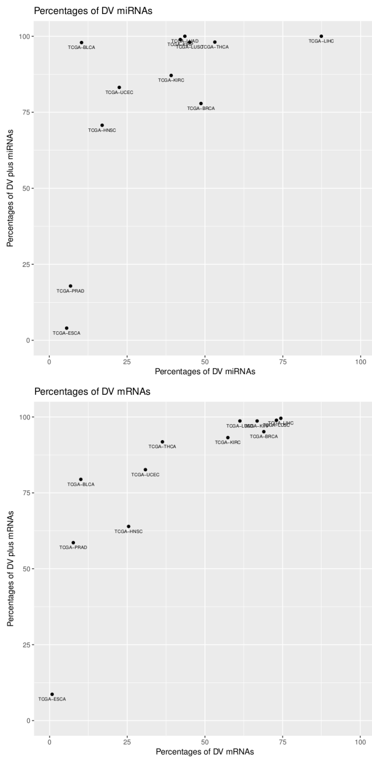
FIGURE 3.10 – Pourcentages de gènes, miARN (en haut) et ARNm (en bas), identifiés comme étant différentiellement variants (DV) après l'application du test de Levene dans le cadre de la comparaison des échantillons tumoraux et sains du TCGA. L'axe des ordonnées sur ces graphiques représente le pourcentage de gènes présentant une augmentation de leur variance d'expression (« DV plus ») dans les tumeurs parmi l'ensemble des gènes différentiellement variants.
