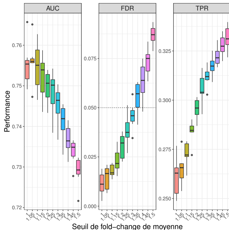
FIGURE 4.14 – Performances obtenues avec MDSeq pour la détection de différence de dispersion avec des jeux de données simulées composés de deux populations de 50 échantillons. Paramètres de simulation : 10 000 gènes, 50% de gènes différentiellement dispersés avec une différence de dispersion d’au moins 50%, les gènes non différentiellement dispersés ont la même valeur de dispersion pour les deux populations, une valeur de fold-change de moyenne de 1,5 définit la séparation entre gènes différentiellement exprimés et non différentiellement exprimés, présence d’un outlier pour 10% des gènes. Les performances ont été mesurées à l’aide de 10 réplicats pour chaque jeu de paramètres. La fonction de retrait d’ outliers de MDSeq a été appliquée. Les gènes différentiellement exprimés ont été filtrés selon différentes valeurs de seuil de fold-change de moyenne. Les gènes différentiellement dispersés ont été identifiés à l’aide d’un seuil de fold-change égal à 1.
