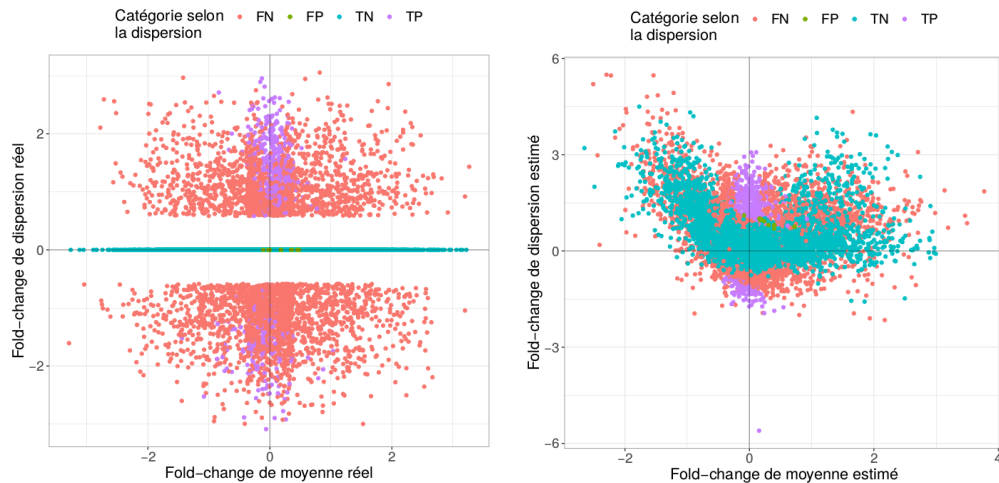
FIGURE 4.11 – Valeurs réelles de fold-changes de moyenne et de dispersion d’un jeu de données simulées composé de populations de 50 échantillons pour la première condition et de 500 échantillons pour la seconde condition (les mêmes valeurs que pour le jeu de données de la figure 4.5, à gauche). Valeurs de fold-changes de moyenne et de dispersion estimées par MDSeq sur ce même jeu de données simulées (à droite). Les couleurs des points correspondent aux résultats de test de différence de variance réalisés par MDSeq avec un fold-change de 1.
