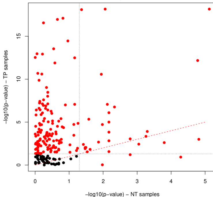
FIGURE 3.2 – P-valeurs obtenues avec le test de Shapiro-Wilk après ajustement par la procédure de Benjamini-Hochberg pour les données d’expression de miARN des échantillons tumoraux et sains du cancer de la prostate. Les valeurs normalisées d’expression ont été transformées en \log_2 . Seuls les 217 miARN dont l’expression moyenne est supérieure ou égale à 2 parmi les deux groupes d’échantillons ont été conservés. Les valeurs -\log_{10} des p-valeurs sont représentées. Les seuils à 0,05 pour les deux groupes et la droite d’identité ont été tracés en pointillés. Les points rouges représentent des miARN dont la p-valeur est inférieure à 0,05 pour au moins l’un des deux groupes d’échantillons. TP : Tumor Primary , NT : Non Tumoral .
