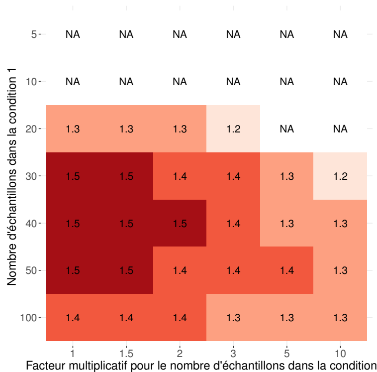
FIGURE 4.12 – Valeurs maximales de fold-change de moyenne permettant d’obtenir un FDR pour la détection de différence de dispersion inférieur à 0,05 dans l’ensemble des réplicats de simulation en fonction de l’ensemble des tailles de population d’échantillons considérées. Une valeur « NA » indique qu’il n’est pas possible d’obtenir un FDR inférieur à 0,05 avec les tailles de population d’échantillons correspondantes, quelle que soit la valeur maximale de fold-change de moyenne.
