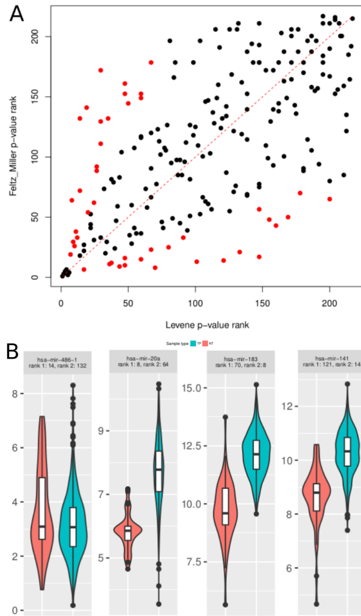
FIGURE 3.5 – A : Comparaison des rangs des p-valeurs obtenues avec les tests de Levene et de Feltz-Miller à partir des données d'expression normalisées de miARN du cancer de la prostate. Les points rouges représentent les miARN les plus discordants selon la formule 2.3. B : Boxplots des valeurs d'expression parmi les échantillons tumoraux (TP) et sains (NT) de quelques miARN discordants. Rang 1 : rang de p-valeur selon le test de Levene, rang 2 : rang de p-valeur selon le test de Feltz-Miller.
