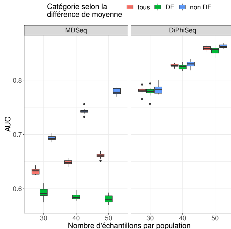
FIGURE 4.3 – AUC obtenues avec MDSeq et DiPhiSeq pour la détection de différence de dispersion avec des jeux de données simulées composés de populations d'échantillons de tailles égales. Paramètres de simulation : 10 000 gènes, 50% de gènes différentiellement dispersés avec une différence de dispersion d'au moins 50%, les gènes non différentiellement dispersés ont la même valeur de dispersion pour les deux populations, une valeur de fold-change de moyenne de 1,3 définit la séparation entre gènes différentiellement exprimés (DE) et non différentiellement exprimés (non DE), présence d'un outlier pour 10% des gènes. Les performances ont été mesurées à l'aide de 10 réplicats pour chaque jeu de paramètres. La fonction de retrait d' outliers de MDSeq a été appliquée. Les gènes différentiellement dispersés ont été identifiés à l'aide d'un seuil de fold-change égal à 1 pour les deux méthodes.
