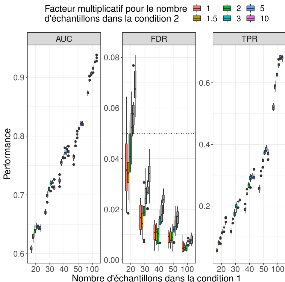
FIGURE A.1 – Performances obtenues avec MDSeq pour la détection de différence de dispersion avec des jeux de données simulées composés de populations d'échantillons de tailles inégales. La taille de la population de la seconde condition peut prendre différentes valeurs, de 1,5 à 10 fois plus grande que la population de la première condition. Paramètres de simulation : 10 000 gènes, 50% de gènes différentiellement dispersés avec une différence de dispersion d'au moins 50%, les gènes non différentiellement dispersés ont la même valeur de dispersion pour les deux populations, les fold-changes de moyenne sont limités par une valeur maximale de 1,1, présence d'un outlier pour 10% des gènes. Les performances ont été mesurées à l'aide de 10 réplicats pour chaque jeu de paramètres. La fonction d' outliers de MDSeq a été appliquée. Les gènes différentiellement dispersés ont été identifiés à l'aide d'un seuil de fold-change égal à 1.
